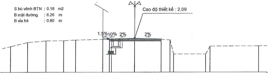
Cọc 17 Km 0 + 460.00 Cao độ :1.96
