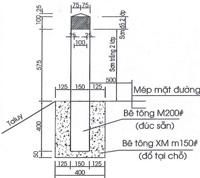
CẦU TẠO CỌC TIÊU
