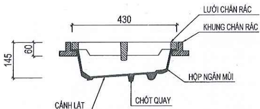
MẶT CẮT 1-1 (TRẠNG THÁI ĐÓNG NGĂN MÙI)
