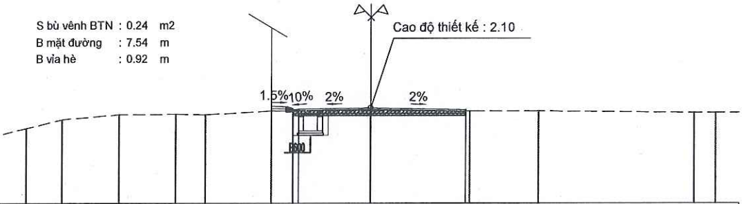
Cọc D8 Km 0 + 467.75 Cao độ :1.96
