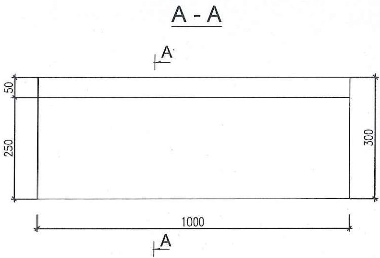
CHI TIẾT BÓ VĨA VÁT HOA VẪN KT(12.5X30X100)CM
