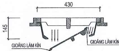
MẶT CẮT 1-1 (TRẠNG THÁI MỞ XẢ NƯỚC)
