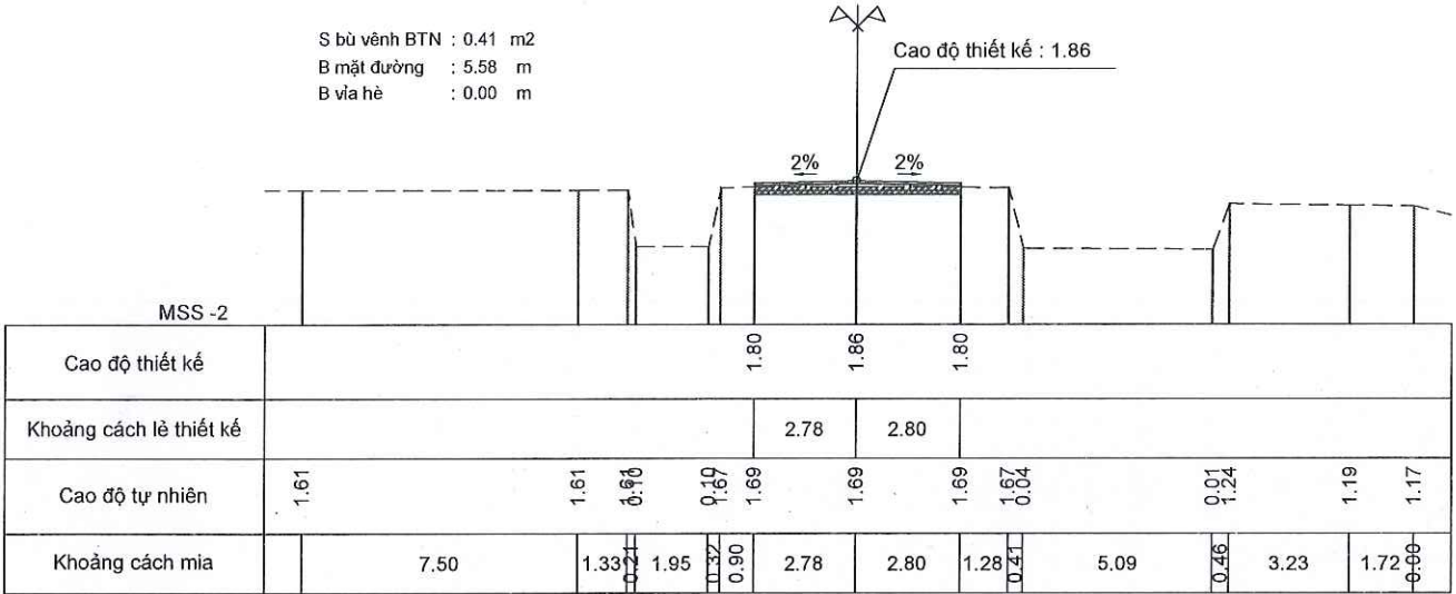
Cọc 7 Km 0 + 220.00 Cao độ :1.69
