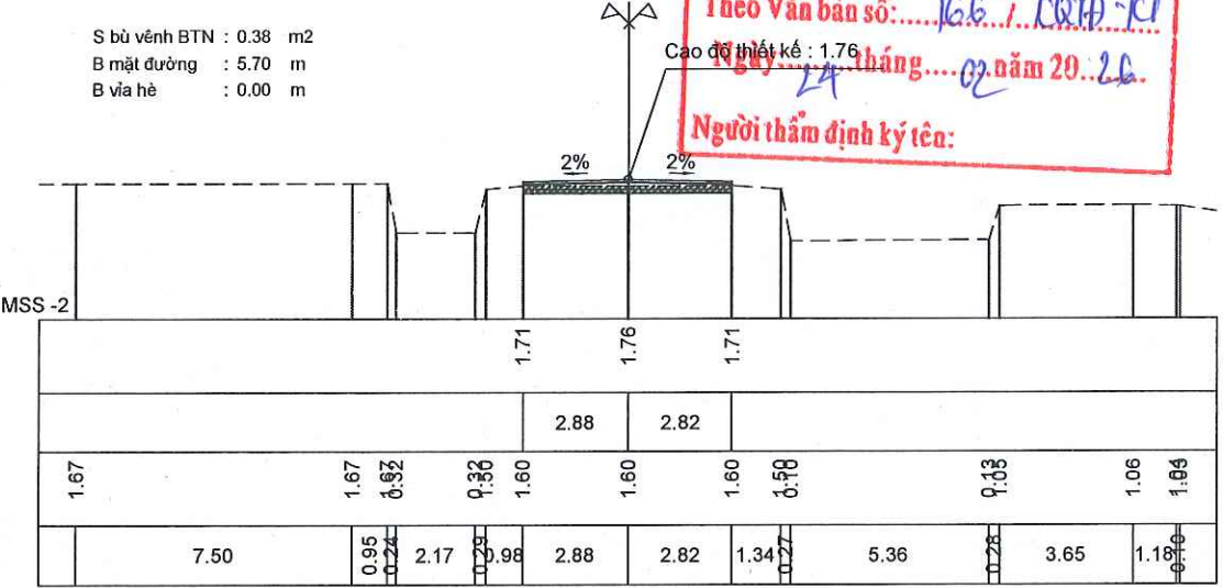
Cọc 9 Km 0 + 260.00 Cao độ :1.60
