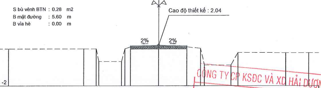
Cọc D3 Km 0 + 179.72 Cao độ :1.89
