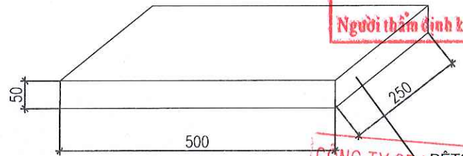
TẦM ĐẠN RÃNH BTXM M300 ĐÁ 1X2
