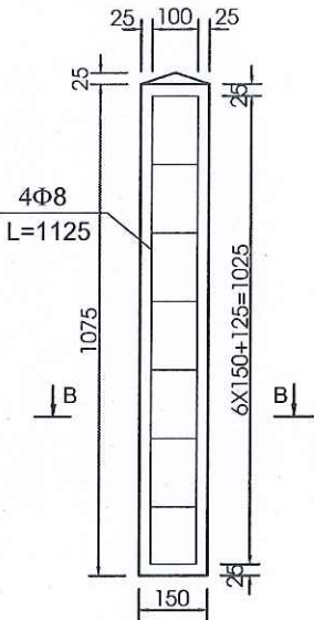
BỐ TRÍ CỐT THÉP
