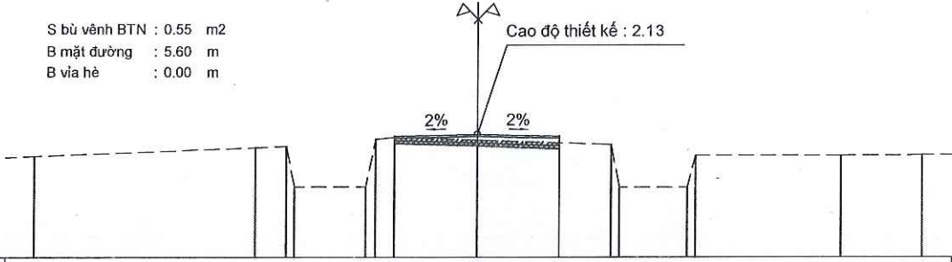
Cọc 5 Km 0 + 140.00 Cao độ :1.94
