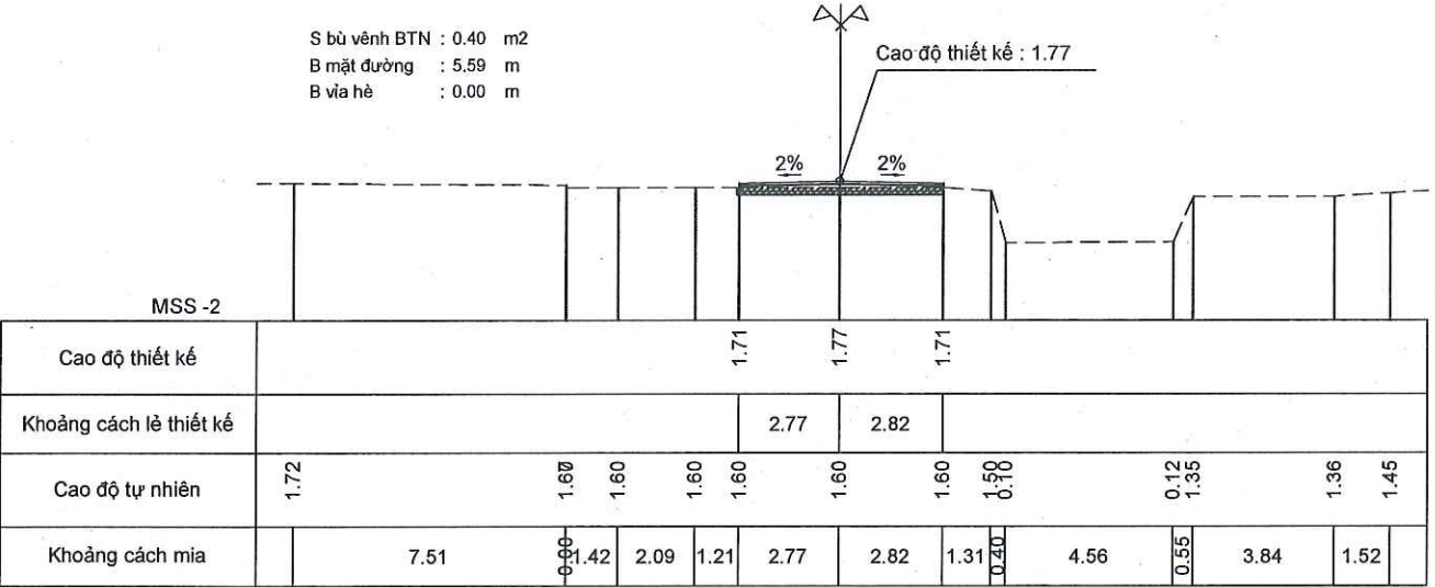
Cọc 8 Km 0 + 240.00 Cao độ :1.60
