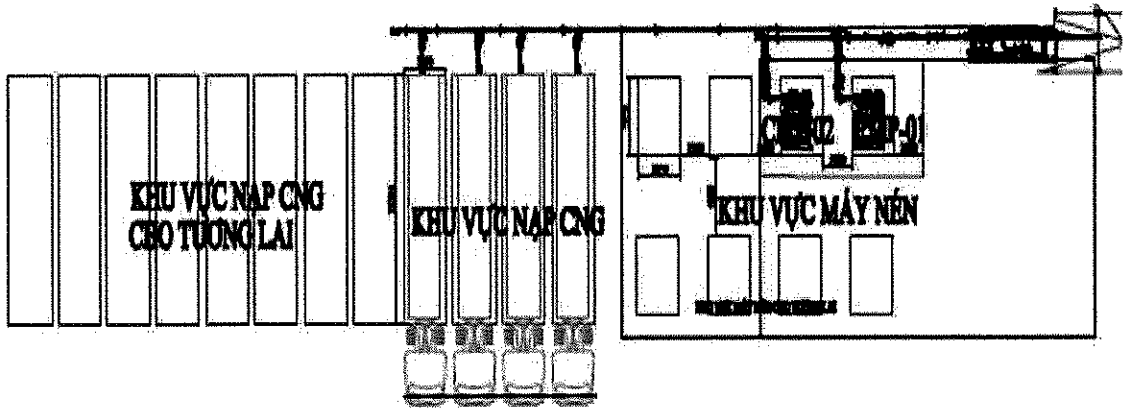
Hình ảnh: Sơ đồ ý tưởng trạm nén CNG tại GPP Cà Mau
