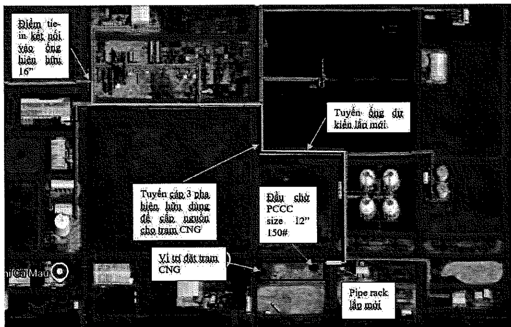
Hình ảnh: vị trí lắp đặt trạm nén CNG
