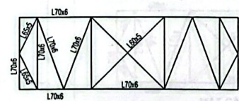
MAT CẮT 2-2
