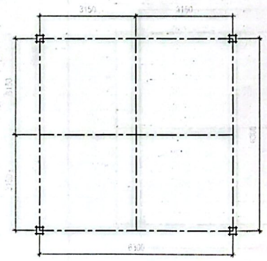
MAT BẢNG ĐỊNH VỊ CHÂN CỘT
