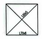
MAT CẮT 3-3
