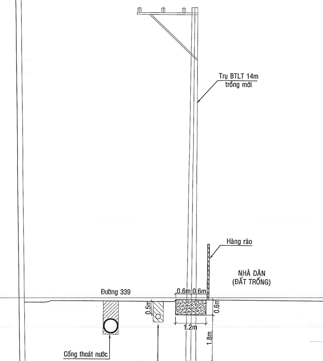
MẶT CẮT NGANG ĐIỂN HÌNH KHU VỰC ĐƯỜNG 46 ĐOẠN TRƯ TRƯ THỐNG MỚI X.BỐT/T14C/1C ĐẾN TRỤ X.BỐT/T14C/5C
