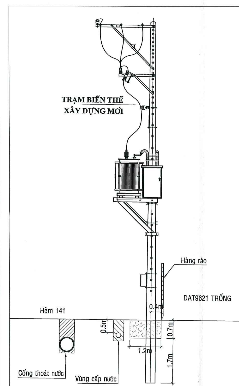
MẶT CẮT NGANG ĐIỂN HÌNH VỊ TRÍ TRẠM PHÚ HỮU 2/4 XÂY DỰNG MỚI
