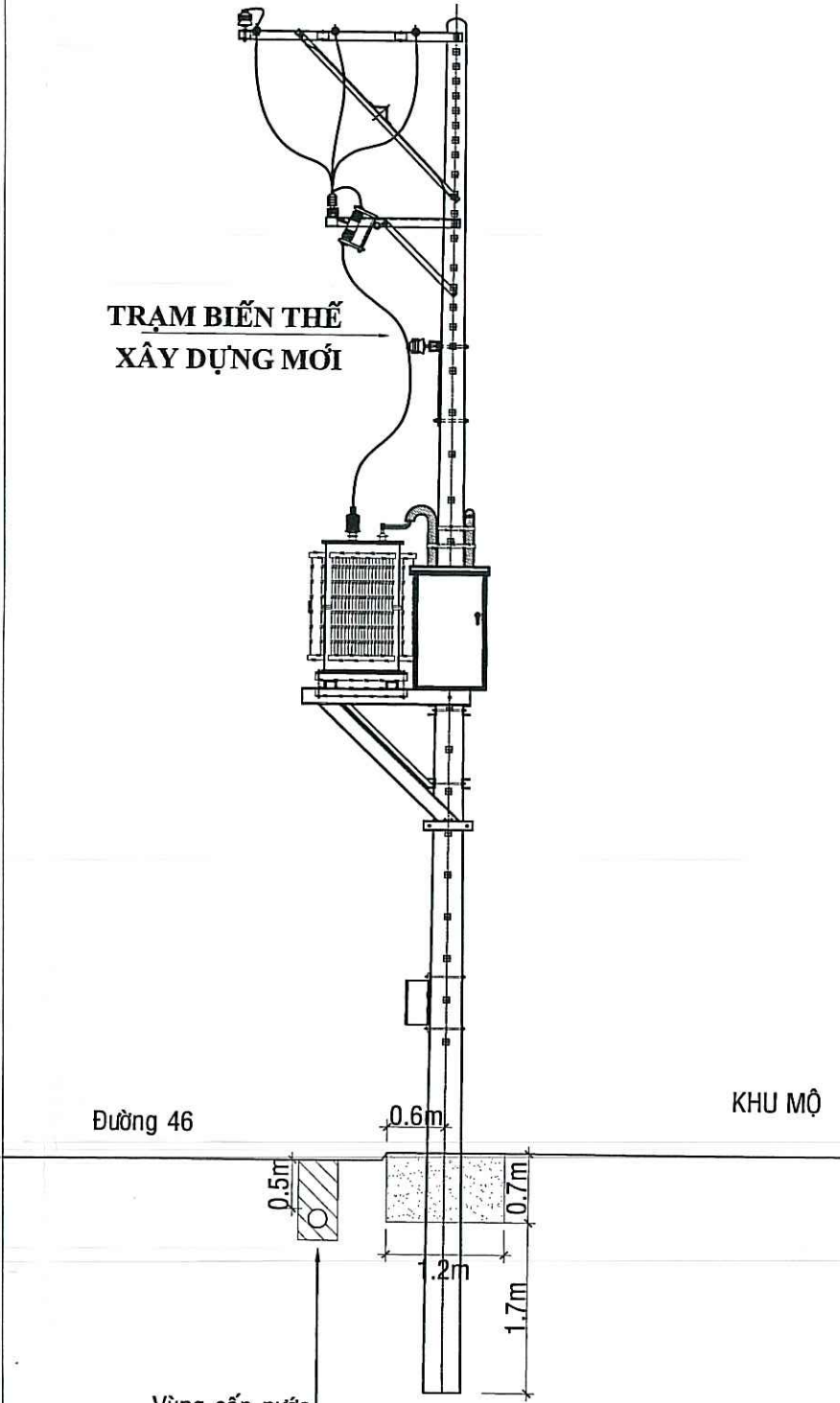
MẶT CẮT NGANG ĐIỂN HÌNH VỊ TRÍ TRẠM TÂN ĐIỆN 2 XÂY DỰNG MỚI
