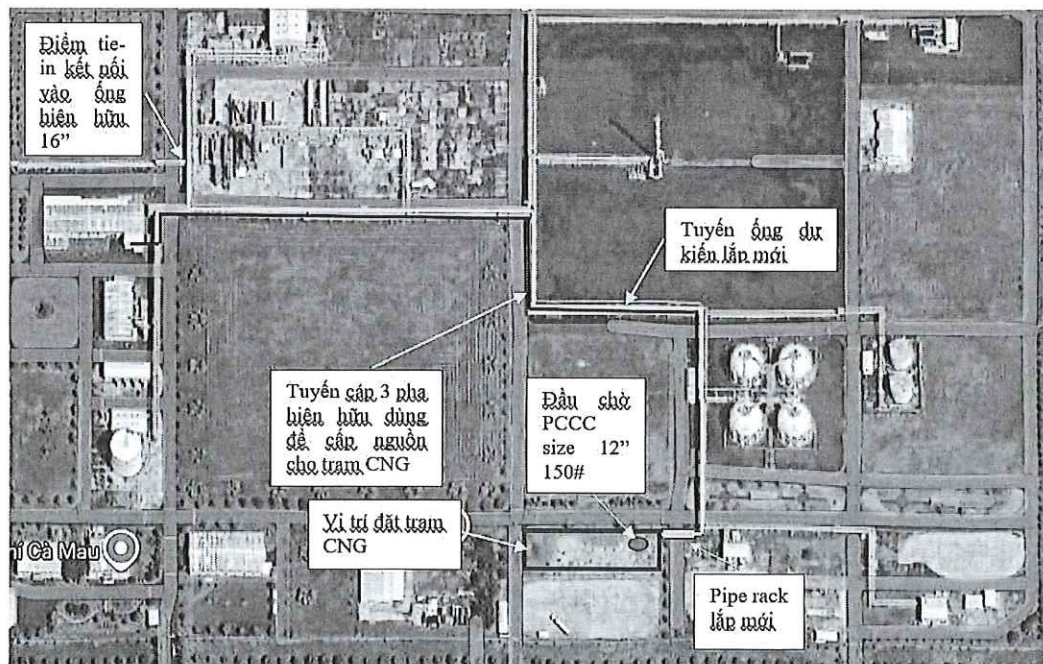
Hình ảnh: Sơ đồ ý tưởng tuyến ống lắp mới
