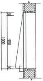
MẶT CẮT 2-2
