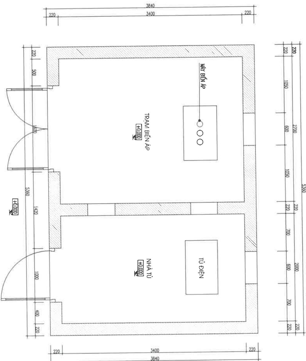
MẶT BẰNG TRẠM HIỆN TRẠNG
