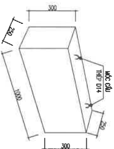
CỤC KẾ MÁY BIẾN ÁP
