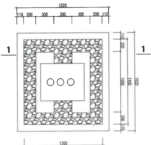
MẶT BẰNG CỤC KÊ MÁY BIẾN ÁP
