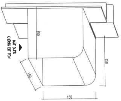
MẶT CẮT 1-1
