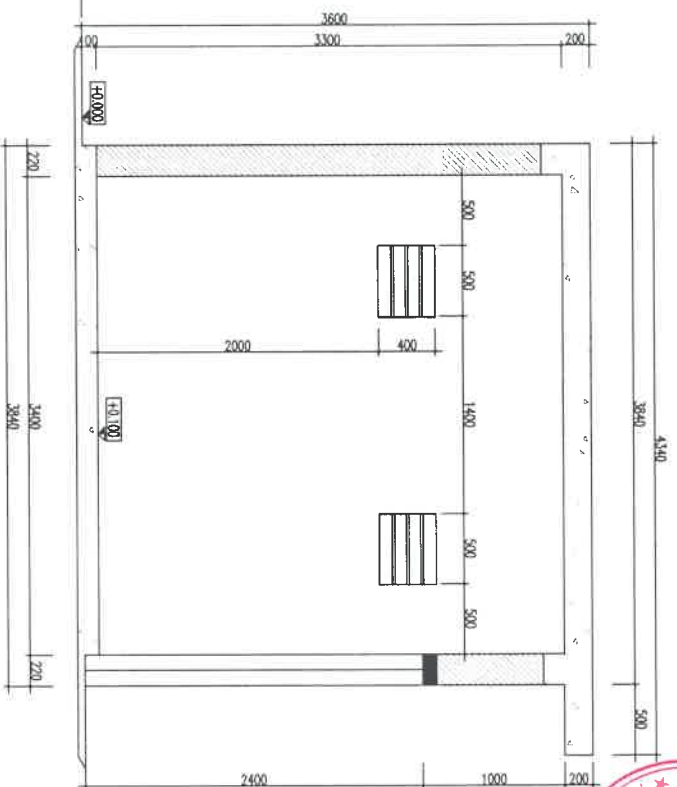
MẶT CẮT 1-1
