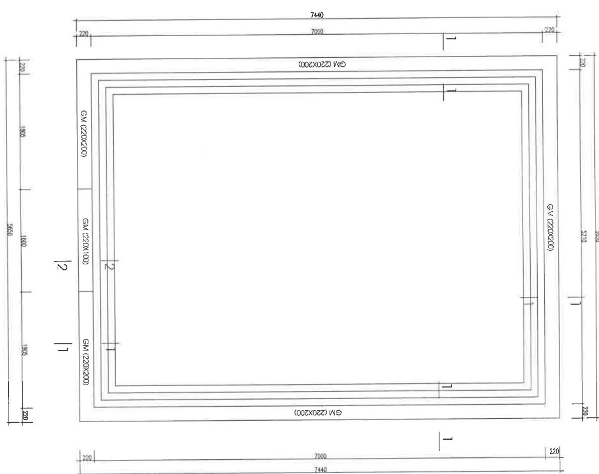
MẶT BẰNG MÔNG + GIẢNG MÔNG TƯỜNG RÀO
