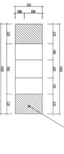
MẶT CẮT 3-3
