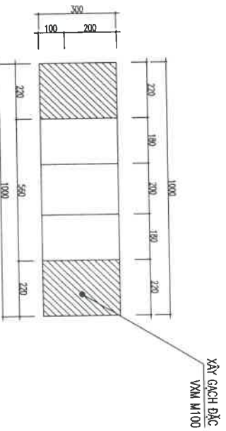
MẶT CẮT 3-3
