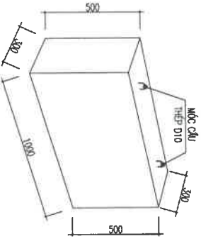
CỤC KÊ MÁY BIẾN ÁP - BỐ BỊC - SỐ LƯỢNG 2 CỤC
