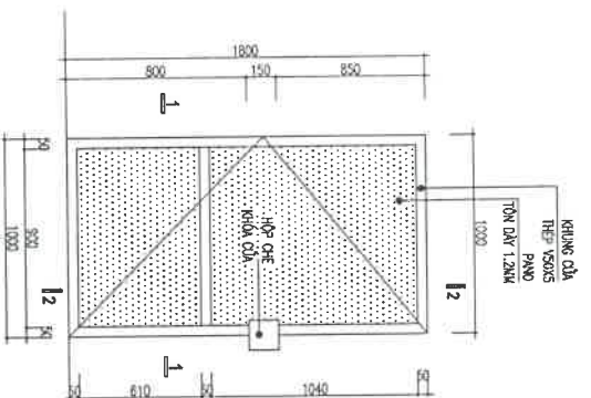
CỬA NHÀ TỬ
