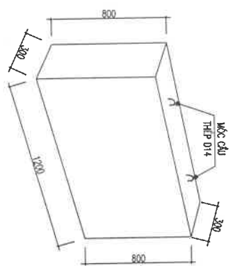
CỤC KÊ MÁY BIẾN ÁP - Ø BỐT - SỐ LƯỢNG 2 CỤC
