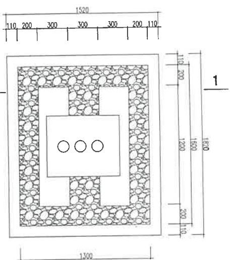
MẶT BẰNG CỤC KÊ MÁY BIẾN ÁP
