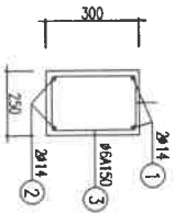
CỘT THÉP CỤC KẾ
