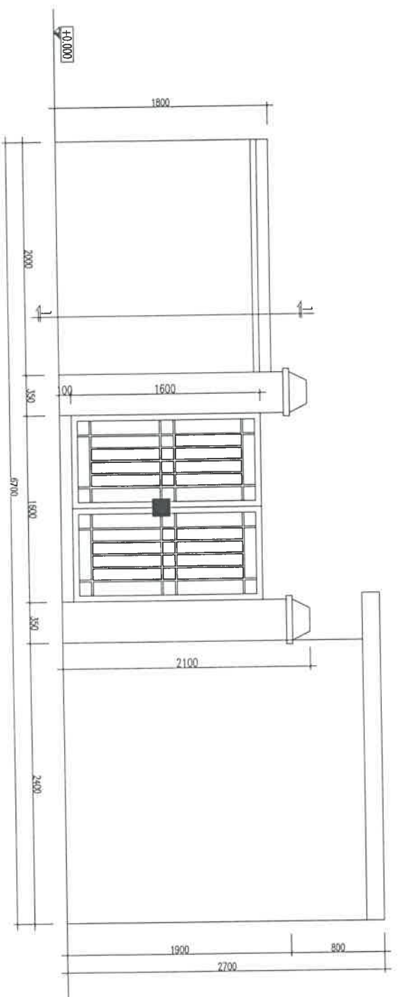
MẶT BẰNG TƯỜNG RÀO TRƯỚC
