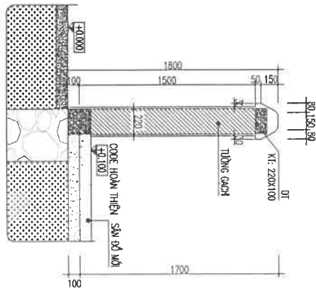
MẶT CẮT 1-1
