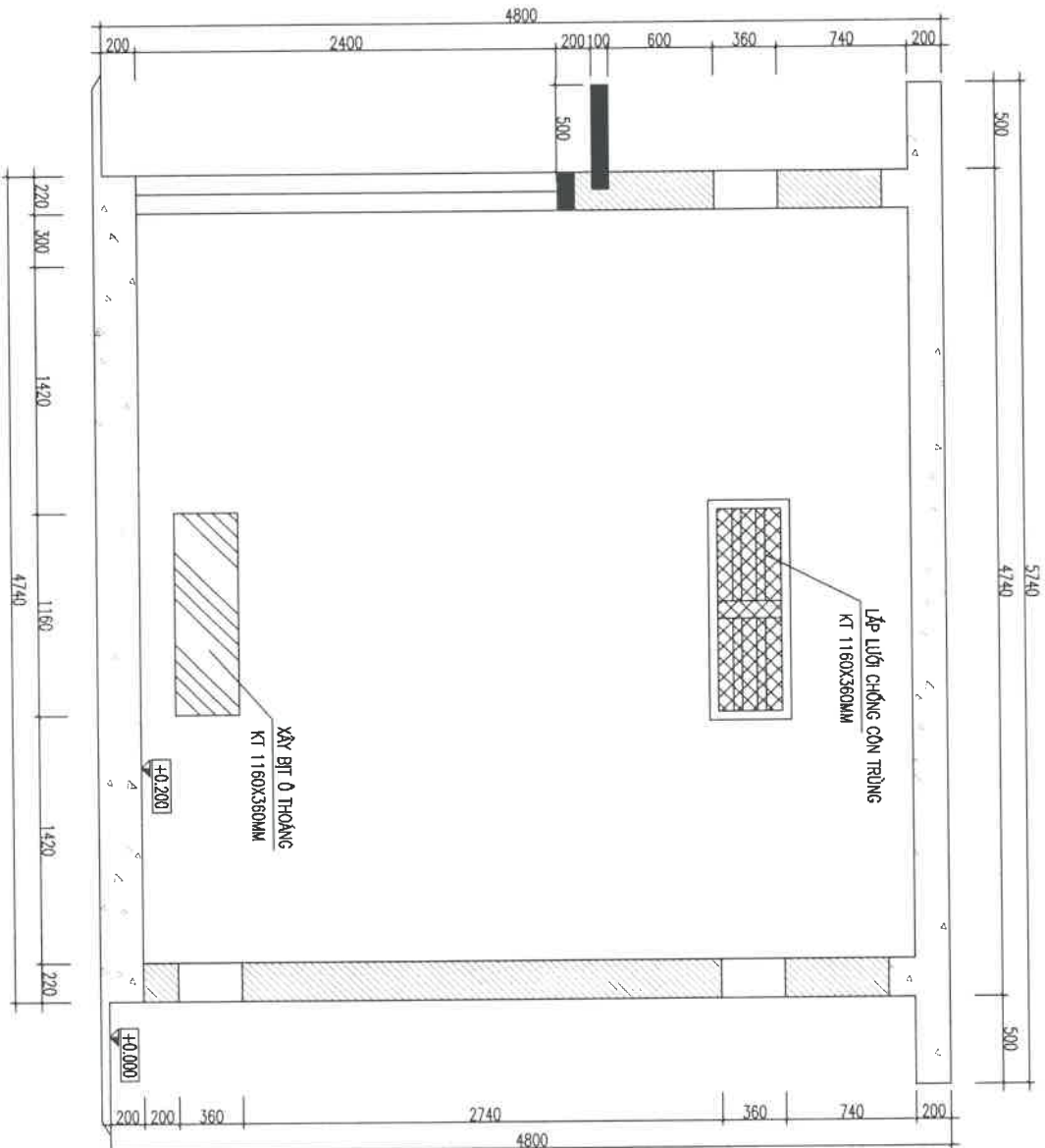
MẶT CẮT 2-2
