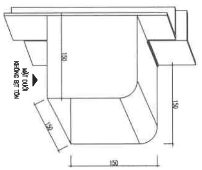
CHI TIẾT HỘCH CHE KHÓA CỬA
