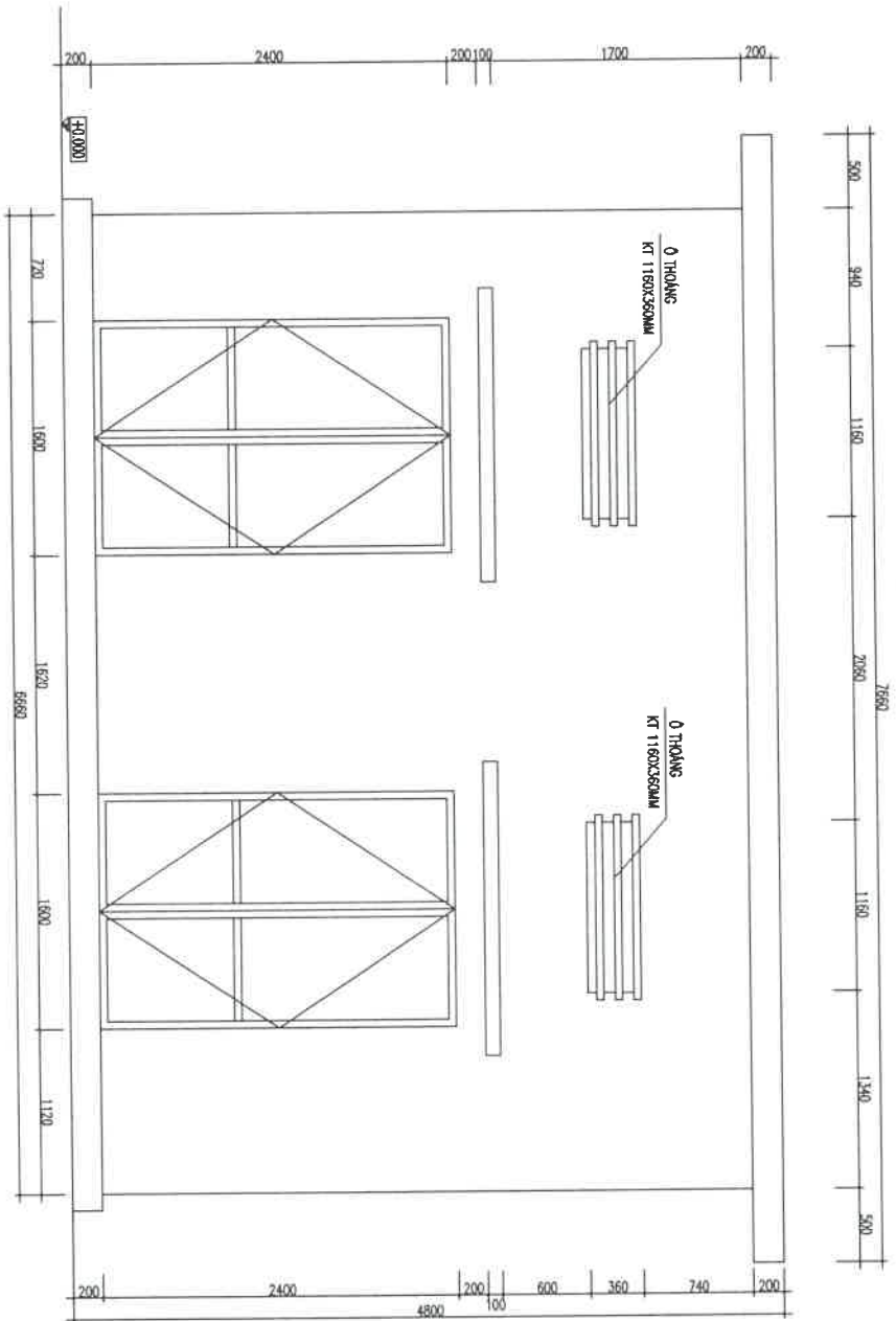
MẶT TRƯỚC TRẠM SỬA CHỮA
