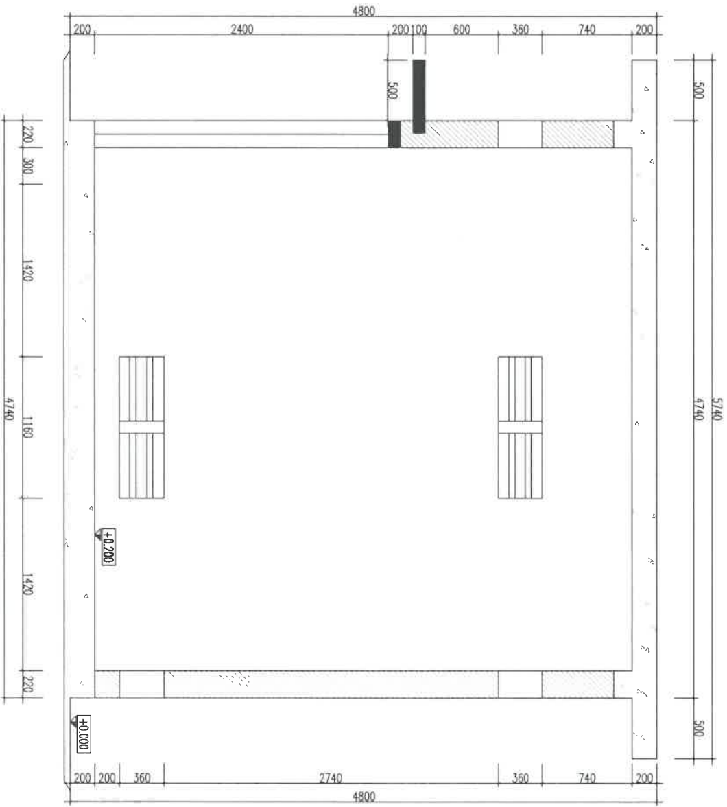
MẶT CẮT 2-2
