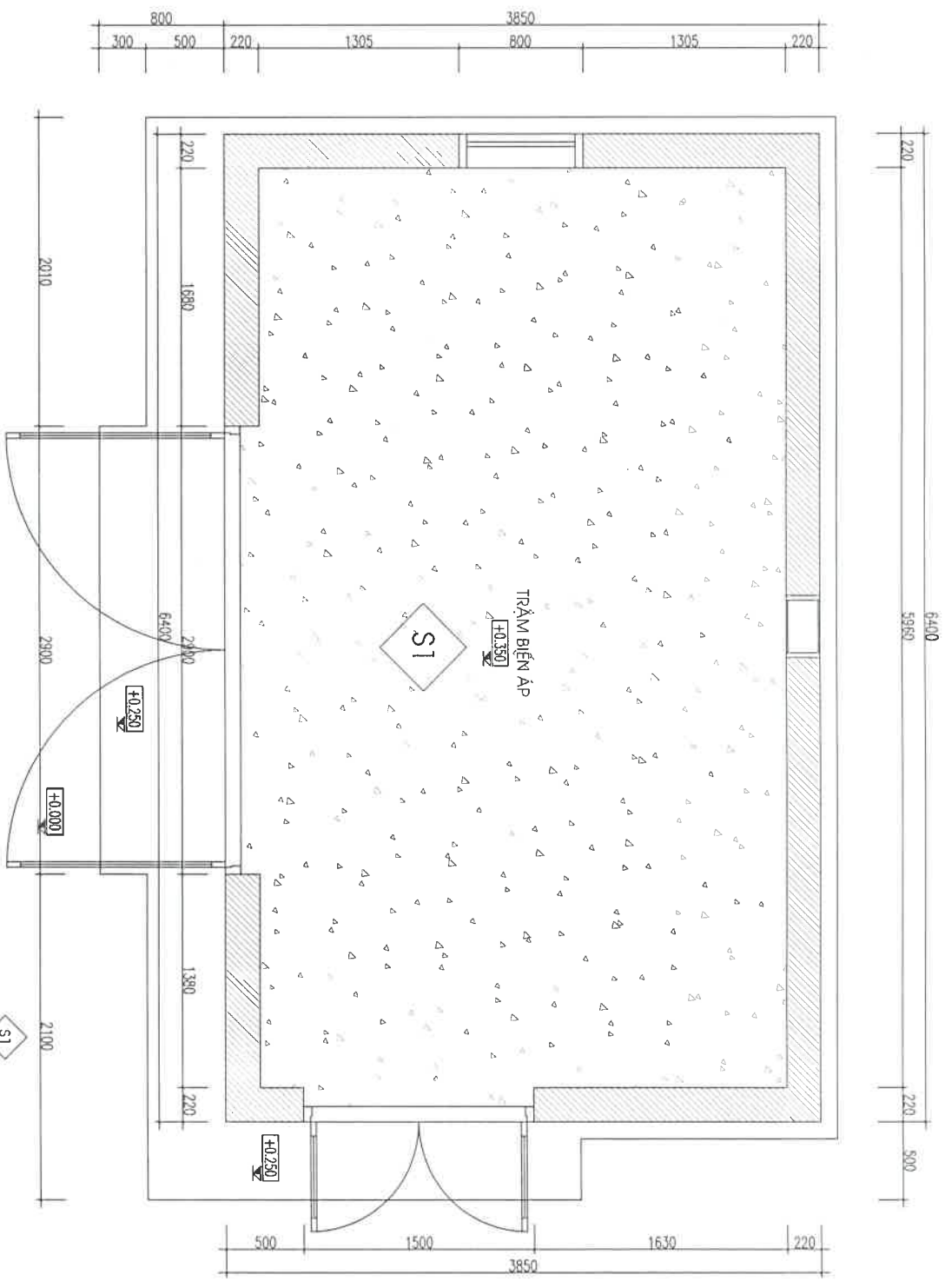
MẶT BẰNG ĐỒ BÊ TÊN TRẠM
