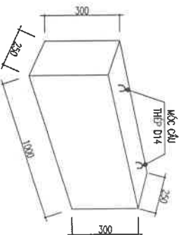
CỤC KÊ MÁY BIẾN ÁP
