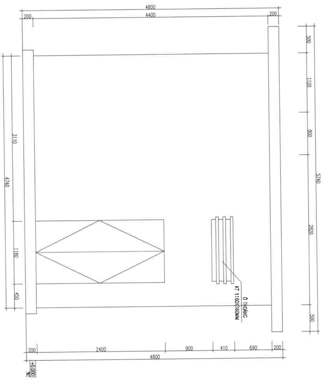
MẶT SAU TRAM HIỆN TRANG
