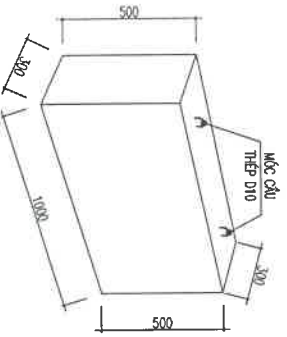
CỤC KÊ MÂY BIẾN ÁP - ĐỒ BỊT - SỐ LƯỢNG 2 CỤC
