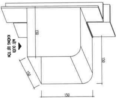
GHI TIẾT HỘCH CHE KHÓA CỬA
