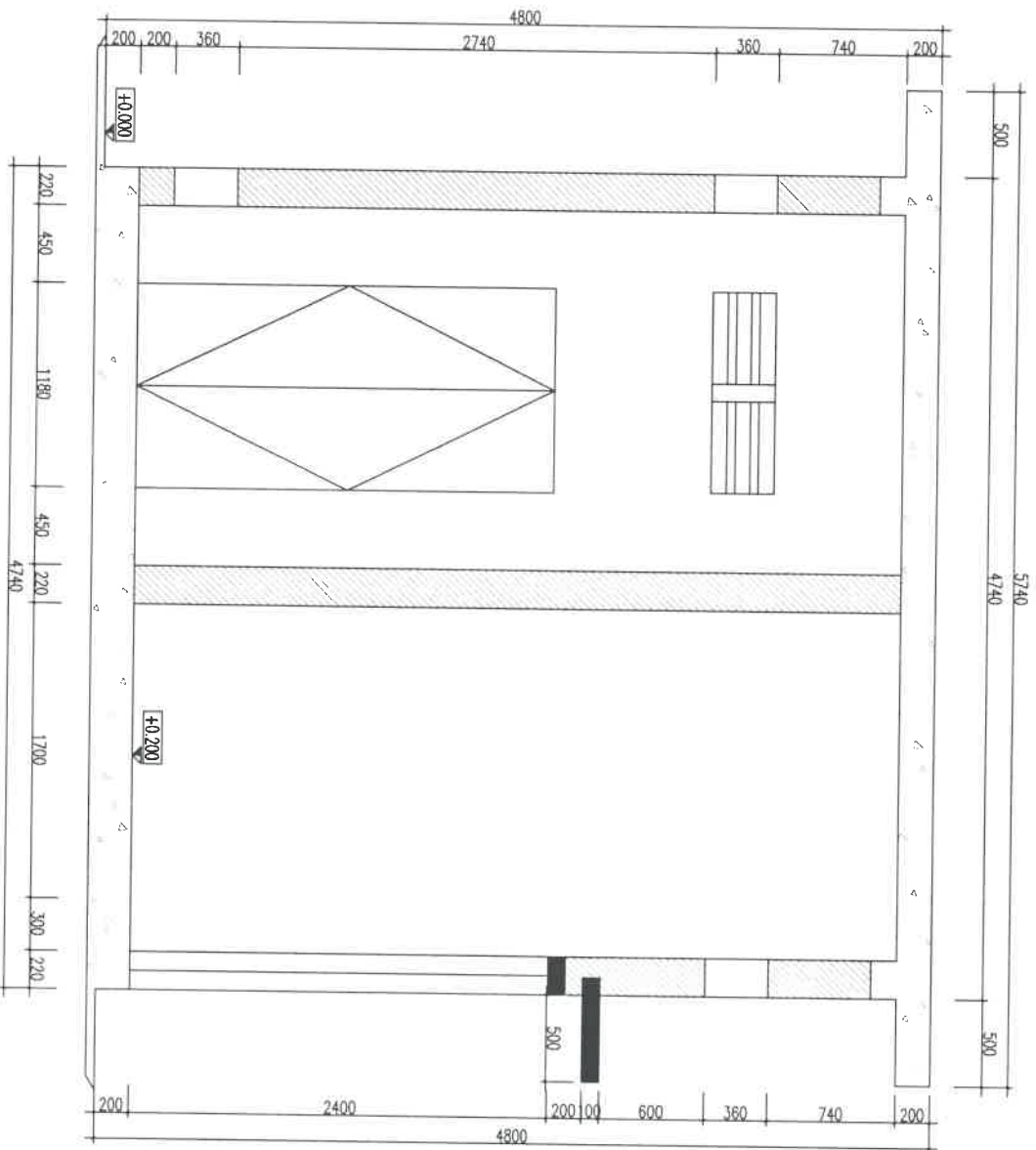
MẶT CẮT 3-3
