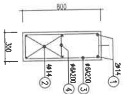
CỘT THÉP CỤC KÊ
