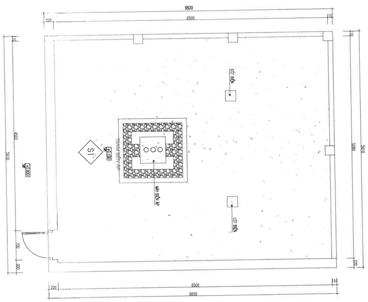
MẶT BẰNG ĐỔ BÊ TÔNG TRẠM
