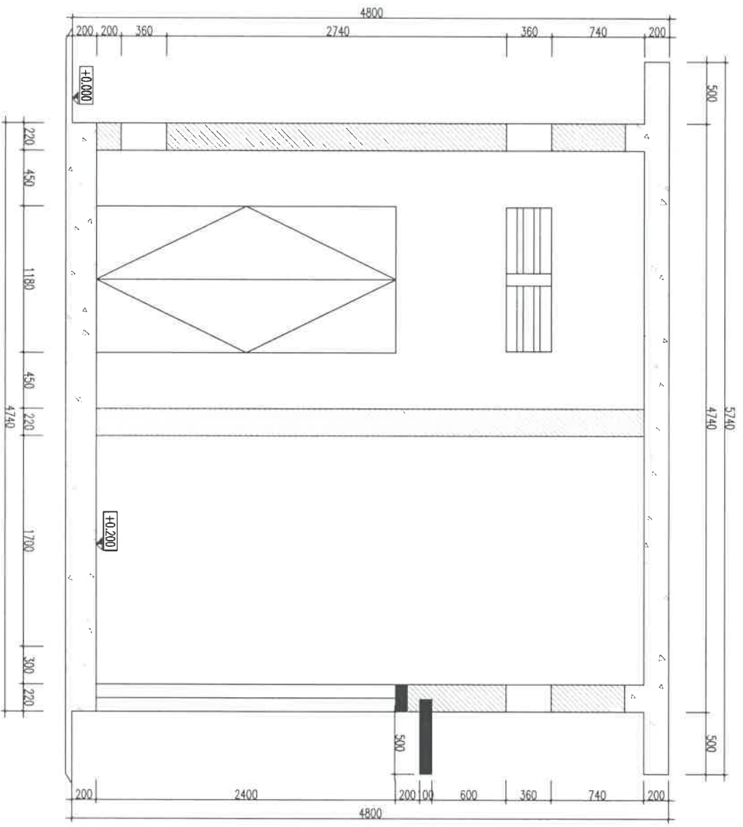
MẶT CẮT 3-3
