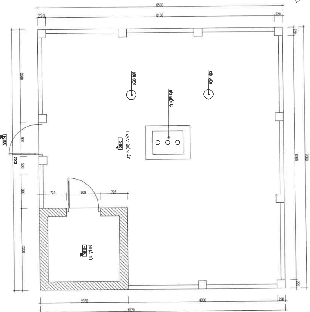
MẶT BẰNG TRẠM HIỆN TRẠNG
