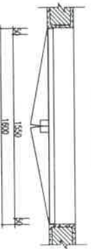
MẶT CẮT 2-2
