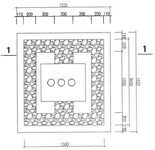
MẶT BẰNG CỤC KÊ MÂY BIẾN ÁP
