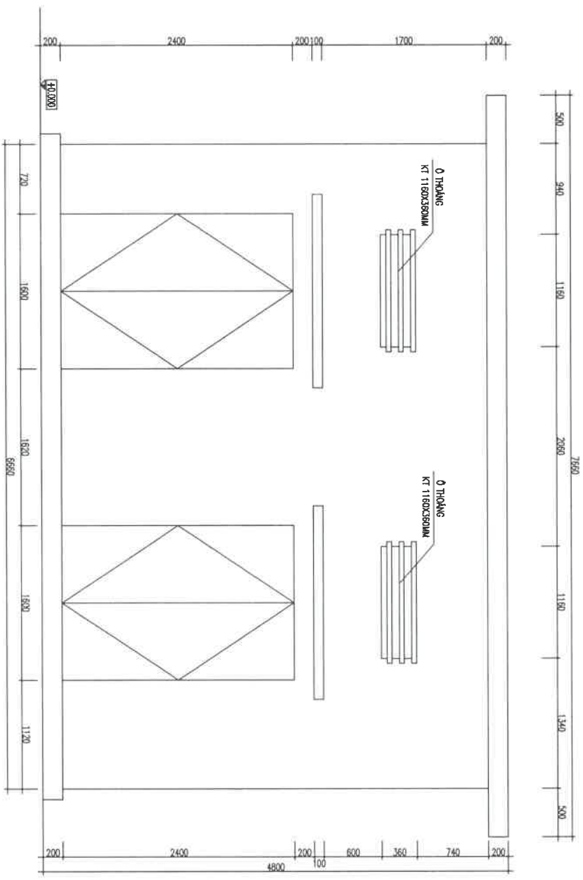
MẶT TRƯỚC TRẠM HIỆN TRẠNG
