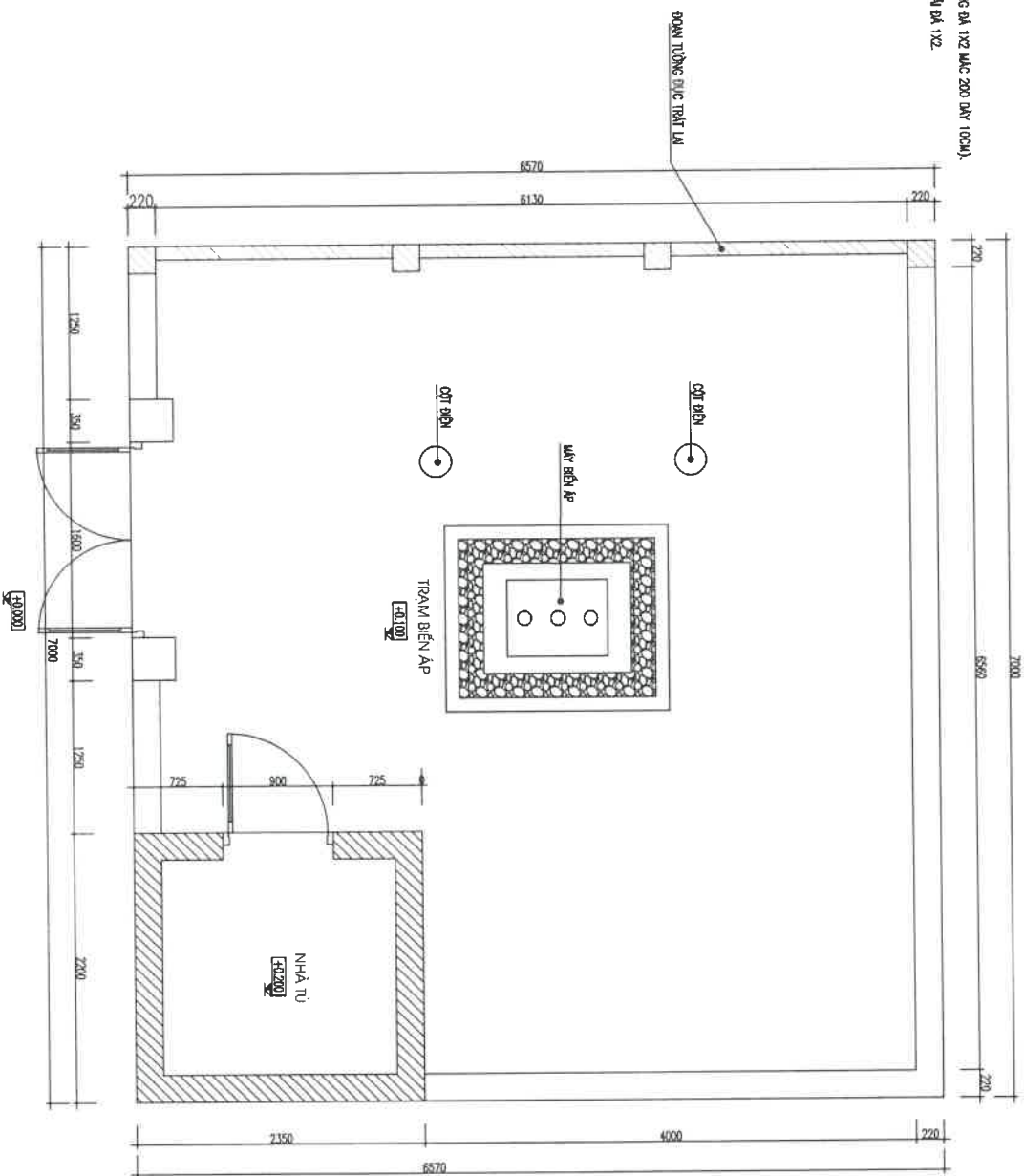
MẶT BẰNG TRẠM SỬA CHỮA
