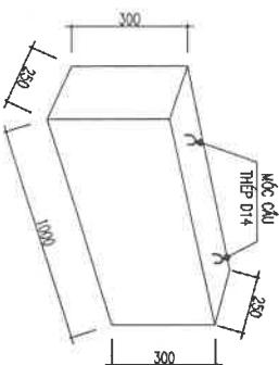
CỤC KẾ MÁY BIẾN ÁP
