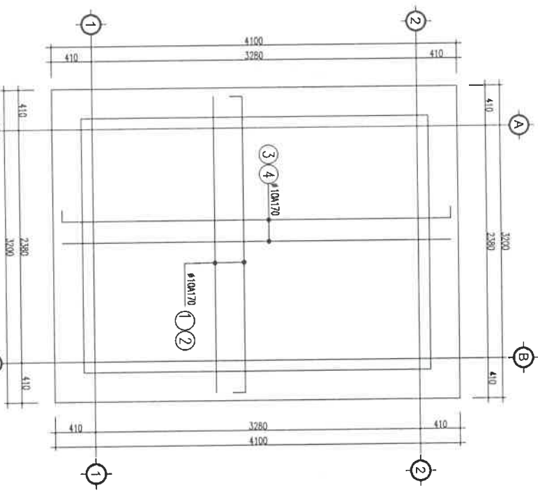
MẶT BẰNG DẪM SÀN MÁI
