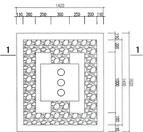
MẶT BẰNG CỤC KẾ MÁY BIẾN ÁP
