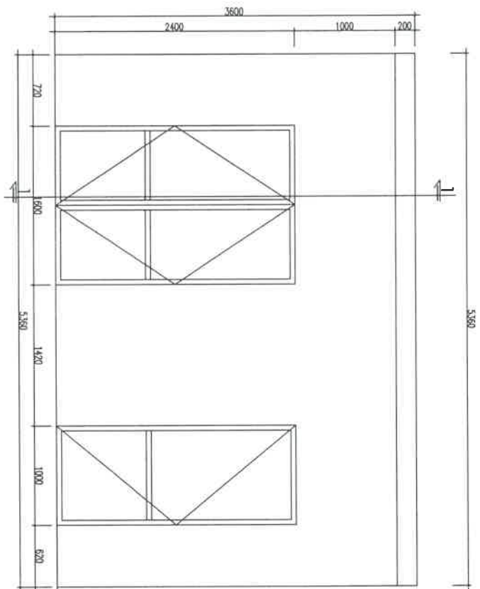
MẶT TRƯỚC TRAM SỬA CHỬA
