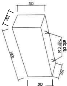
CỤC KẾ MÁY BIẾN ÁP
