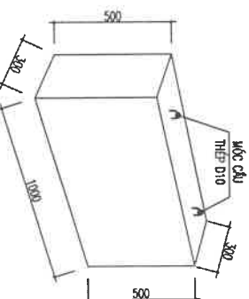
CỤC KÊ MÁY BIẾN ÁP
