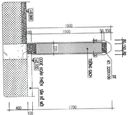
MẶT CẮT 1-1
