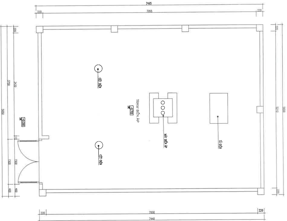
MẶT BẰNG TRẠM HIỆN TRĂNG
