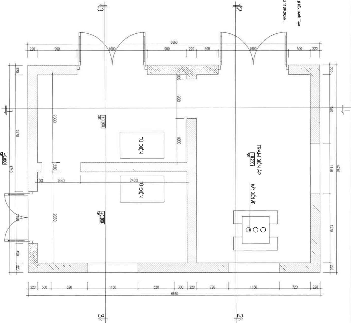
MẶT BẰNG TRẠM HIỆN TRẠNG
