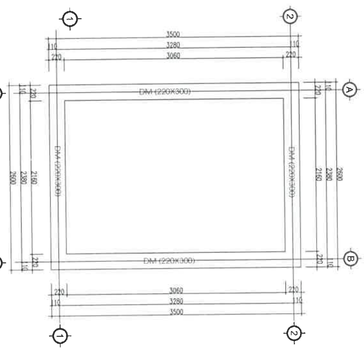
MẶT BẰNG DẪM SÀN MÁI
