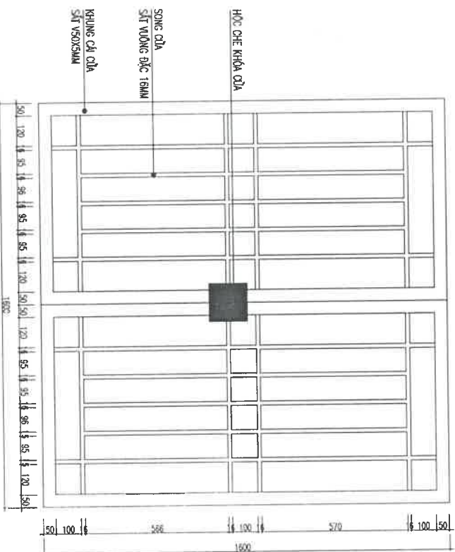
CỬA D1 (CỬA TRAM)
