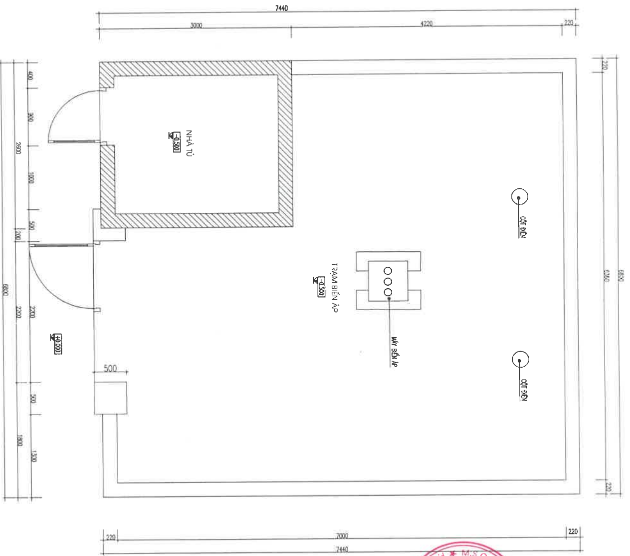
MẶT BẰNG TRẠM HIỆN TRẠNG
