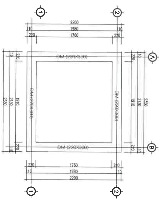
MẶT BẰNG DÂM SÀN MẶT
