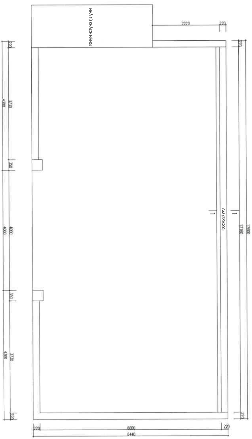
MẶT BẰNG MÔNG + GIẢNG MÔNG TƯỜNG RÀO ĐOẠN A-B
