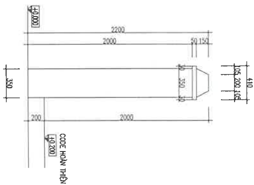
CHI TIẾT TRƯ TƯỜNG RÀO
