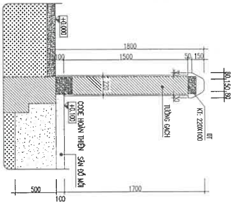
MẶT CẮT 1-1
