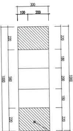
MẶT CẮT 3-3
