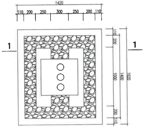
MẶT BẰNG CỤC KẾ MÁY BIẾN ÁP
