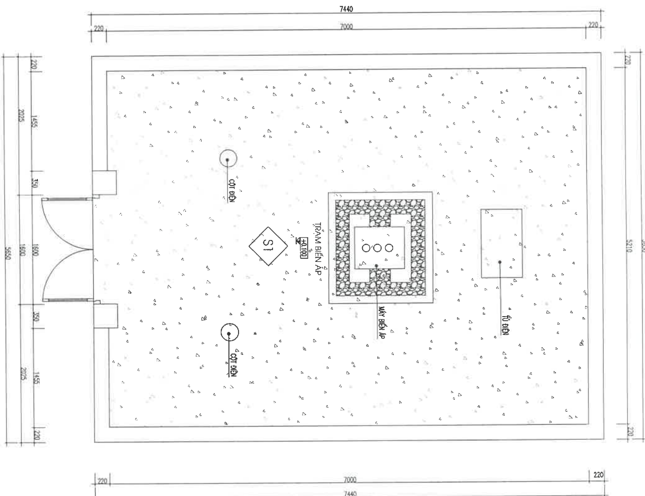
MẶT BẰNG ĐÓ BT NỀN TRAM
