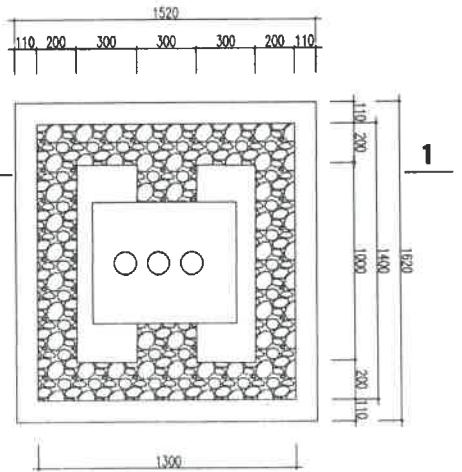
MẶT BẰNG CỤC KÊ MÁY BIẾN ÁP
