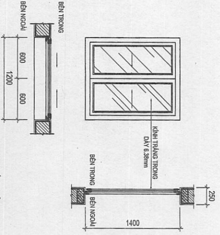
CHI TIẾT CỬA S2 - CHUÔNG LOẠI : CỬA NHỎM KÍNH ĐÌNH HÌNH - KÍNH TRẮNG TRONG DÀY 6.38mm - DAN DECAL MỜ - KÍCH THƯỚC : 1200X1400mm - SỐ LƯỢNG : 02 (B0)
