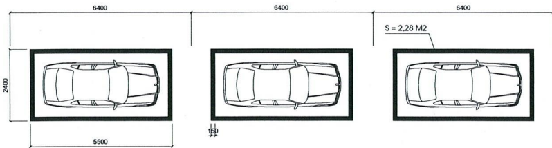
CHI TIẾT ĐỖ XE Ô TÔ (TỪ MC 1+440 ĐẾN MC1+590) (SỐ LƯỢNG: 25)
