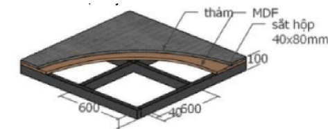
Chi tiết sàn nhà tiền chế
