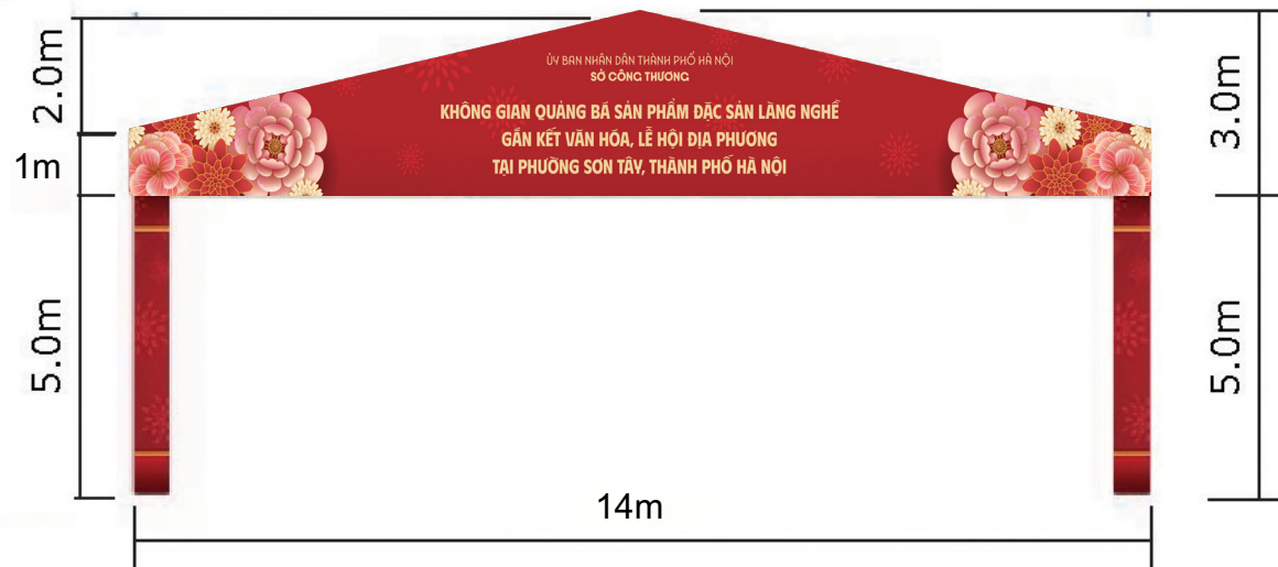
CHI TIẾT ỚP CỘT - TRẦN NGANG - TRẦN ĐẦU HỒI
