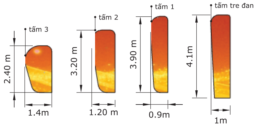
Tấm ốp trang trí 2 bên cổng
