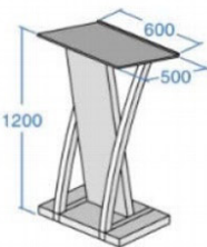
CHI TIẾT BỤC PHÁT BIỂU
