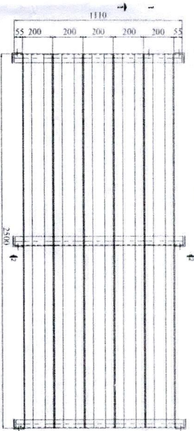
MAT CẮT 1-1 TL 1/10
