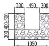
MẶT CẮT : 4-4 (L=20.5m)
