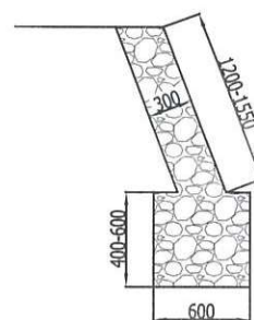
MẶT CẮT : 2-2
