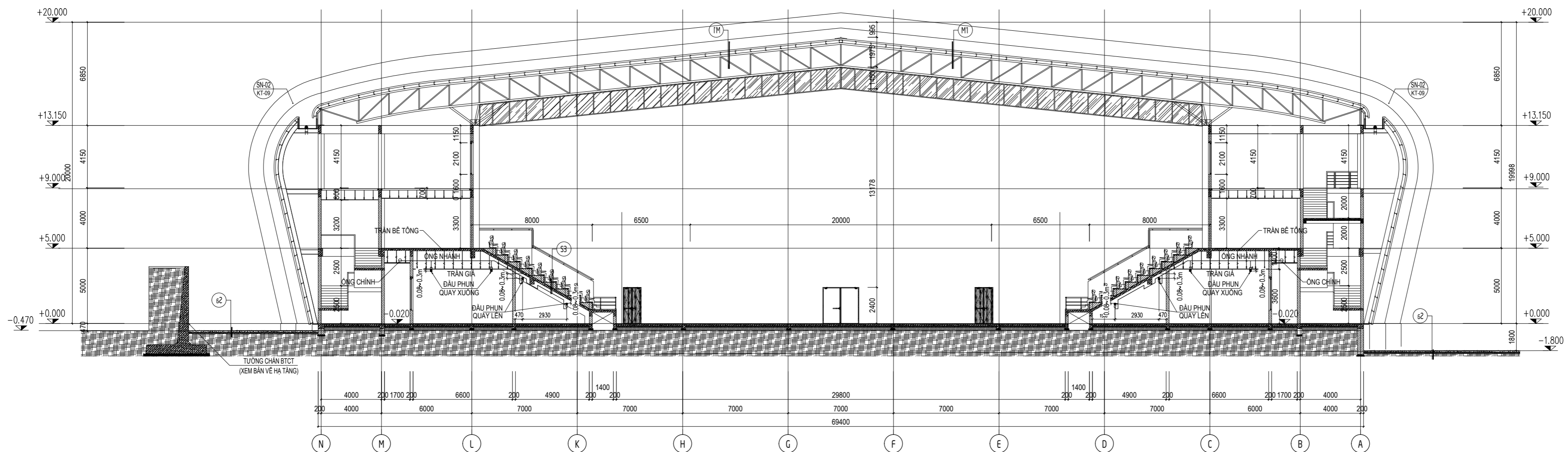
MẶT CẮT BỐ TRÍ ĐẦU PHUN ĐIỂN HÌNH
