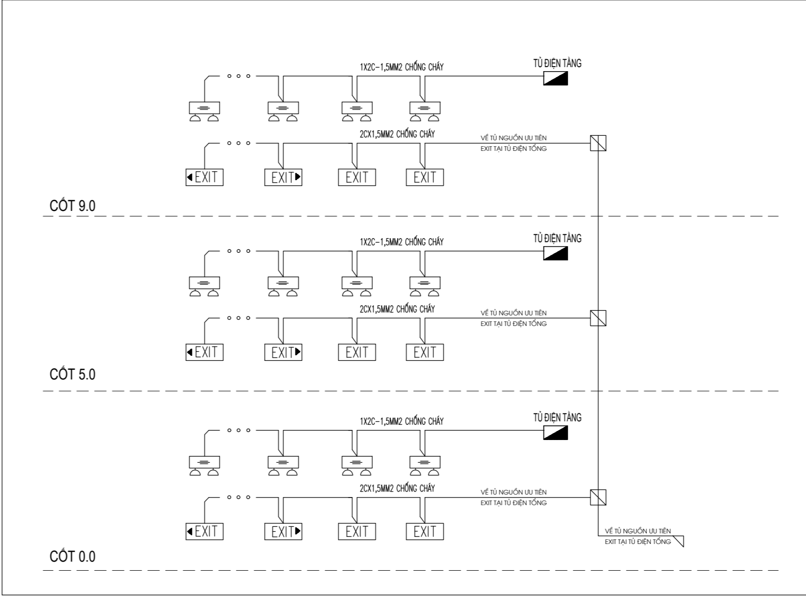
SƠ ĐỒ NGUYÊN LÝ HỆ THỐNG ĐÈN EXIT - SỰ CỐ
