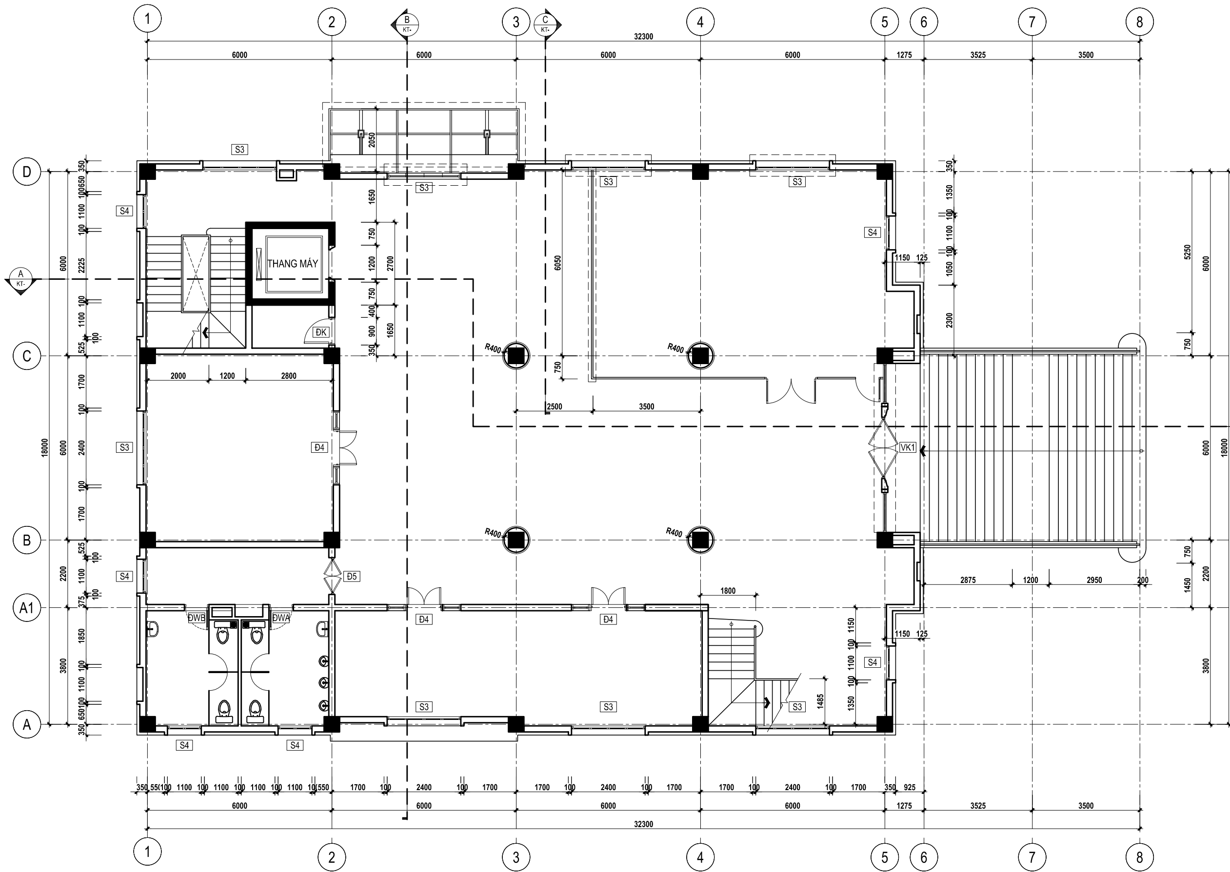
MẶT BẰNG TẦNG 1 HIỆN TRẠNG TL:1/100
