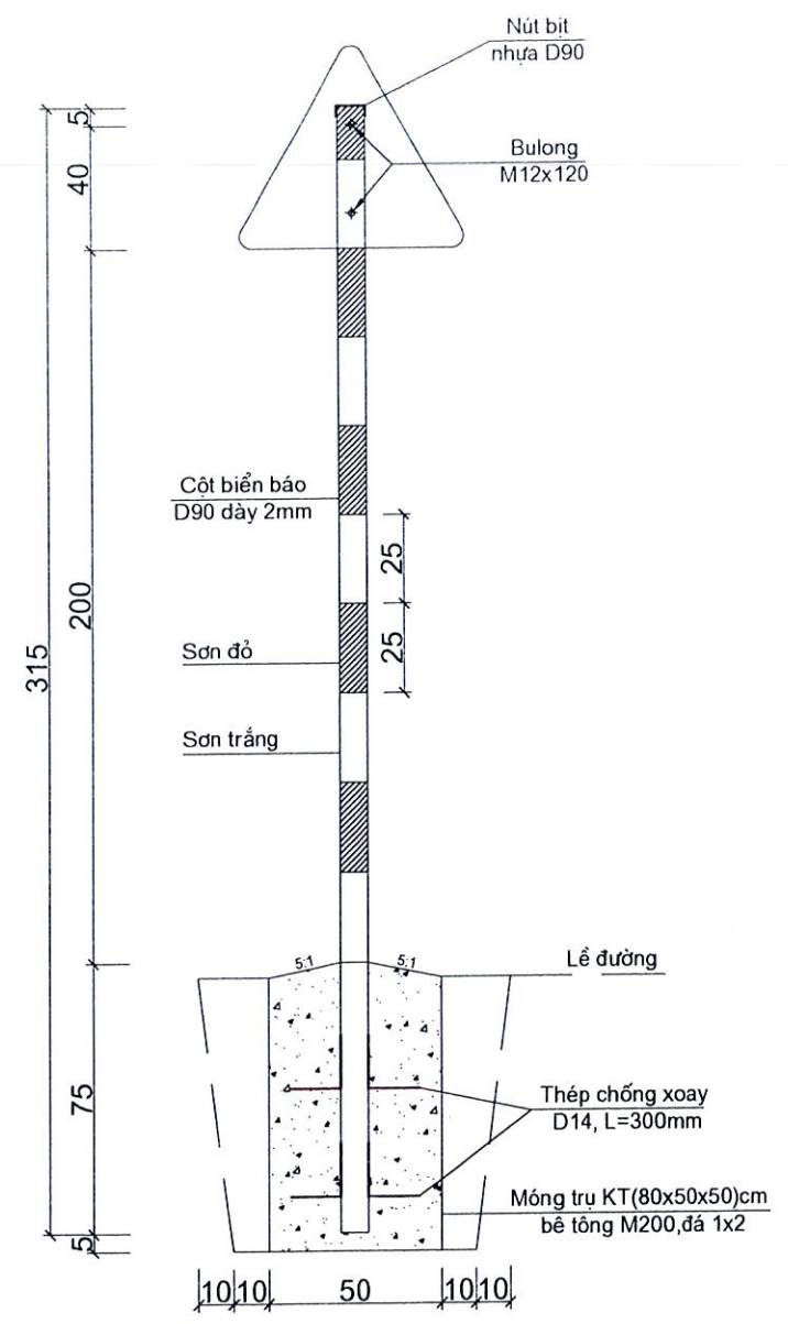
CHI TIẾT TRỤ BIỂN BÁO GẮN BIỂN BÁO TAM GIÁC (SL: 10CK)
