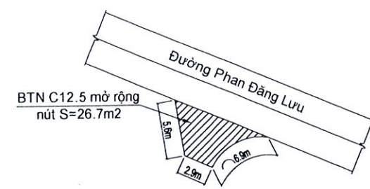
CHI TIẾT MỞ RỘNG NÚT GIAO ĐƯỜNG VÀO KHU DÂN CƯ TẠI CỘC SỐ 29
