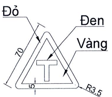
CHI TIẾT BIỂN W.205d ĐƯỜNG GIAO NHAU (SL: 01CK)
