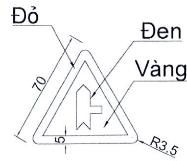
CHI TIẾT BIỂN W.207b GIAO NHAU VỚI ĐƯỜNG KHÔNG ƯU TIÊN (SL: 03CK)
