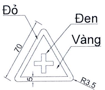
CHI TIẾT BIỂN W.205a ĐƯỜNG GIAO NHAU (SL: 01CK)
