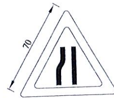
① BIỂN BÁO W.203a,b,c: ĐƯỜNG BỊ THẮT HẸP
