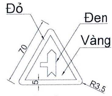
CHI TIẾT BIỂN W.207c GIAO NHAU VỚI ĐƯỜNG KHÔNG ƯU TIÊN (SL: 03CK)
