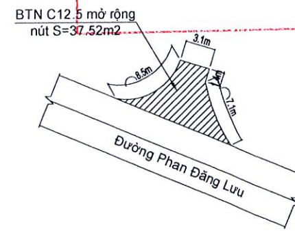
CHI TIẾT MỞ RỘNG NÚT GIAO ĐƯỜNG VÀO KHU DÂN CƯ TẠI CỘC SỐ 41
