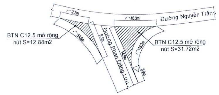
CHI TIẾT MỞ RỘNG NÚT GIAO ĐƯỜNG NGUYỄN TRẦN
