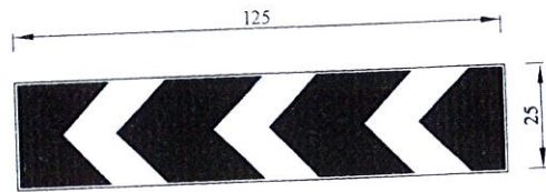
④ BIỂN BÁO S.507: HƯỚNG RẼ
