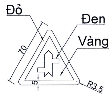
CHI TIẾT BIỂN W.207d GIAO NHAU VỚI ĐƯỜNG KHÔNG ƯU TIÊN (SL: 02CK)
