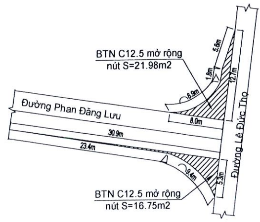
CHI TIẾT MỞ RỘNG NÚT GIAO ĐƯỜNG LÊ ĐỨC THỌ
