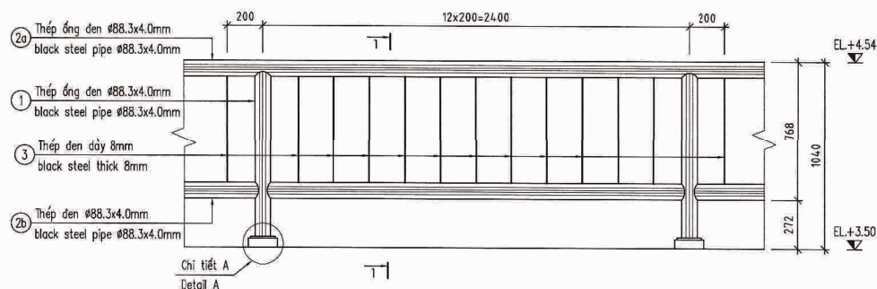
CHI TIẾT ĐOẠN 2,4M DETAIL OF SEGMENT 2.4M
