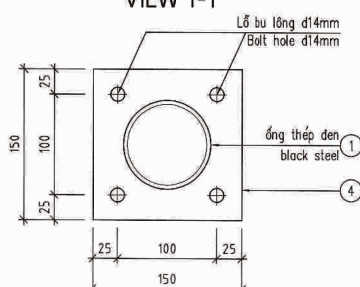
NHÌN THEO 1-1 VIEW 1-1
