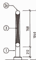
MẶT CẮT 1-1 SECTION 1-1
