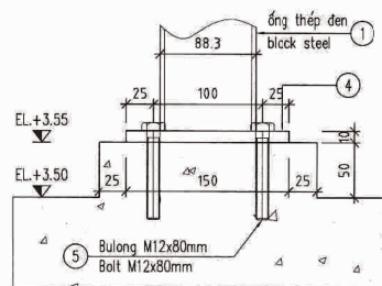
CHI TIẾT A/DETAIL A
