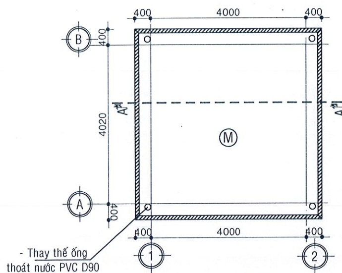
MẶT BẰNG THIẾT KẾ MÁI (TL: 1/100)
