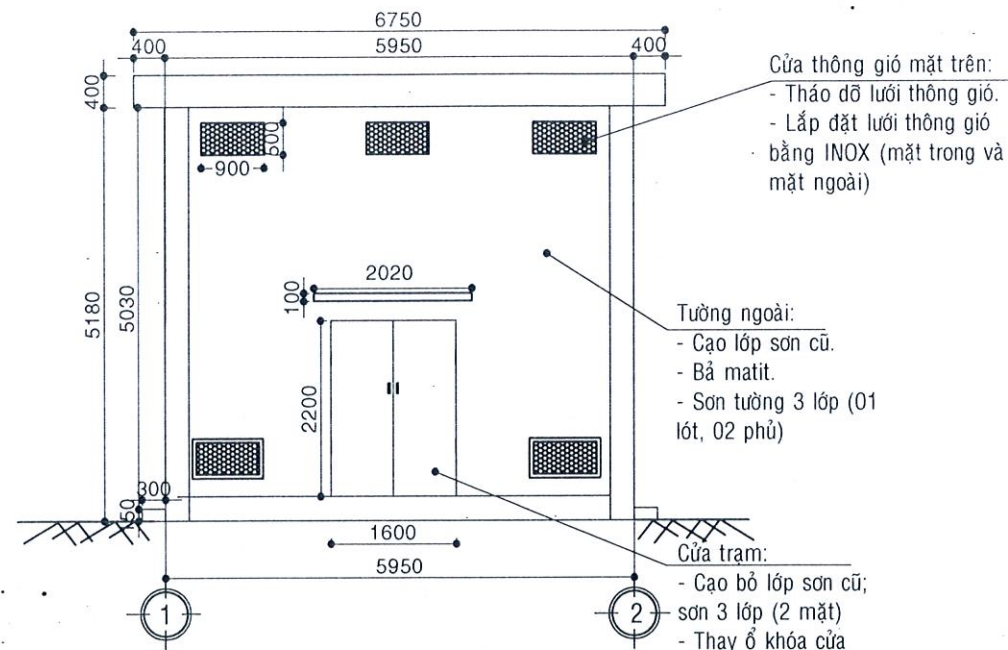
MẶT ĐỨNG THIẾT KẾ TRỤC 1-2 (TL: \frac{1}{100} )
