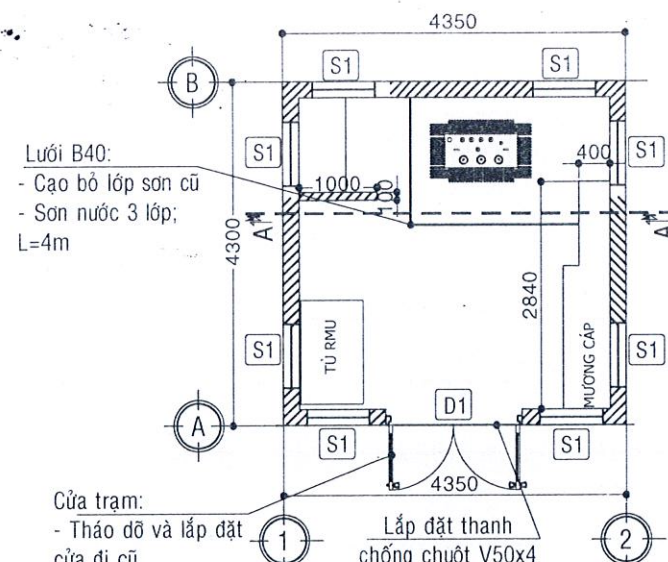
MẶT BẰNG THIẾT KẾ (TL: 1/100)
