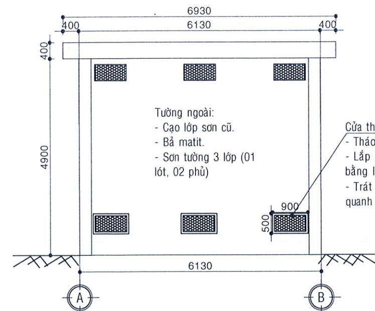
MẶT ĐỨNG THIẾT KẾ TRỤC A-B; B-A (TL: 1/100)
