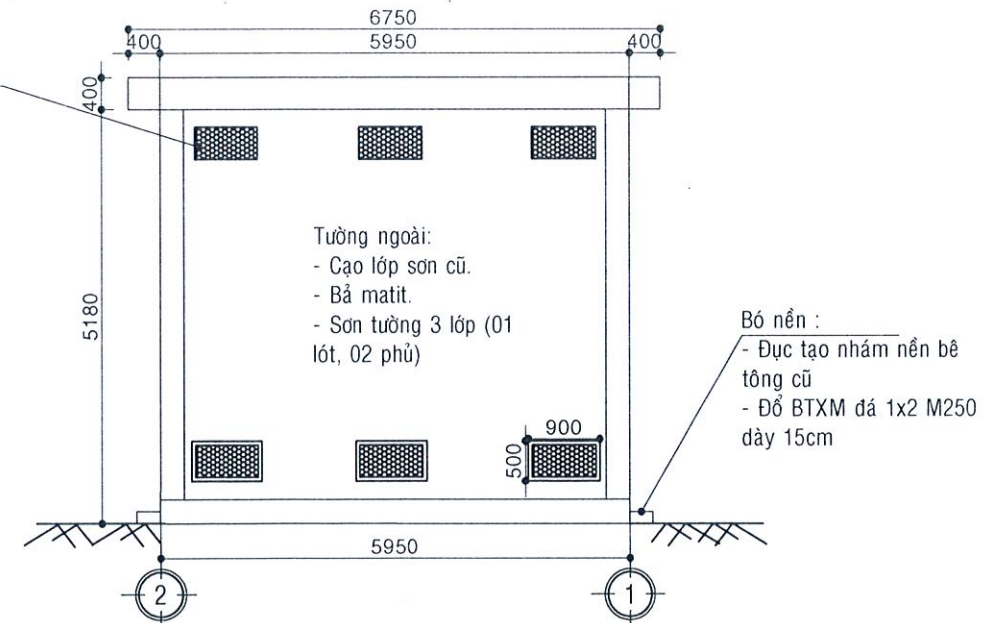
MẶT ĐỨNG THIẾT KẾ TRỤC 2-1 (TL: \frac{1}{100} )
