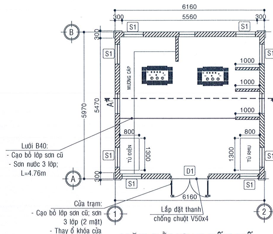
MẶT BẰNG THIẾT KẾ (TL: \frac{1}{100} )
