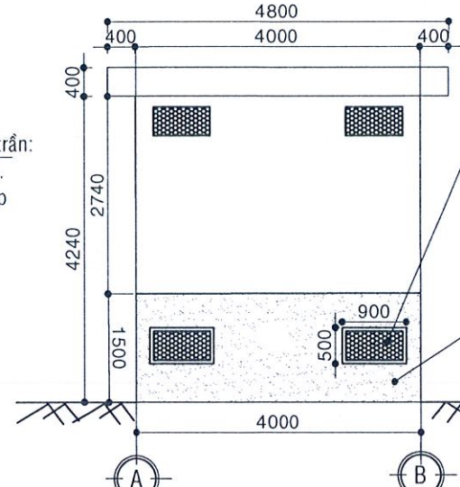
MẶT ĐỨNG THIẾT KẾ TRỤC A-B; B-A (TL: 1/100)
