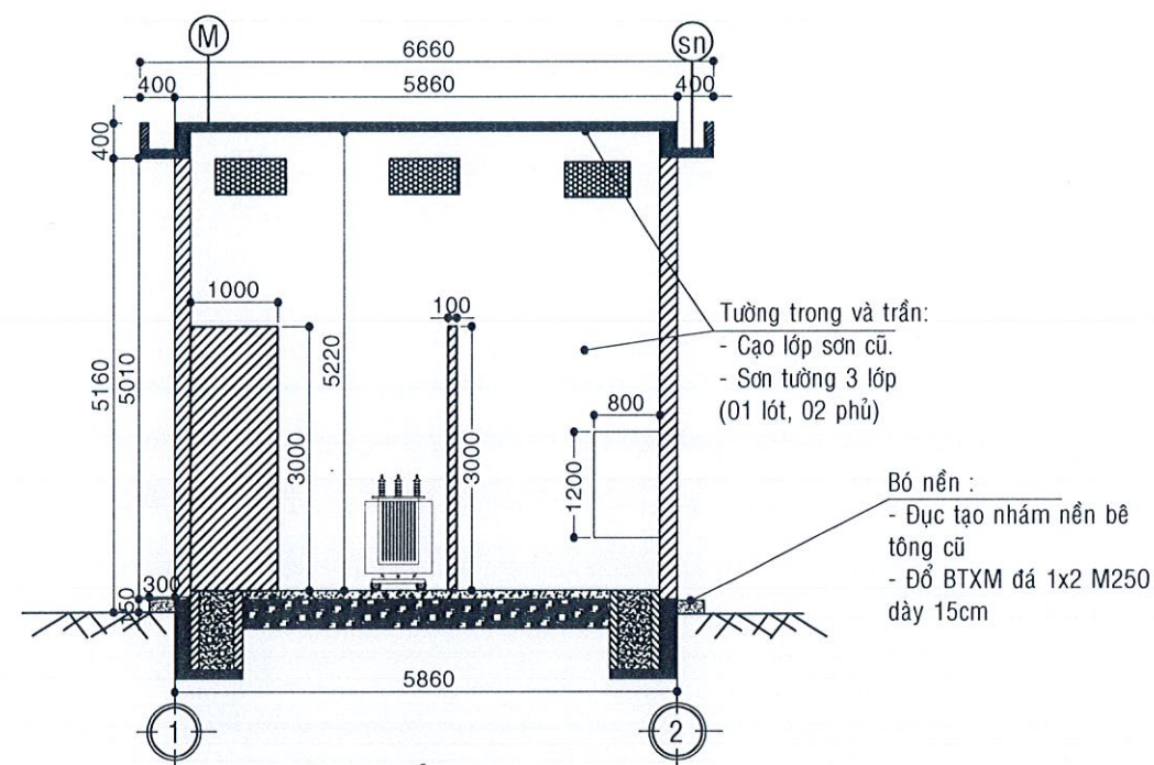
MẶT CẮT A-A (TL: \frac{1}{100} )
