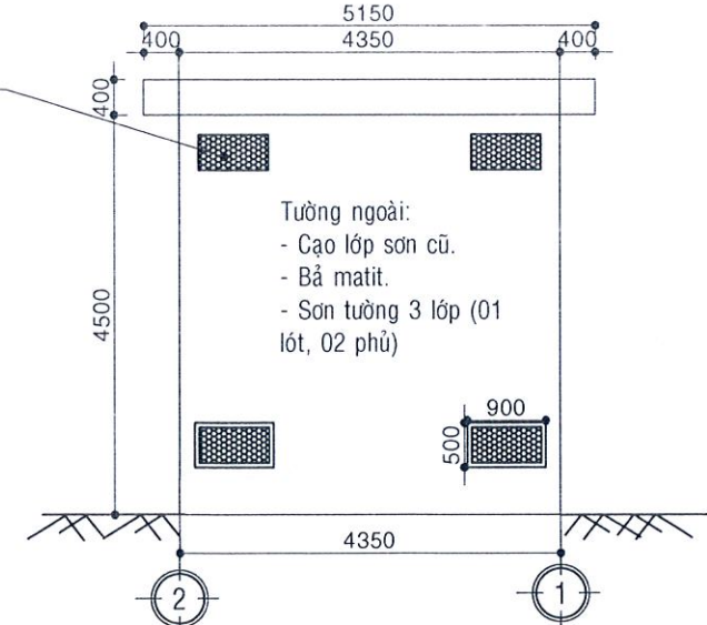
MẶT ĐỨNG THIẾT KẾ TRỤC 2-1 (TL: 1/100)
