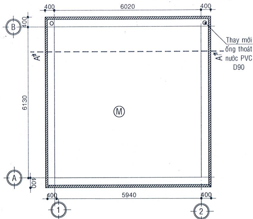
MẶT BẰNG THIẾT KẾ MÁI (TL: 1/100)
