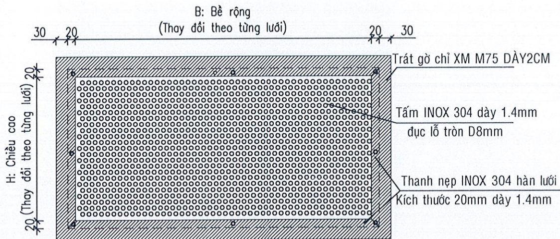
CHI TIẾT THIẾT KẾ LƯỚI THÔNG GIÓ (TL: 1/10)
