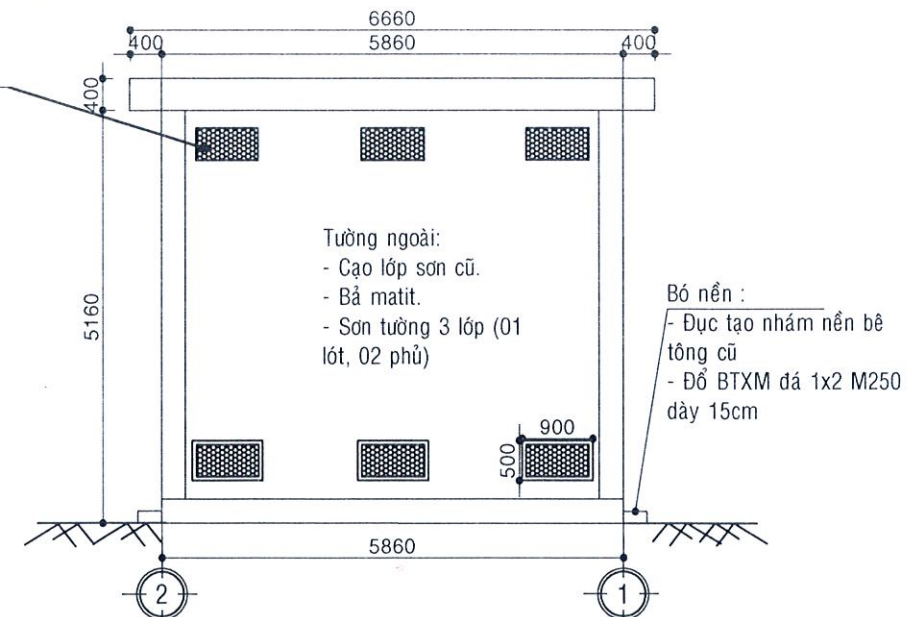
MẶT ĐỨNG THIẾT KẾ TRỤC 2-1 (TL: \frac{1}{100} )
