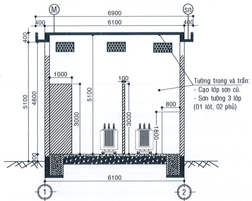
MẶT CẮT A-A (TL: \frac{1}{100} )
