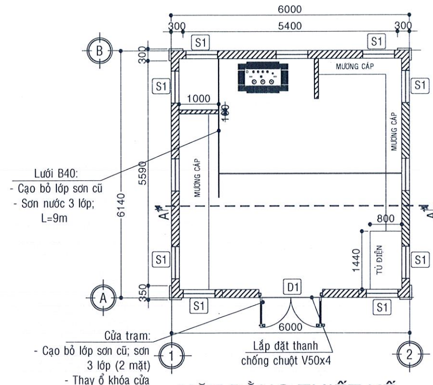
MẶT BẰNG THIẾT KẾ (TL: \frac{1}{100} )
