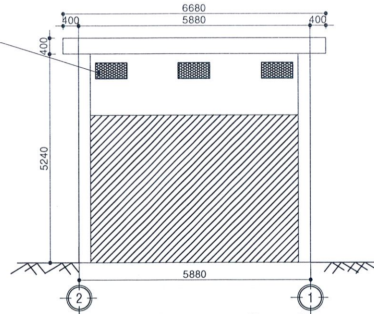
MẶT ĐỨNG THIẾT KẾ TRỤC 2-1 (TL: \frac{1}{100} )
