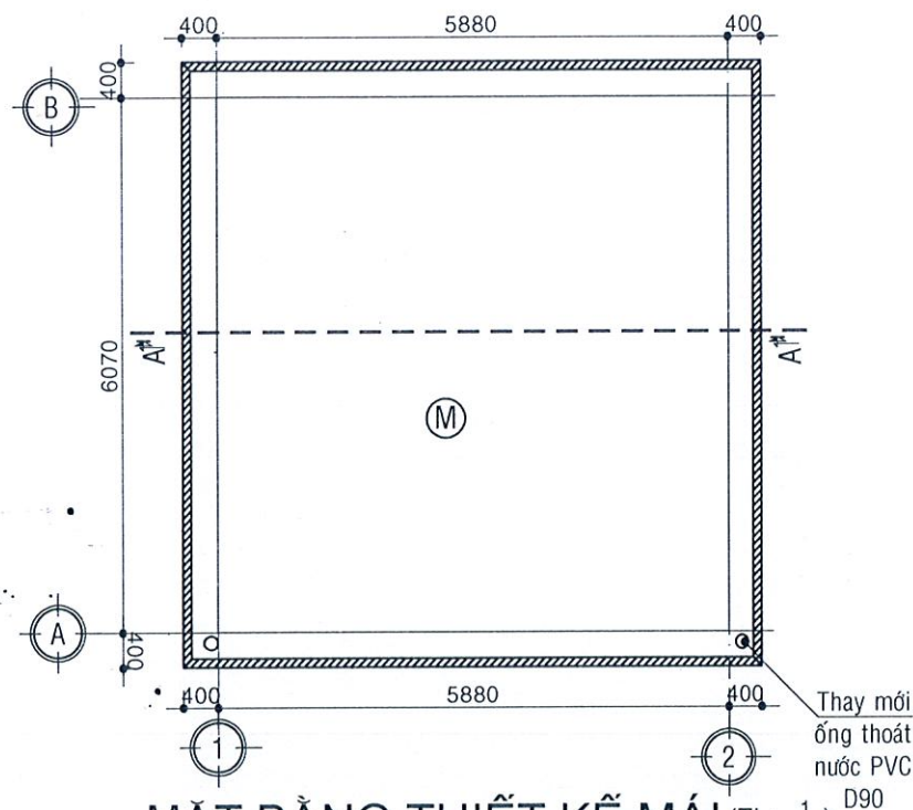
MẶT BẰNG THIẾT KẾ MÁI (TL: 1/100)
