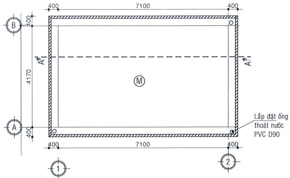
MẶT BẰNG THIẾT KẾ MÁI (TL: 1/100)
