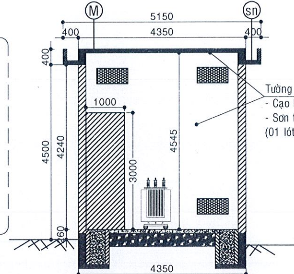
MẶT CẮT A-A (TL: 1/100)
