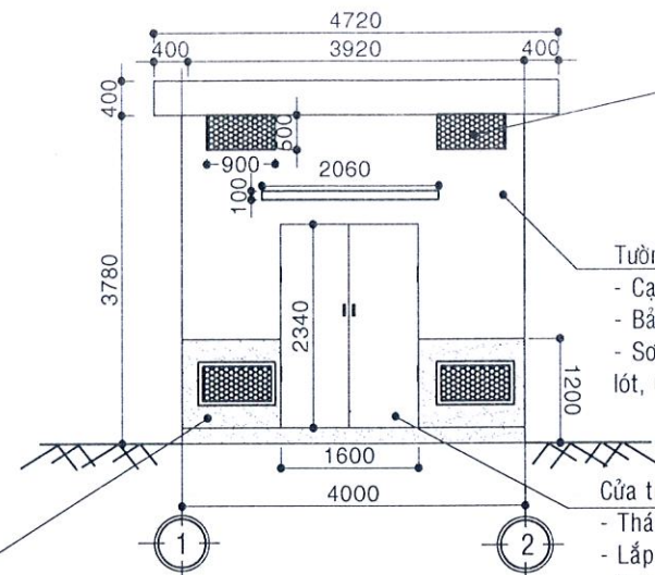
MẶT ĐỨNG THIẾT KẾ TRỤC 1-2 (TL: 1/100)
