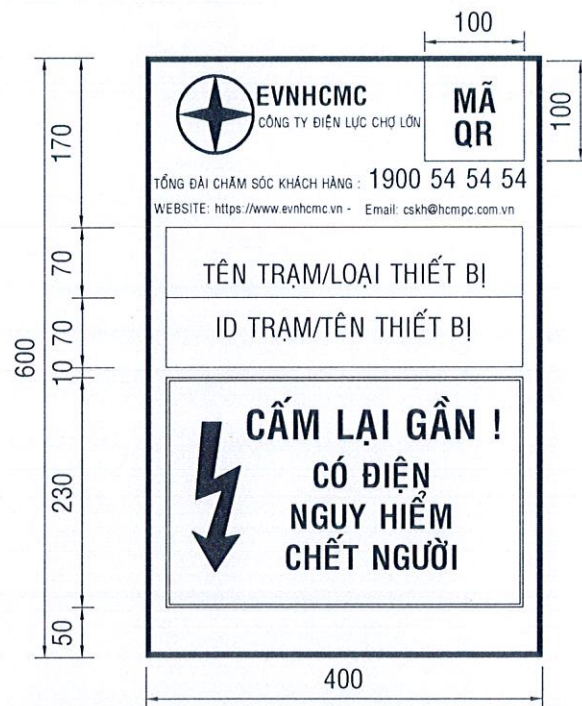
BẢNG CẢNH BÁO NGUY HIỂM - BẢNG TÊN TRẠM
