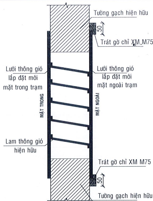
CHI TIẾT THIẾT KẾ KHOAN LẮP ĐẶT LƯỚI THÔNG GIÓ BÊN DƯỚI (MẶT NGOÀI)(TL: 1/10)
