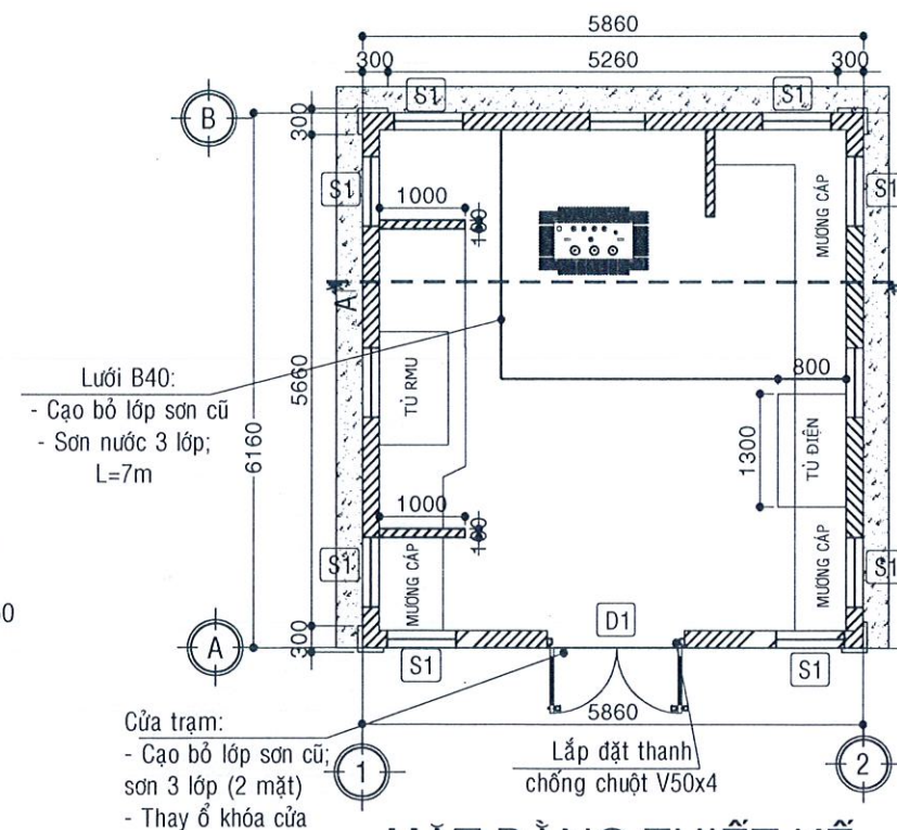
MẶT BẰNG THIẾT KẾ (TL: \frac{1}{100} )
