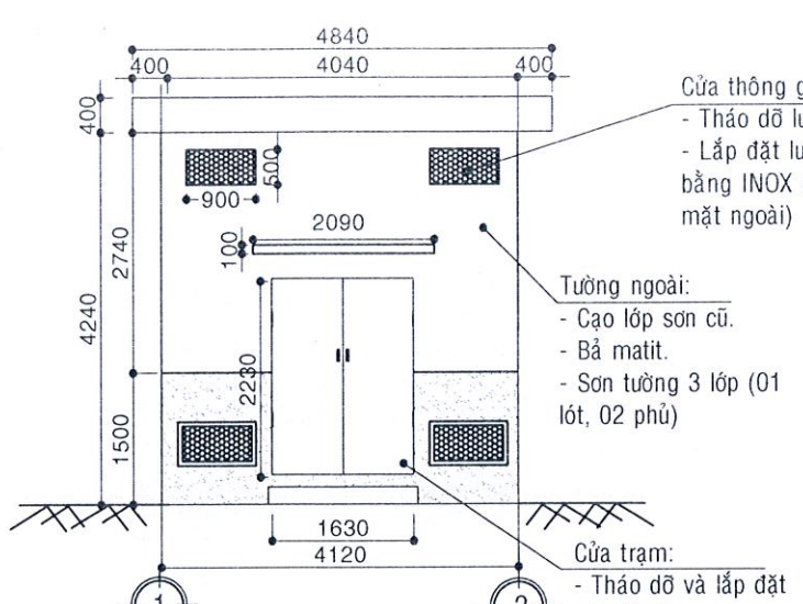
MẶT ĐỨNG THIẾT KẾ TRỤC 1-2 (TL: 1/100)
