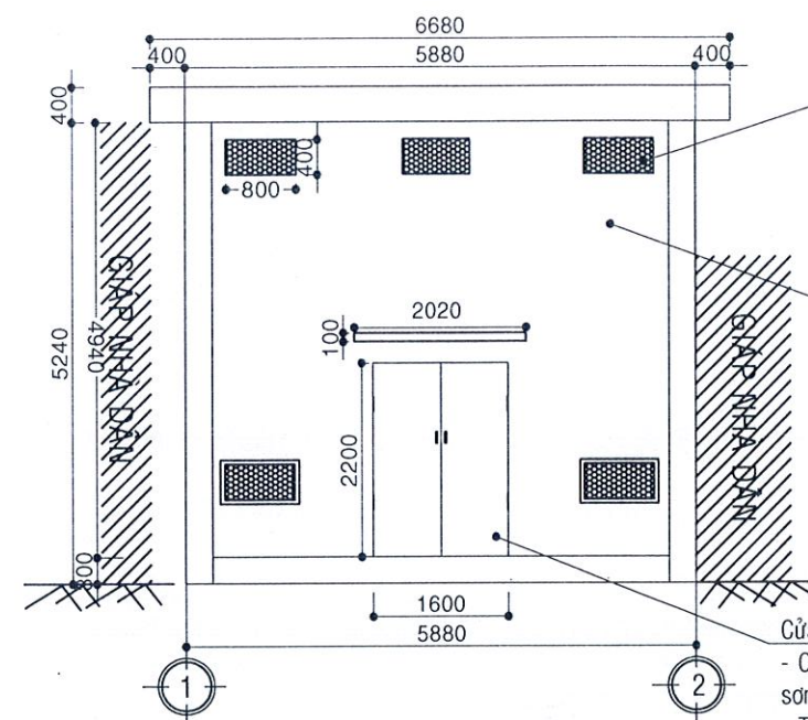
MẶT ĐỨNG THIẾT KẾ TRỤC 1-2 (TL: \frac{1}{100} )
