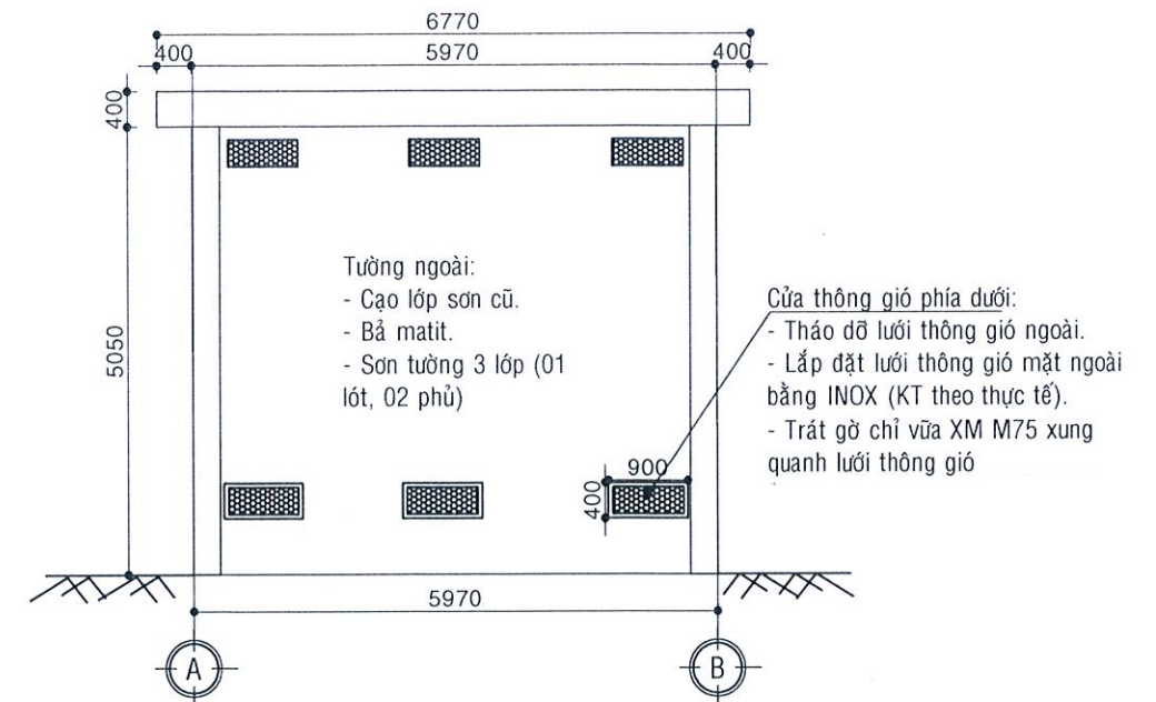
MẶT ĐƯỜNG THIẾT KẾ TRỤC A-B; B-A (TL: 1/100)
