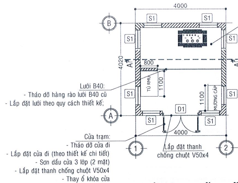
MẶT BẰNG THIẾT KẾ (TL: 1/100)
