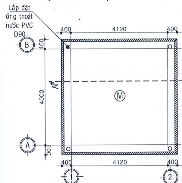
MẶT BẰNG THIẾT KẾ MÁI (TL: 1/100)
