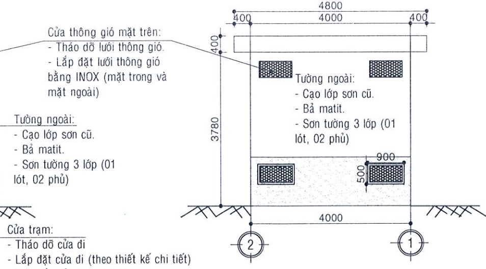
MẶT ĐỨNG THIẾT KẾ TRỤC 2-1 (TL: 1/100)
