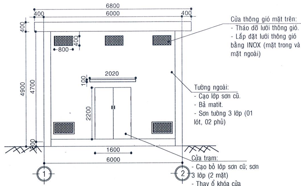
MẶT ĐỨNG THIẾT KẾ TRỤC 1-2 (TL: \frac{1}{100} )
