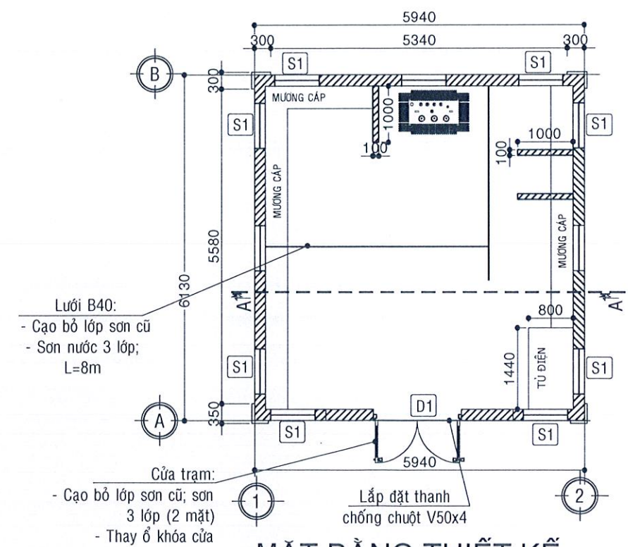
MẶT BẰNG THIẾT KẾ (TL: \frac{1}{100} )
