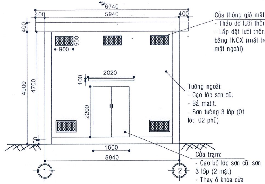
MẶT ĐỨNG THIẾT KẾ TRỤC 1-2 (TL: \frac{1}{100} )
