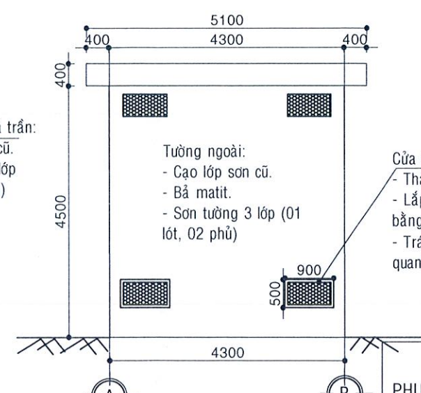
MẶT ĐỨNG THIẾT KẾ TRỤC A-B;B-A (TL: 1/100)
