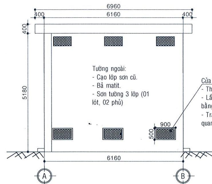
MẶT ĐƯỜNG THIẾT KẾ TRỤC A-B; B-A (TL: 1/100)
