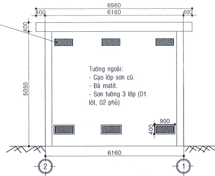
MẶT ĐỨNG THIẾT KẾ TRỤC 2-1 (TL: \frac{1}{100} )
