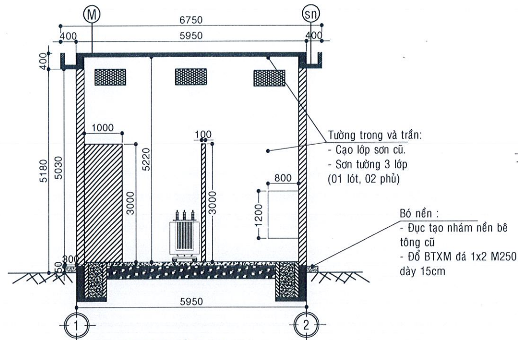
MẶT CẮT A-A (TL: \frac{1}{100} )
