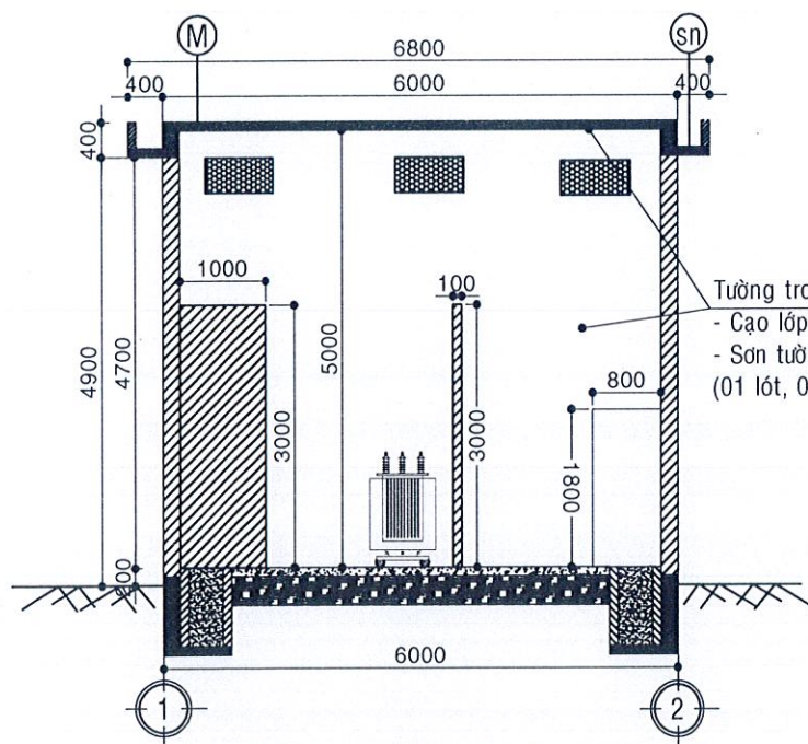
MẶT CẮT A-A (TL: \frac{1}{100} )
