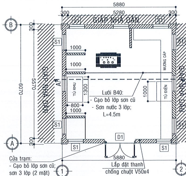
MẶT BẰNG THIẾT KẾ (TL: \frac{1}{100} )
