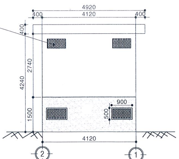
MẶT ĐỨNG THIẾT KẾ TRỤC 2-1 (TL: 1/100)
