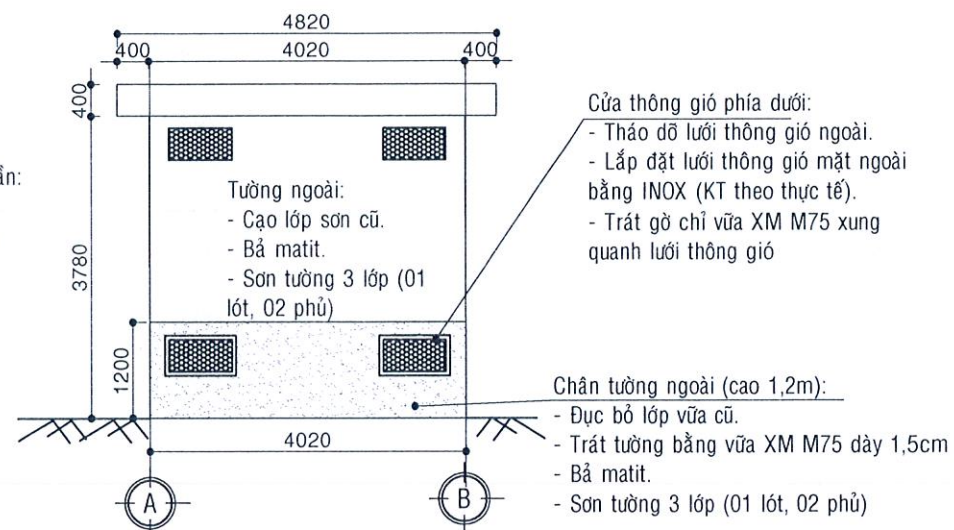
MẶT ĐỨNG THIẾT KẾ TRỤC A-B; B-A (TL: 1/100)
