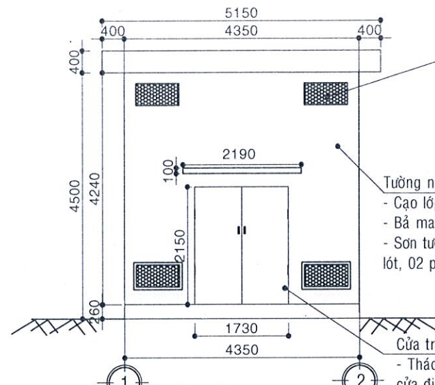
MẶT ĐỨNG THIẾT KẾ TRỤC 1-2 (TL: 1/100)
