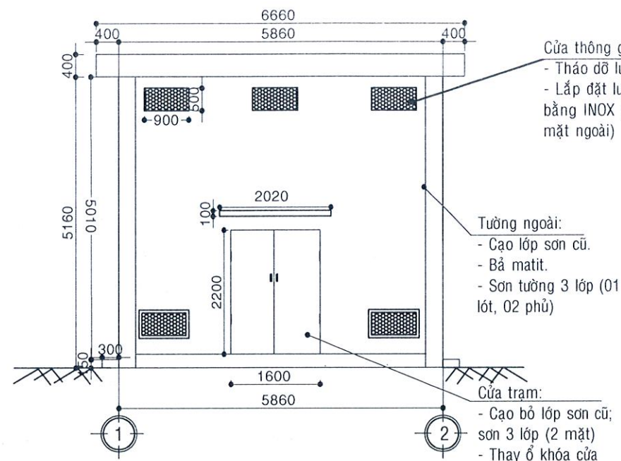
MẶT ĐỨNG THIẾT KẾ TRỤC 1-2 (TL: \frac{1}{100} )
