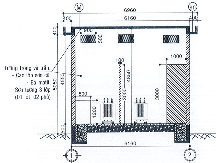
MẶT CẮT A-A (TL: \frac{1}{100} )
