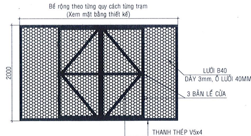
CHI TIẾT THIẾT KẾ KHUNG LƯỚI B40 (TL: 1/50)
