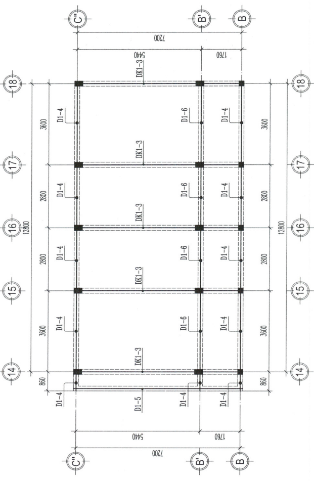
MẶT BẰNG KẾT CẤU CỐT ±0.000 < TL: 1/100 >
