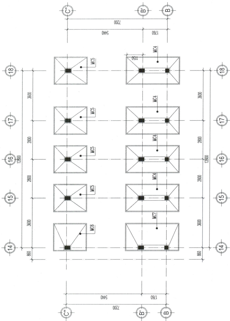
MẶT BẰNG KẾT CẤU MÓNG TRỤC 14-18 <TL: 1/100>
