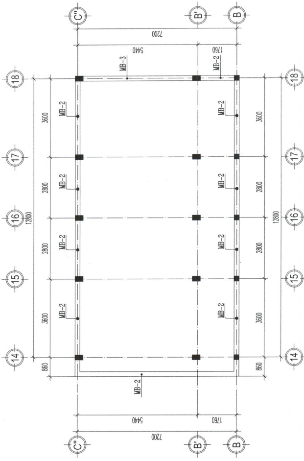
MẶT BẰNG BỐ TRÍ MÓNG BỐ <TL: 1/100>
