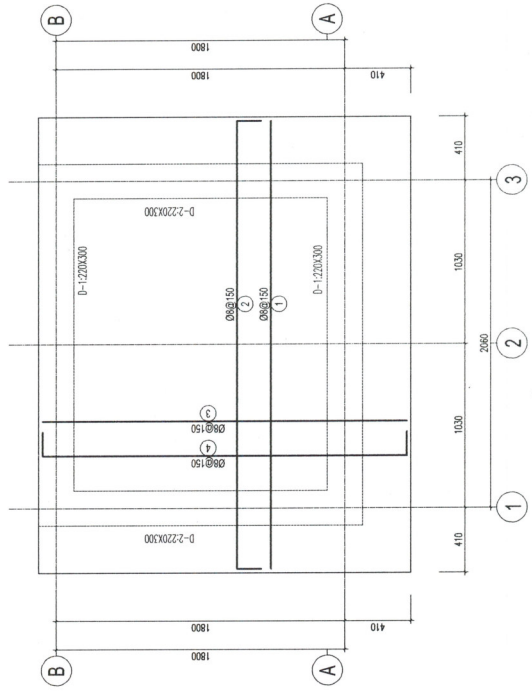
MẶT BẰNG BỐ TRÍ THÉP MÁI
