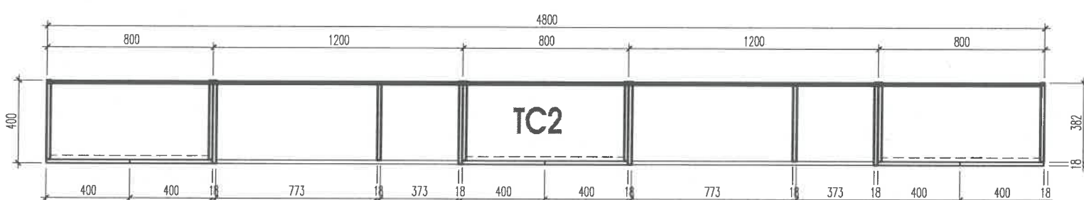
MẶT CẮT 2-2
