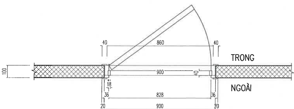
MẶT BẰNG
