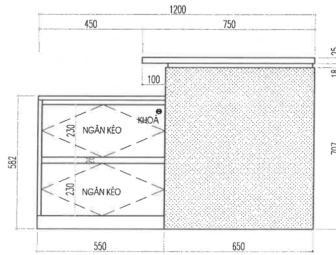
MẶT BÊN 1
