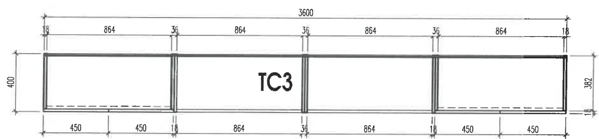
MẶT CẮT 2-2
