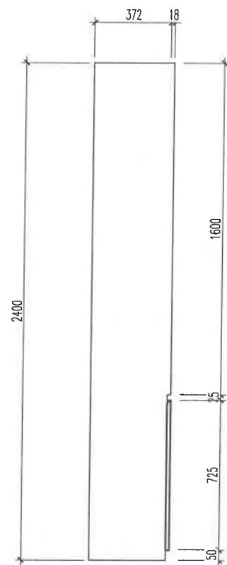
MẶT BÊN HỆ TỦ 1200
