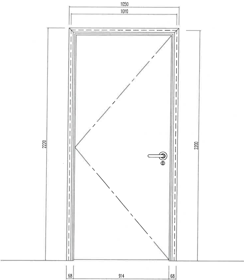
MẶT ĐÚNG NGOÀI
