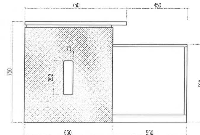
MẶT BÊN 2
