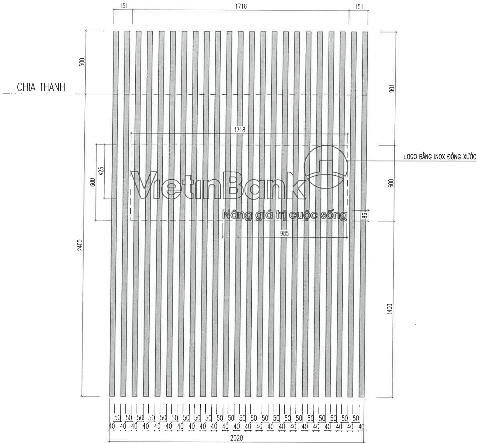
MẶT ĐỨNG
