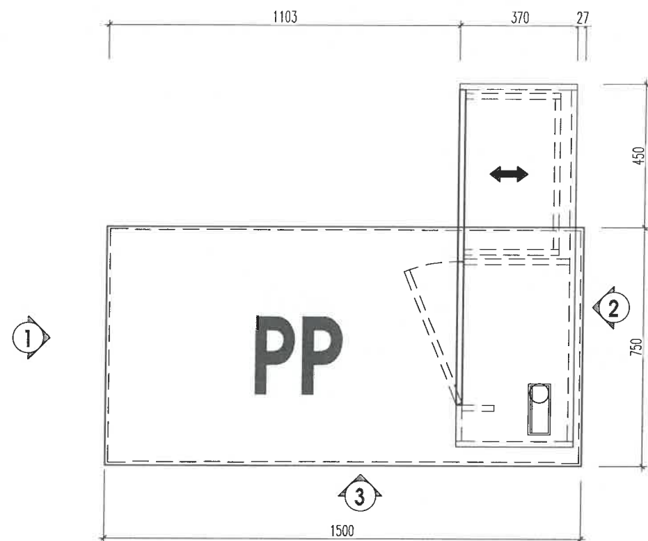
MẶT BẰNG
