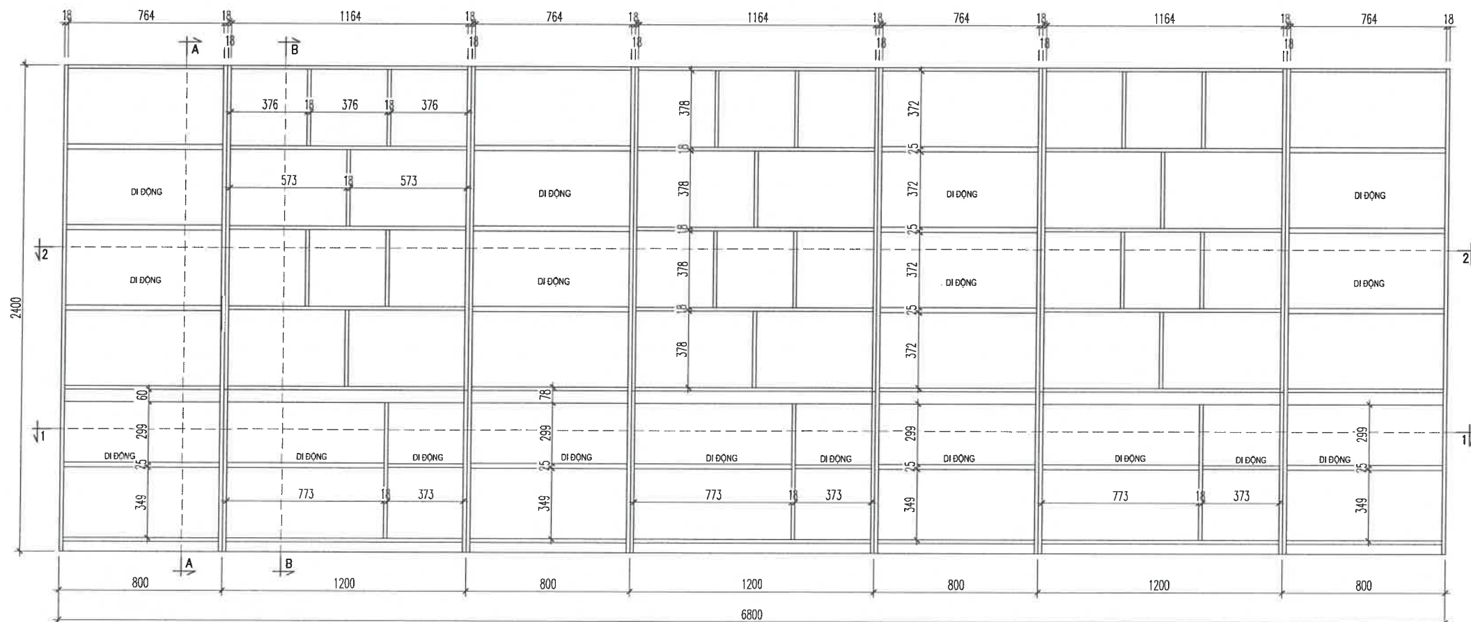
MẶT ĐỨNG BỎ CÁNH
