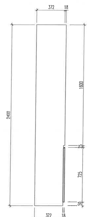
MẶT BÊN HỆ TỦ 1200
