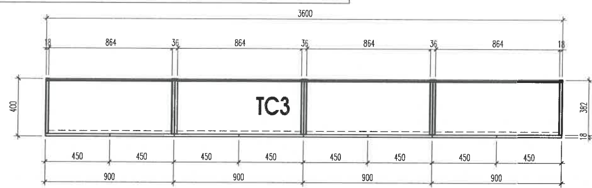
MẶT CẮT 1-1
