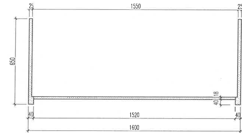
MẶT CẮT 1-1
