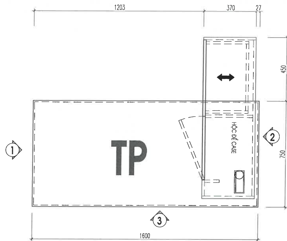
MẶT BẰNG
