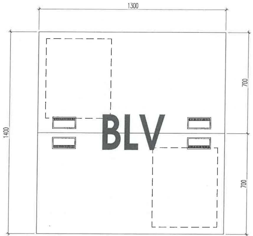
MẶT BẰNG
