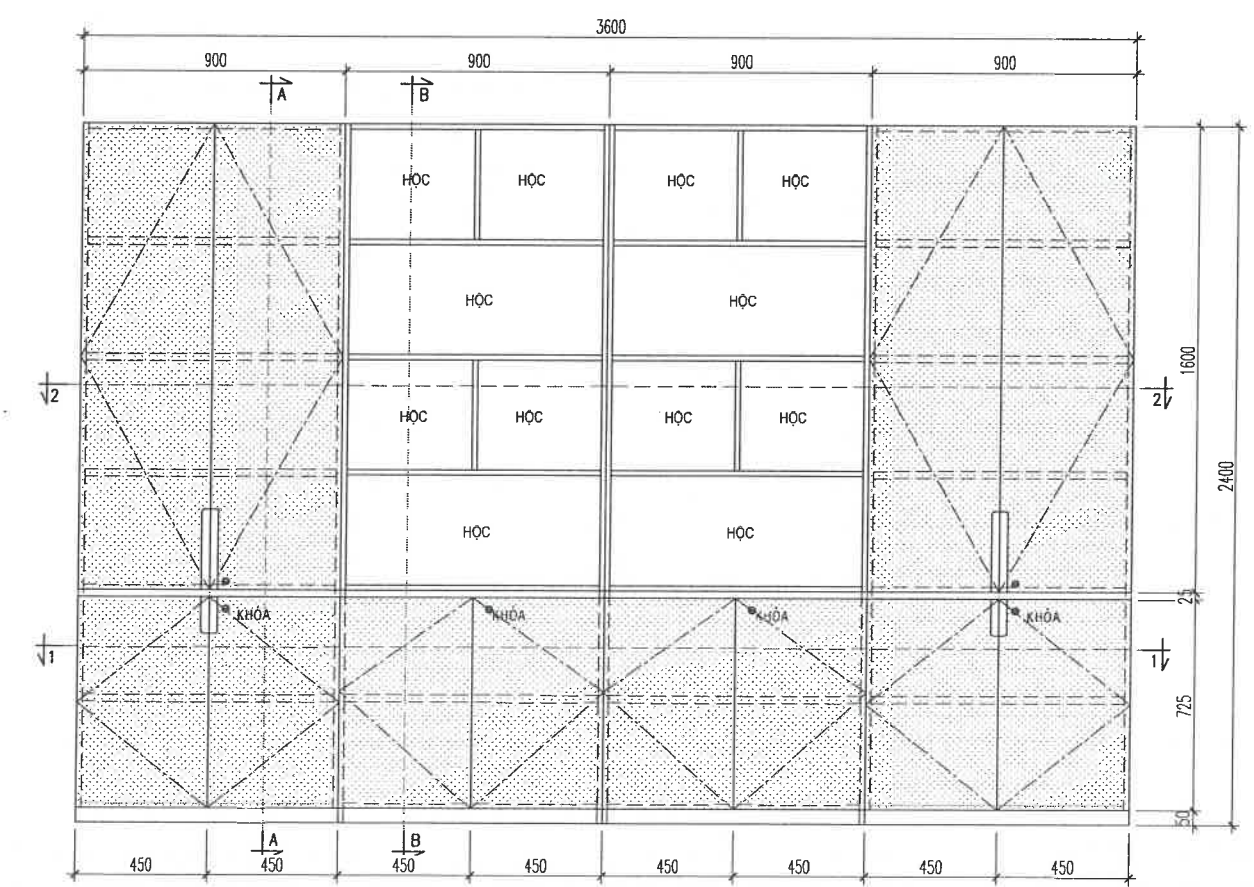
MẶT ĐƯNG TỦ TC3
