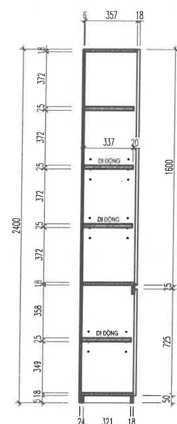
MẶT CẮT A-A
