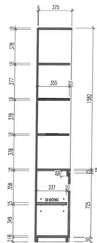
MẶT CẮT B-B
