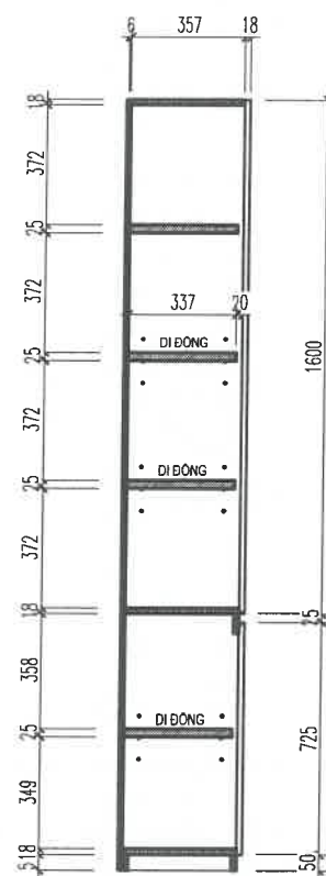
MẶT CẮT A-A
