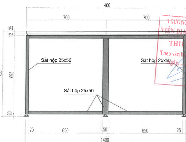
MẶT BÊN
