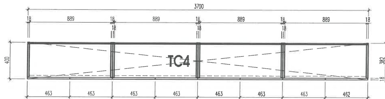
MẶT CẮT 1-1
