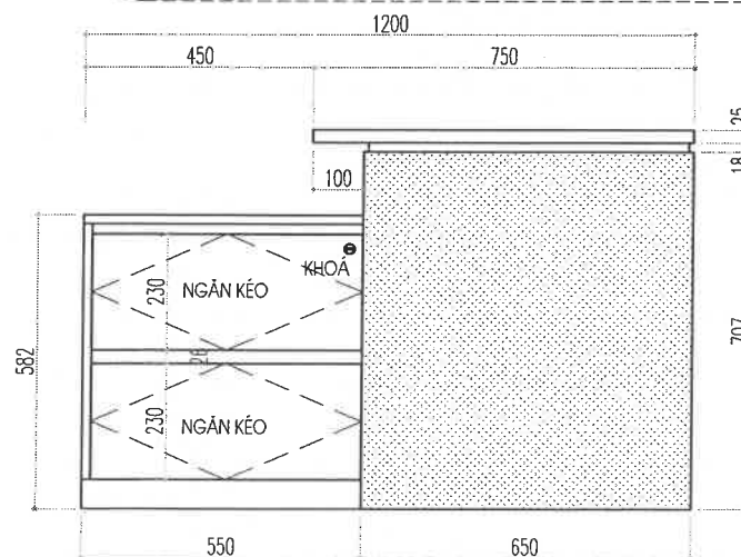
MẶT BÊN 1
