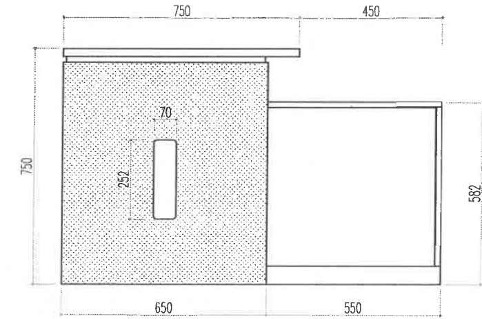
MẶT BÊN 2
