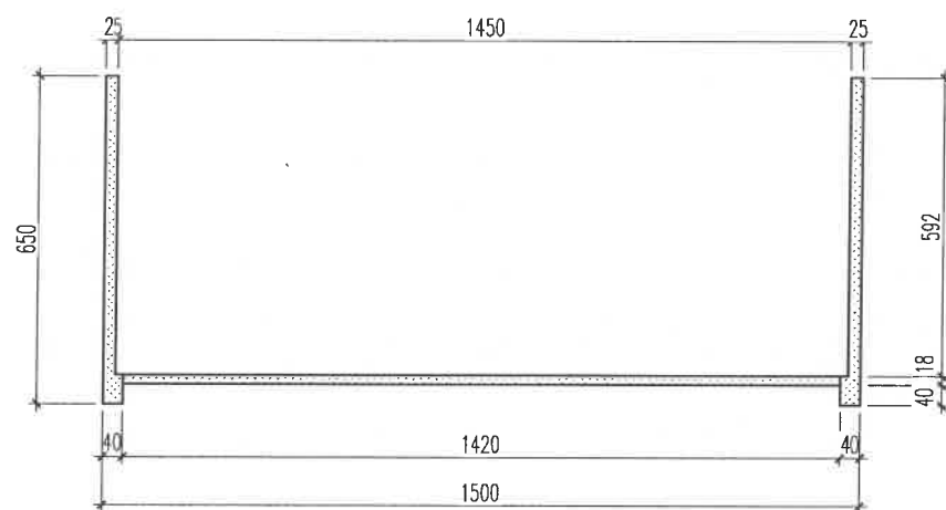
MẶT CẮT 1-1
