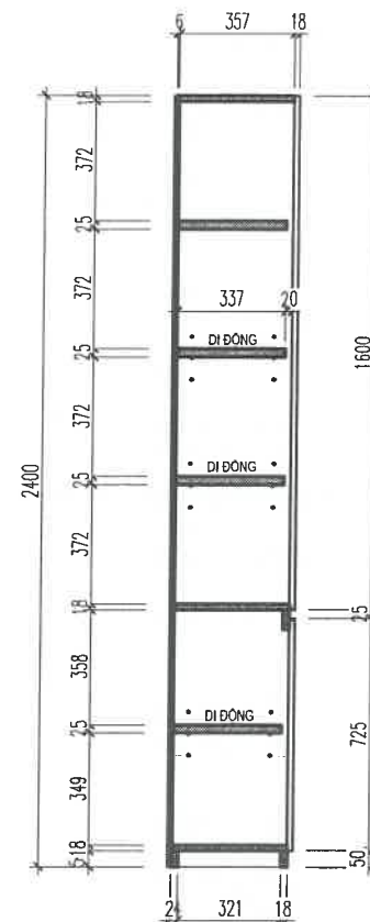
MẶT CẮT A-A
