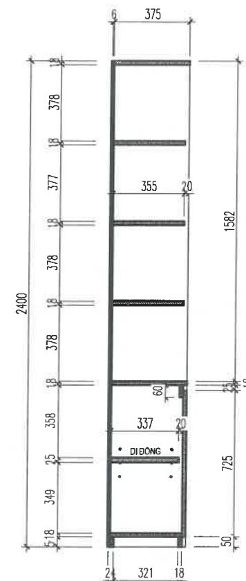
MẶT CẮT B-B
