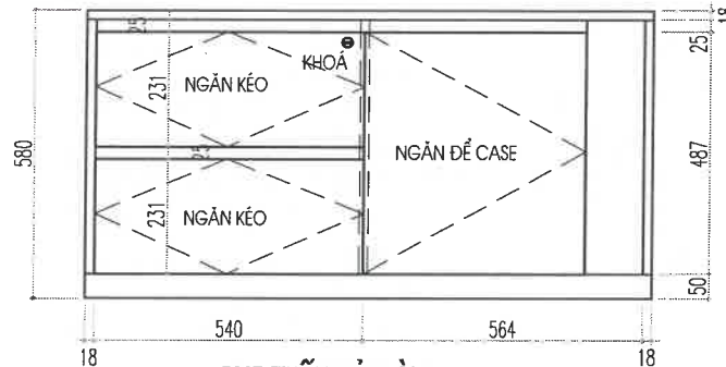
CHI TIẾT TỦ RỜI
