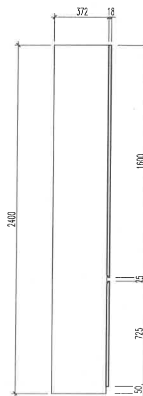
MẶT BÊN HỆ TỦ KÍN
