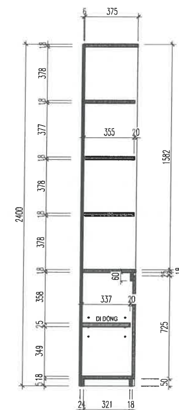
MẶT CẮT B-B
