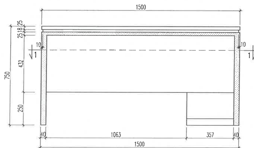
MẶT ĐỨNG 3
