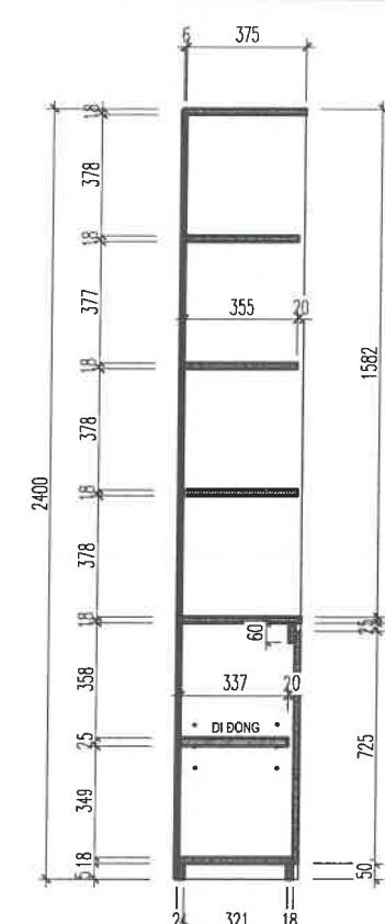
MẶT CẮT B-B
