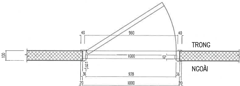
MẶT BẰNG
