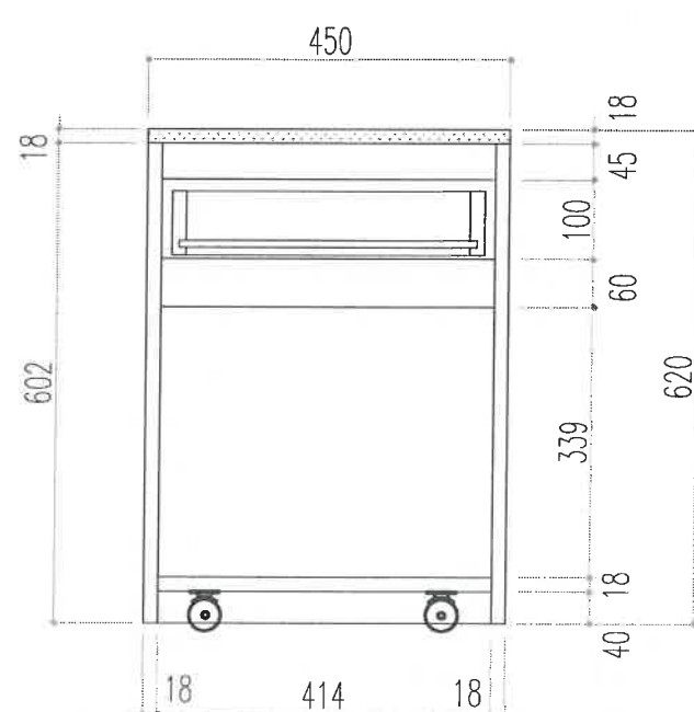
MẶT ĐỨNG BỎ CÁCH
