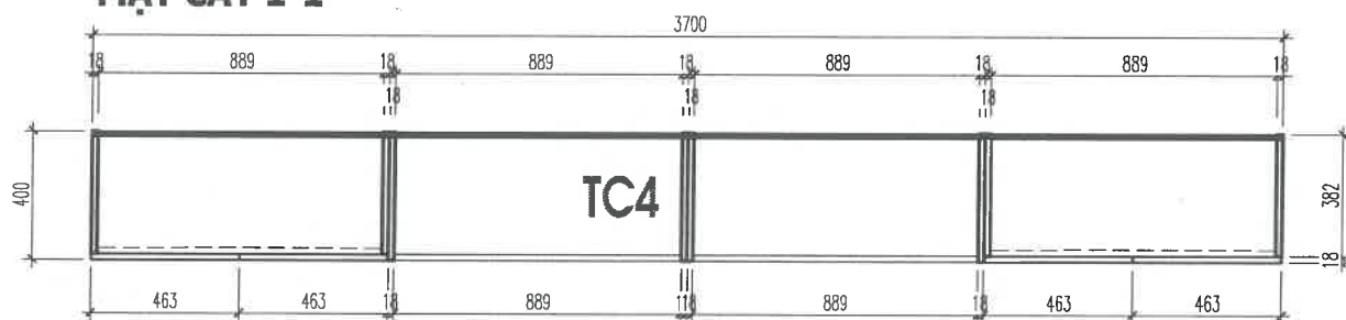
MẶT CẮT 2-2
