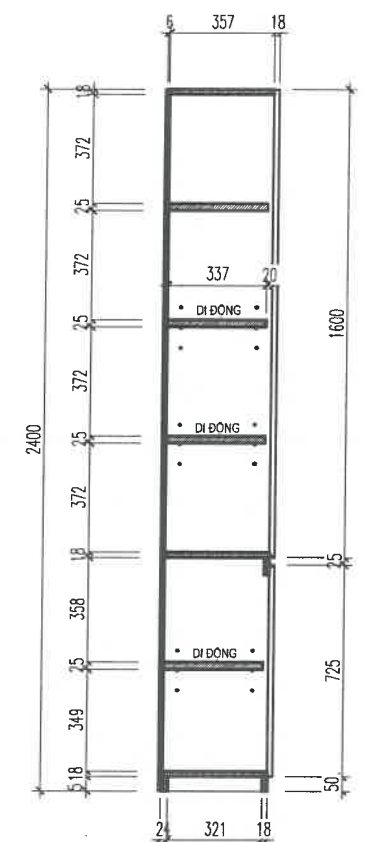
MẶT CẮT A-A
