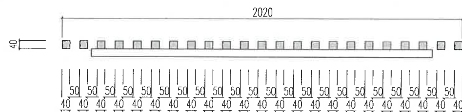
MẶT BẰNG
