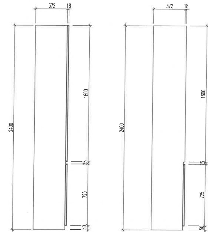
MẶT BÊN HỆ TỦ 800
