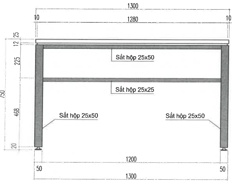
MẶT ĐỨNG
