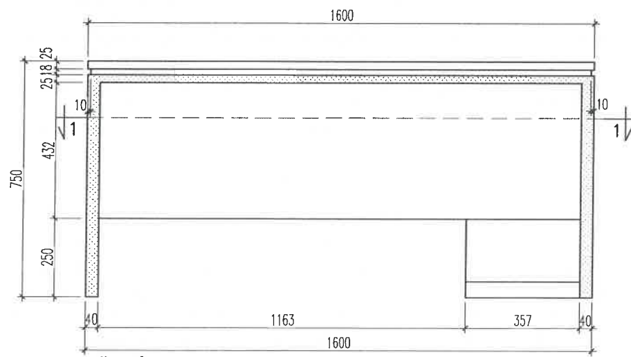
MẶT ĐÚNG 3
