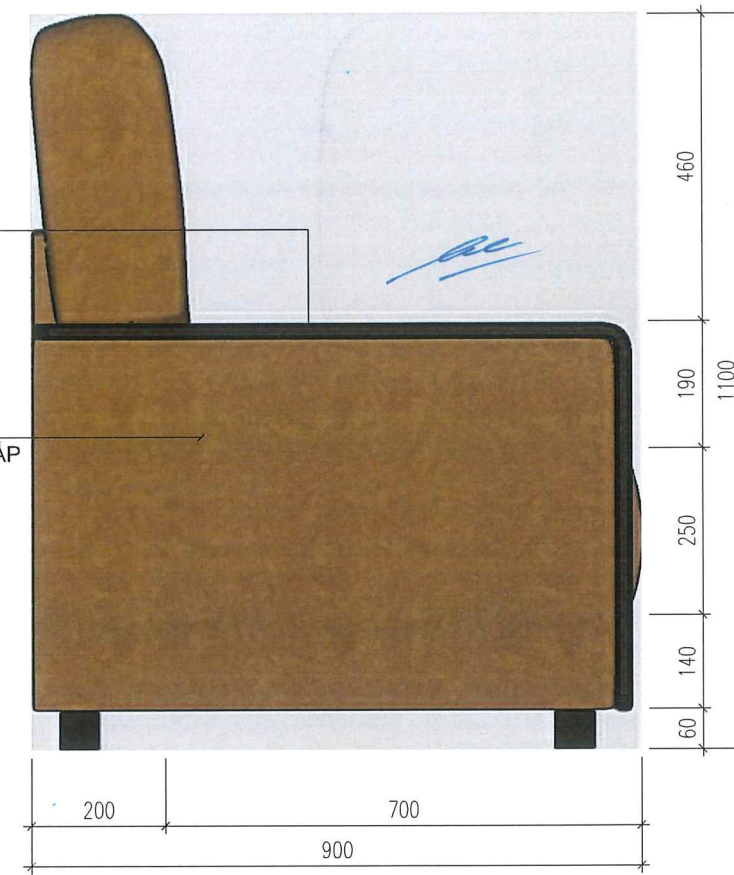
MẶT BÊN
