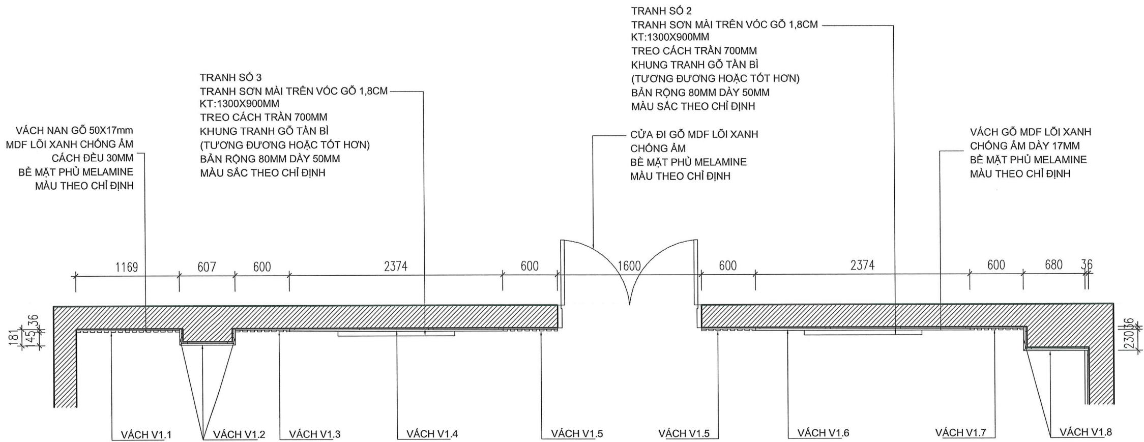
MẶT BẰNG CHI TIẾT DIỆN TƯỜNG-V1
