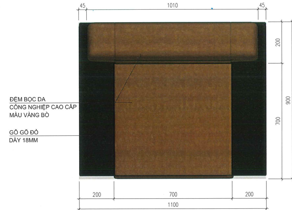
MẶT BẰNG
