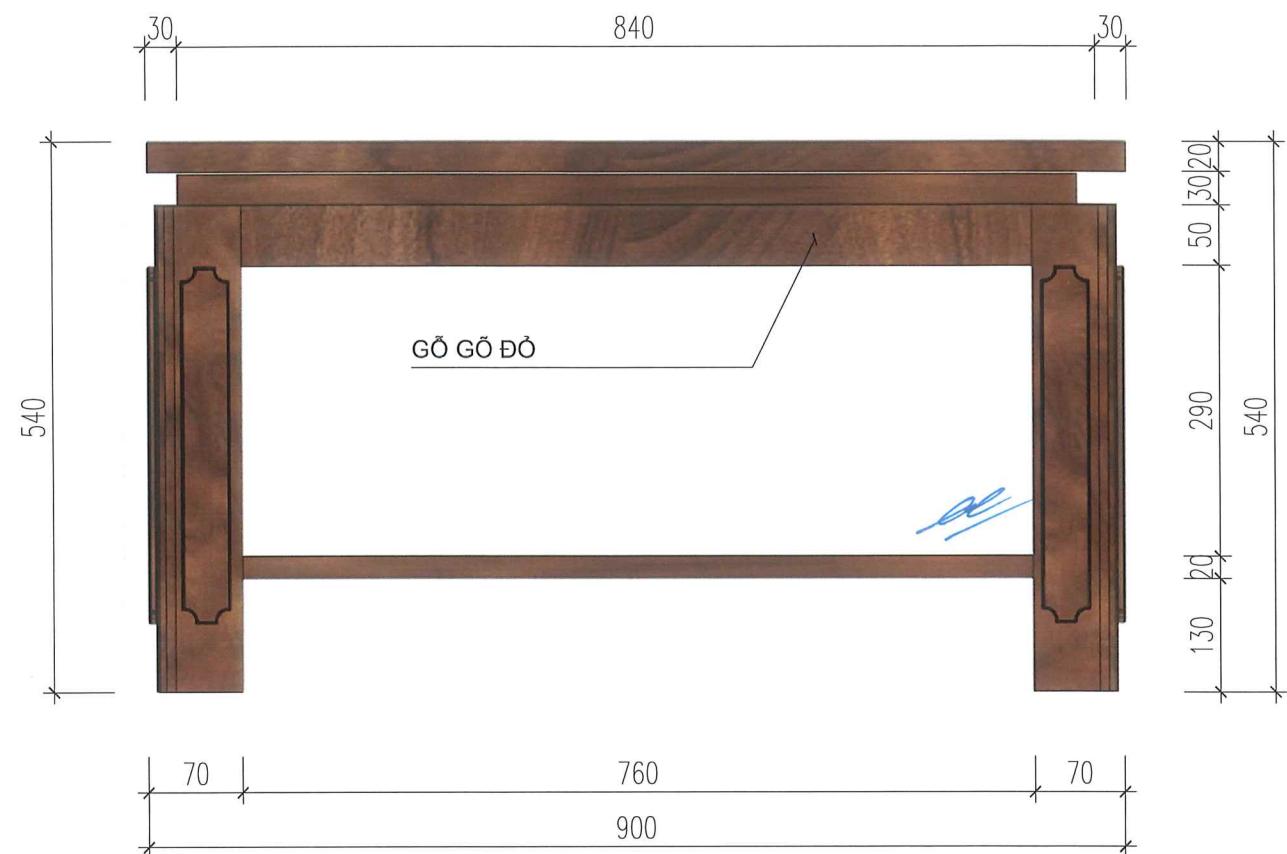
MẶT ĐỨNG
