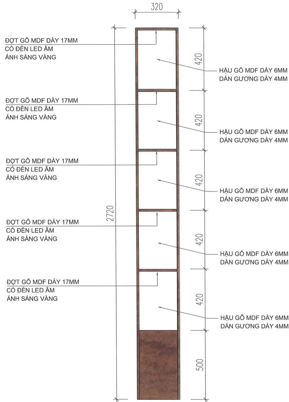
MẶT ĐỨNG
