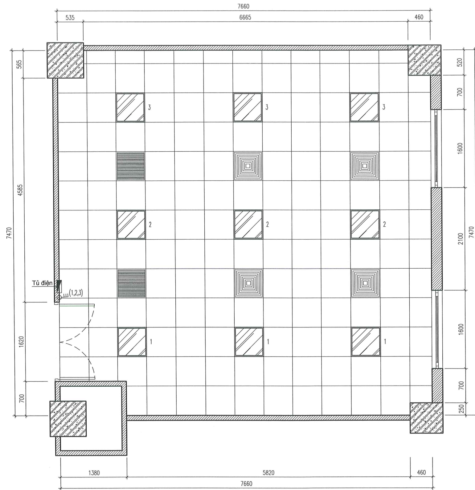
MẶT BẰNG CẤP ĐIỆN CHIẾU SÁNG HIỆN TRẠNG
