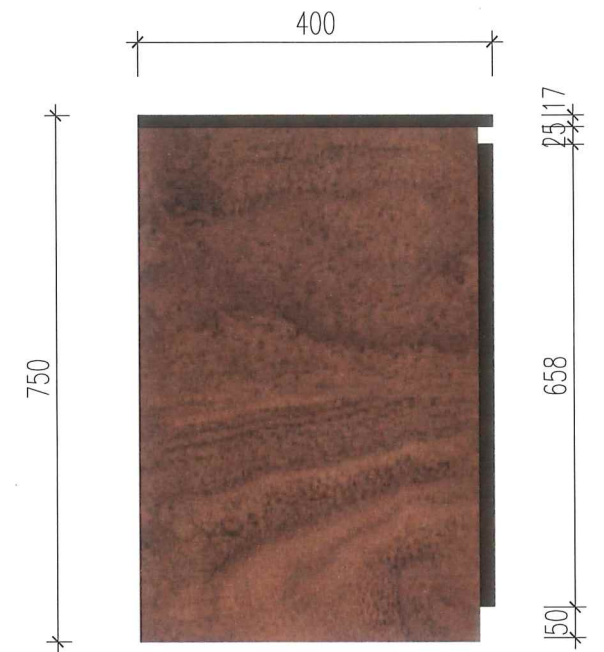
MẶT BÊN
