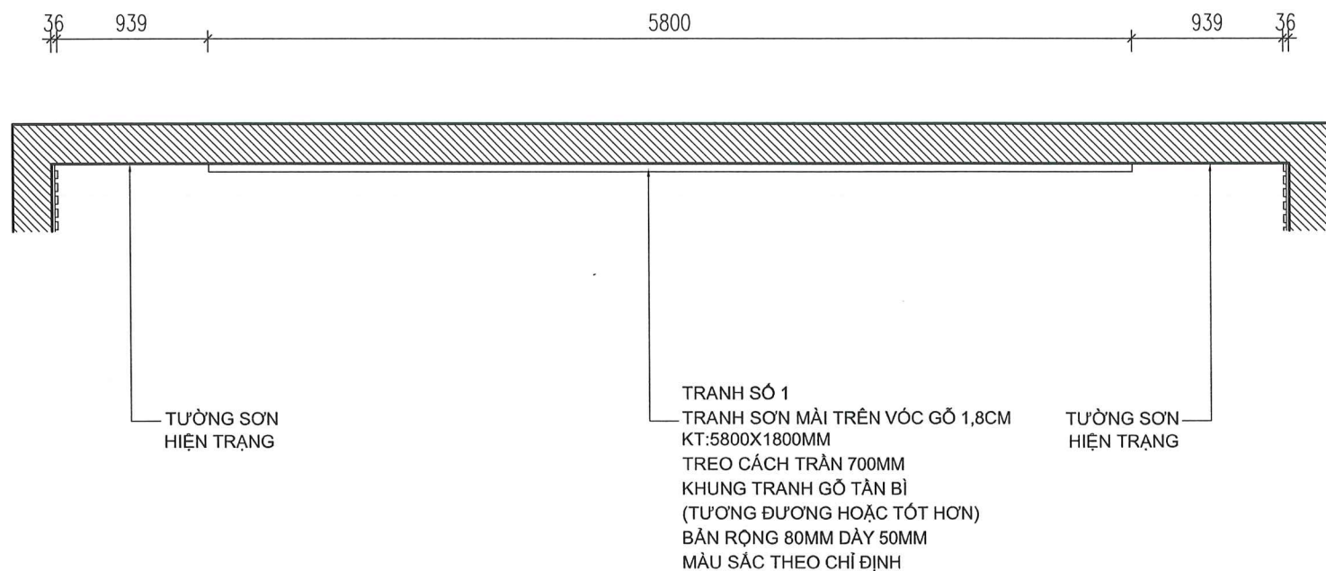
MẶT BẰNG CHI TIẾT DIỆN TƯỜNG-V4
