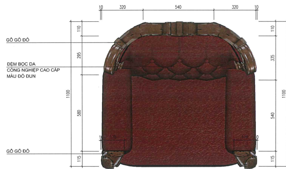
MẶT BẰNG
