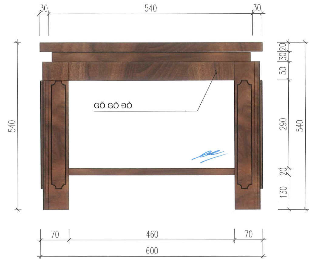
MẶT BÊN
