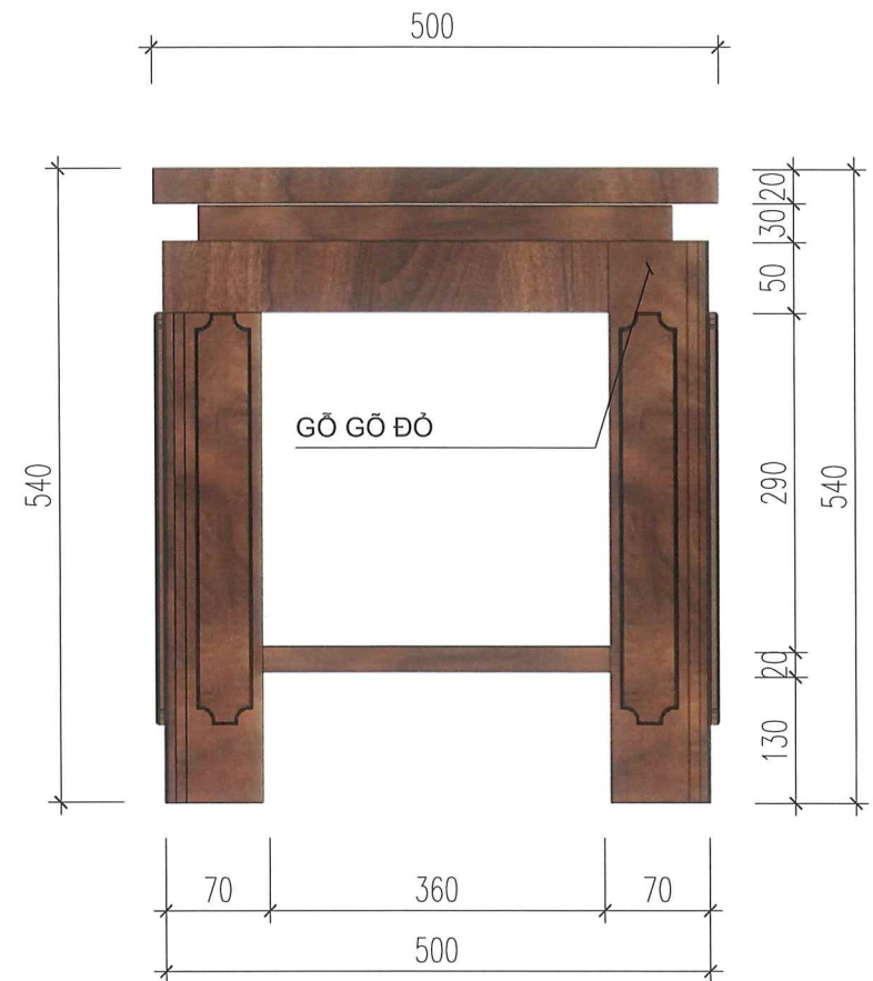
MẶT ĐỨNG
