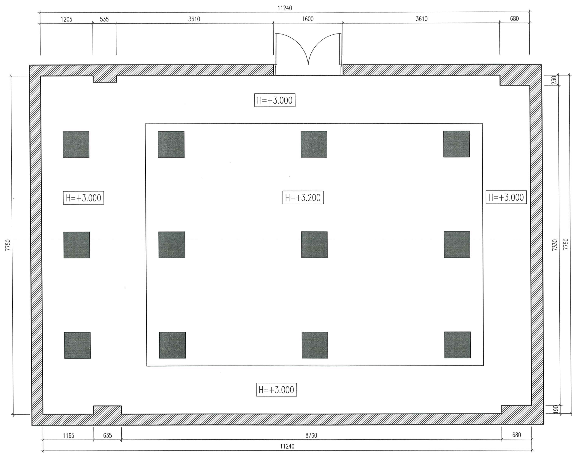
MẶT BẰNG CẢI TẠO TRẦN
