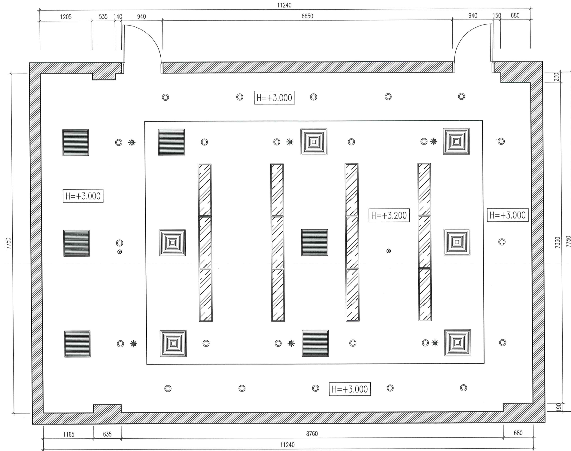
MẶT BẰNG BỐ TRÍ MIỆNG ĐIỀU HÒA HIỆN TRẠNG
