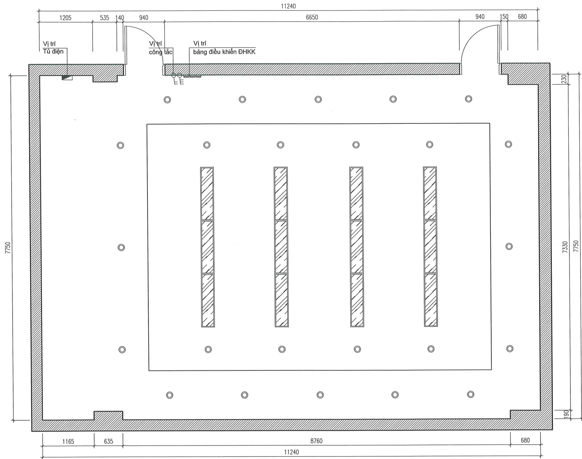
MẶT BẰNG CẤP ĐIỆN CHIẾU SÁNG HIỆN TRẠNG
