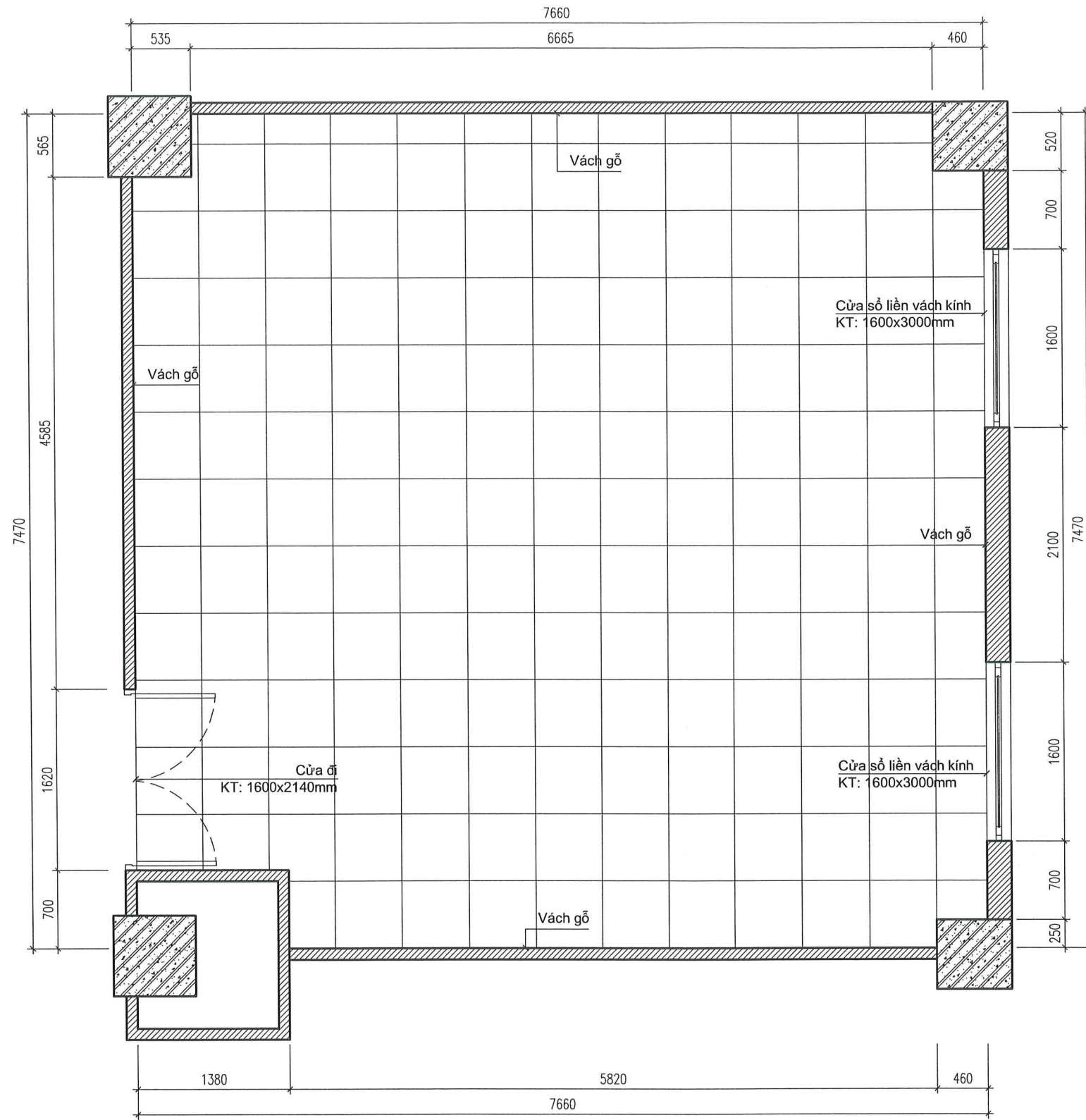
MẶT BẰNG HIỆN TRẠNG
