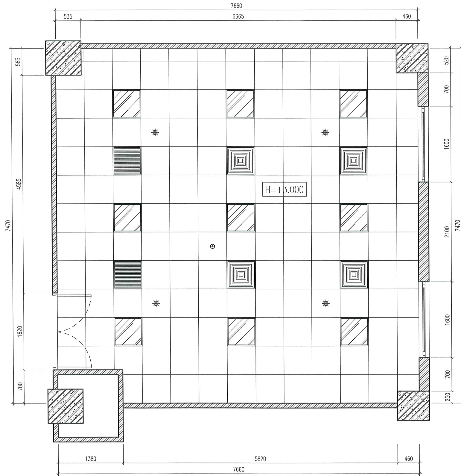
MẶT BẰNG TRẦN HIỆN TRẠNG
