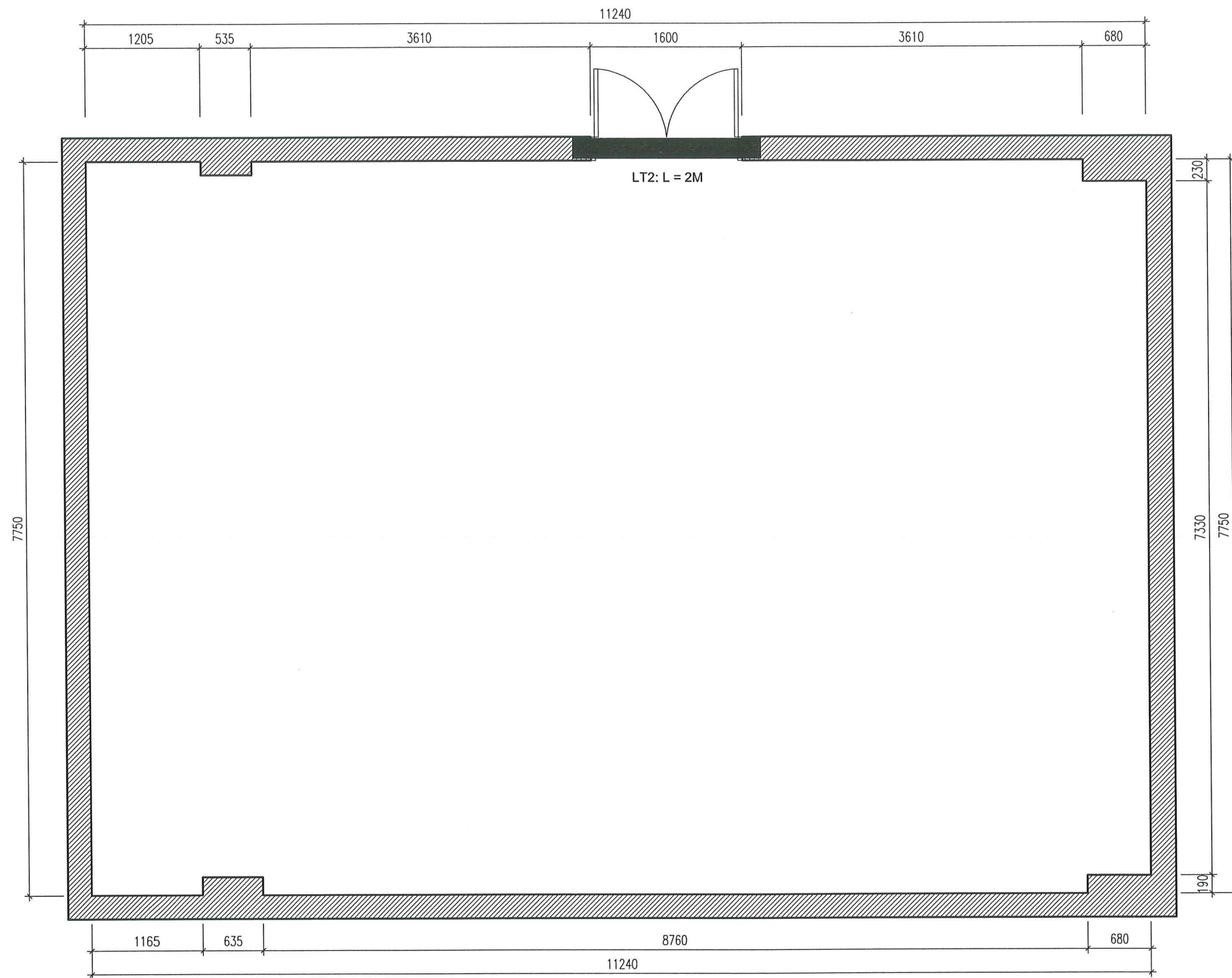
MẶT BẰNG LANH TÔ CỬA
