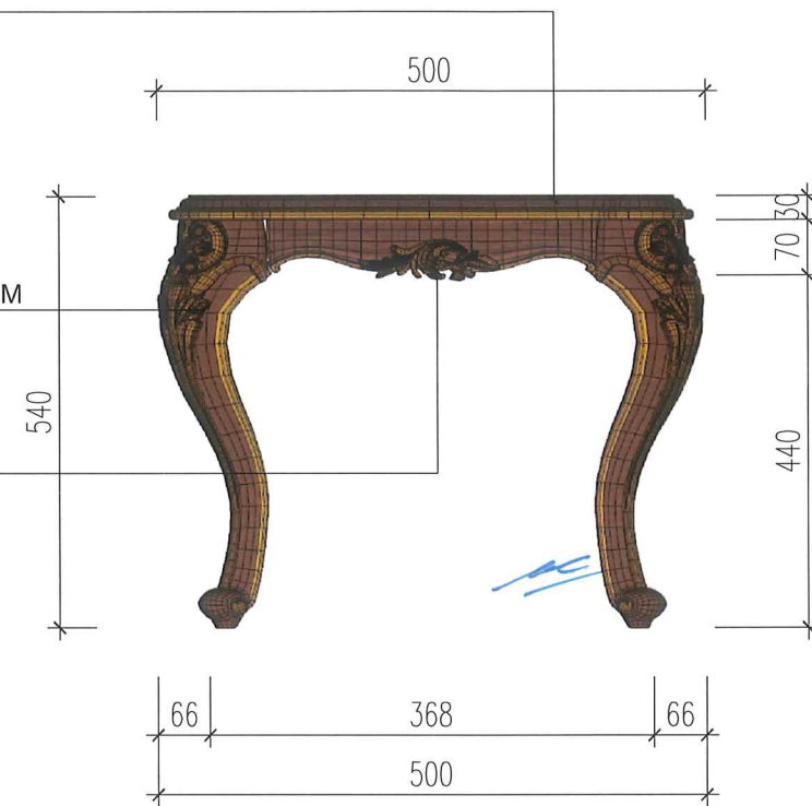
MẶT BÊN
