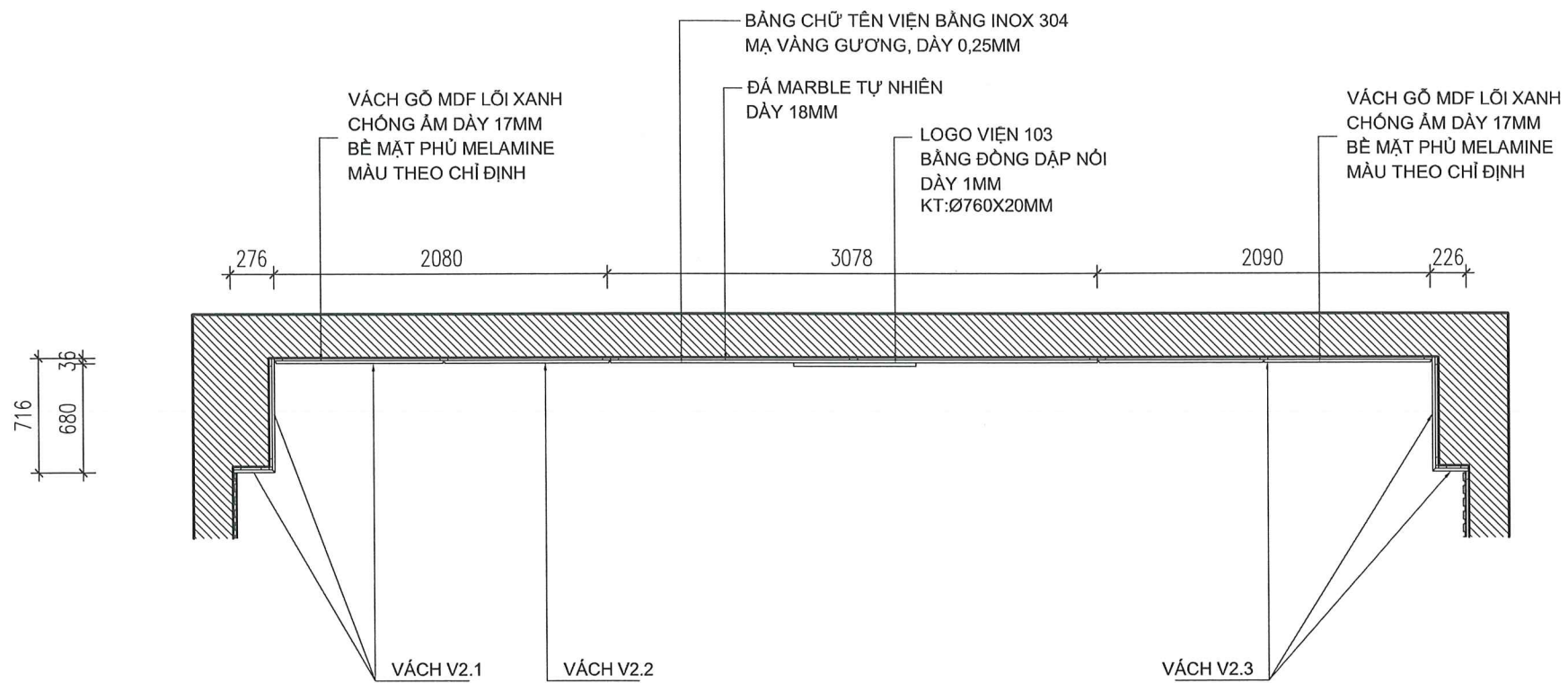
MẶT BẰNG CHI TIẾT DIỆN TƯỜNG-V2
