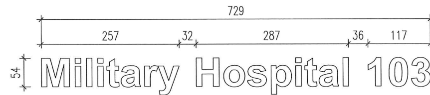
CHI TIẾT 5
