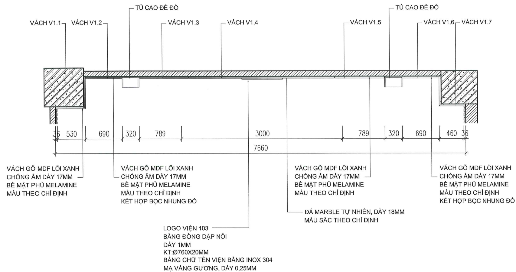
MẶT BẰNG ĐIỆN TƯỜNG-V1
