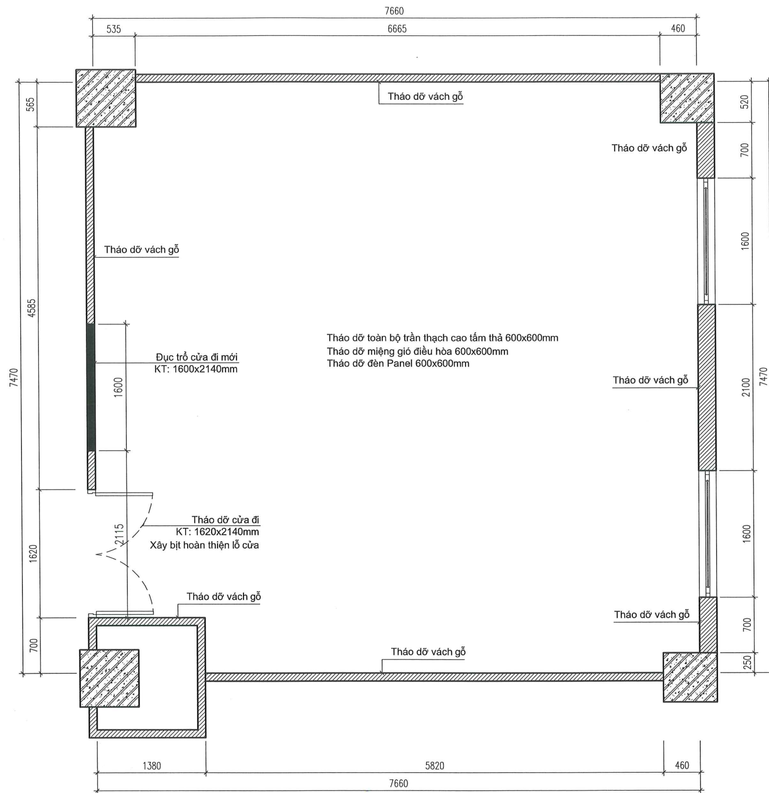
MẶT BẰNG PHÁ DỠ
