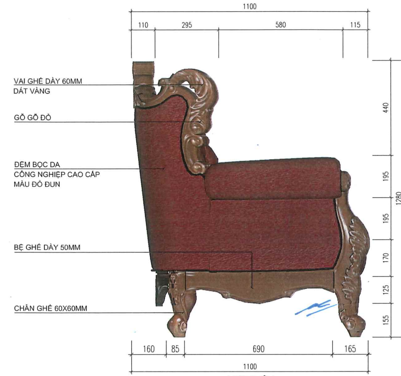
MẶT BÊN
