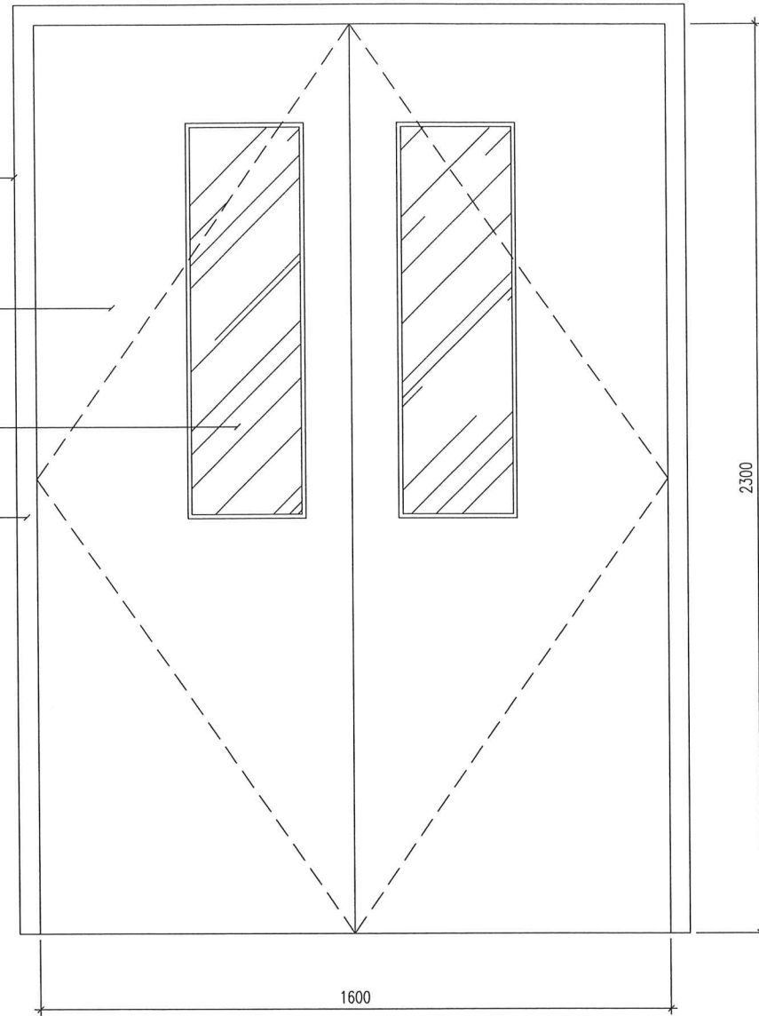
MẶT ĐỨNG
