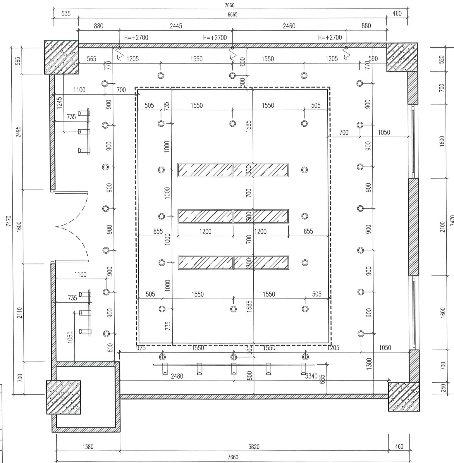
MẶT BẰNG ĐỊNH VỊ ĐÈN CHIẾU SÁNG CẢI TẠO
