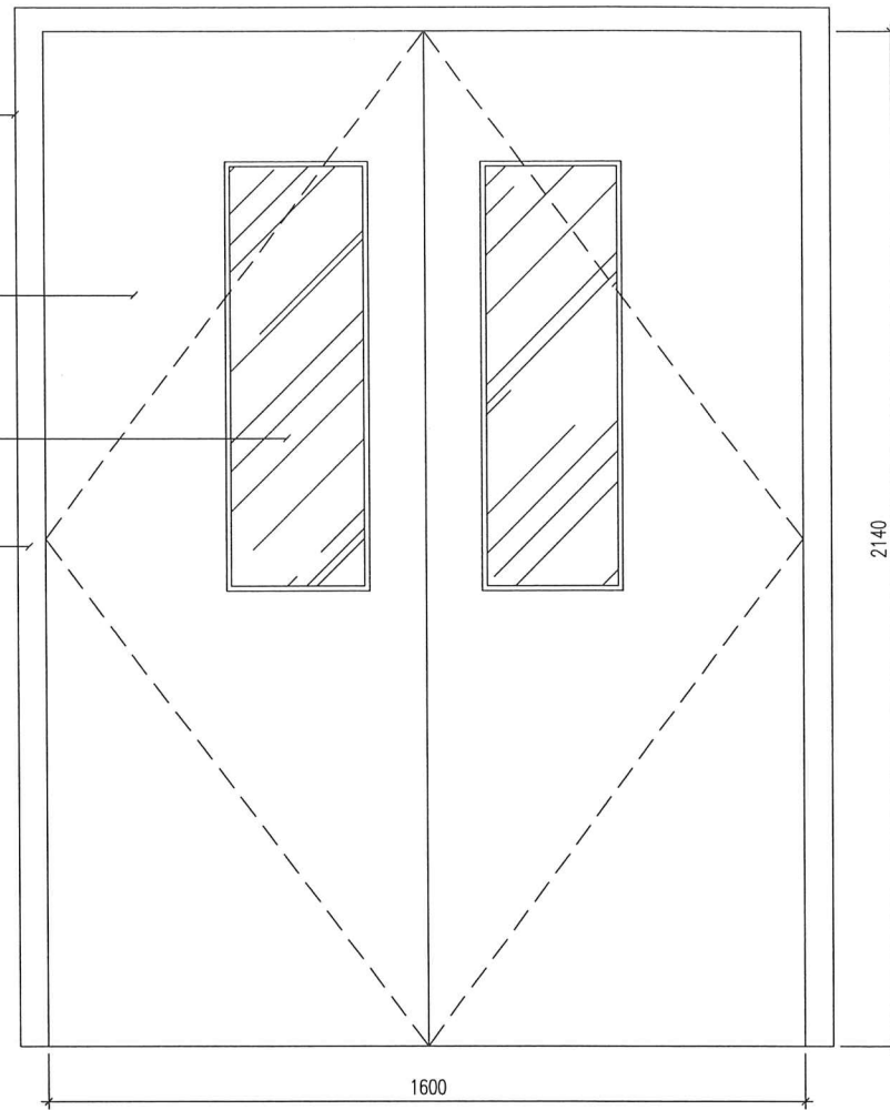
MẶT ĐỨNG
