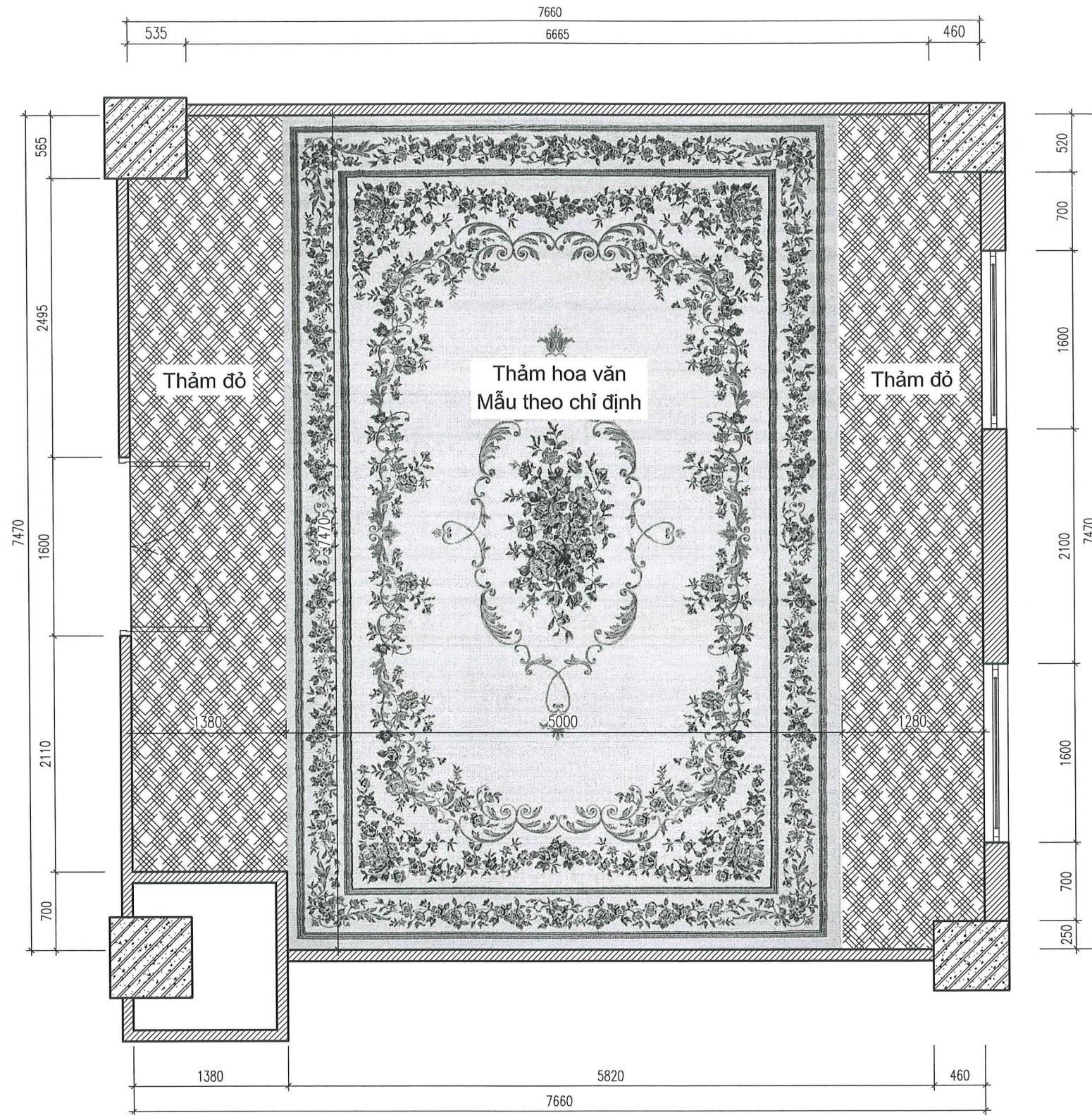
MẶT BẰNG CẢI TẠO SÀN
