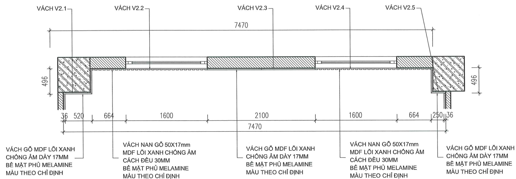
MẶT BẰNG DIỆN TƯỜNG-V2
