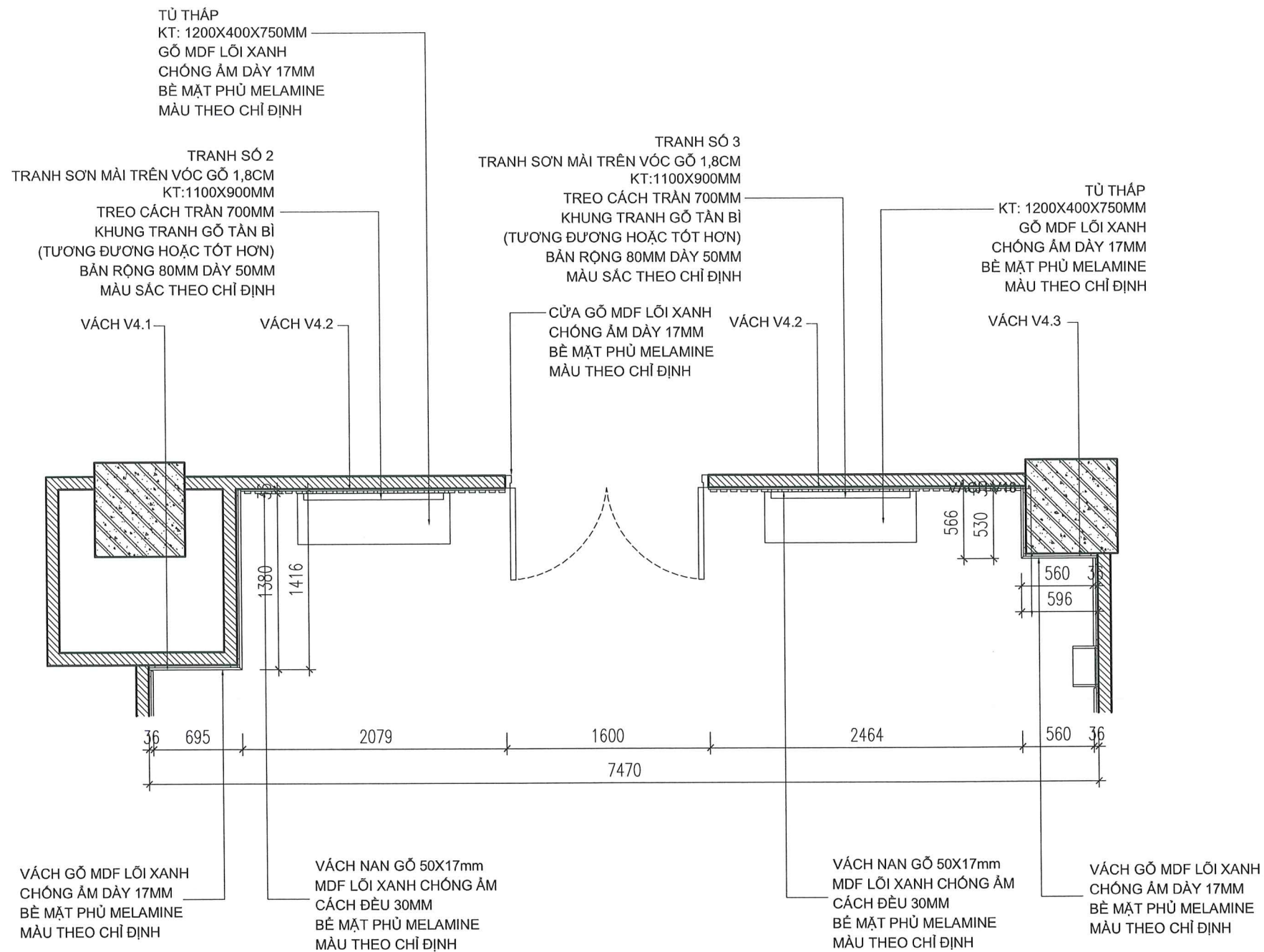
MẶT BẰNG DIỆN TƯỜNG-V4
