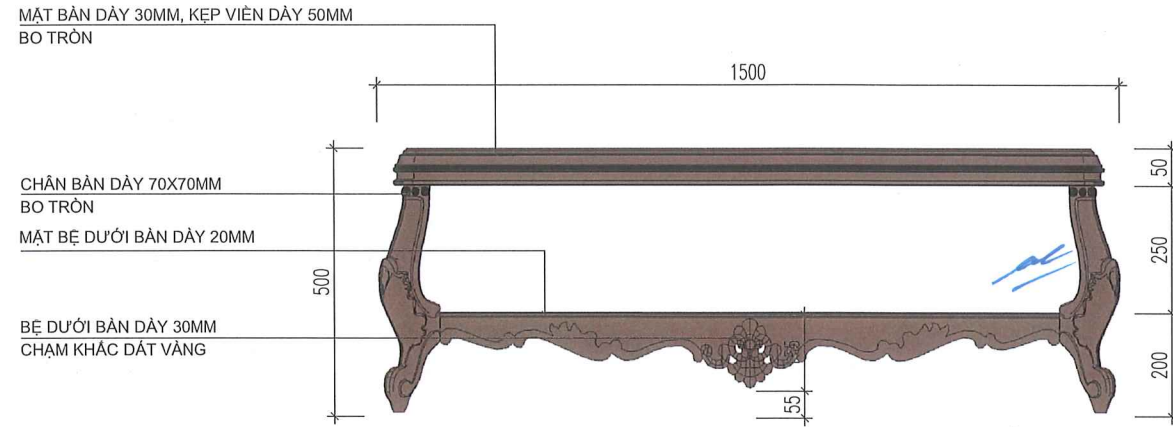
MẶT ĐỨNG
