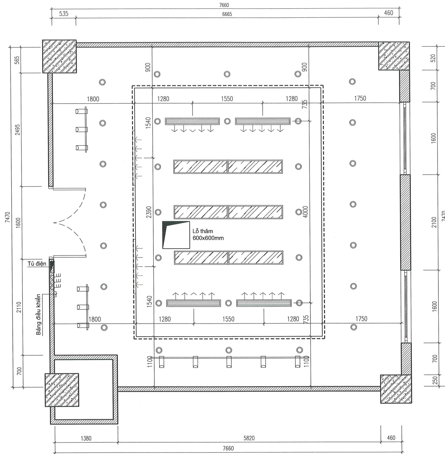
MẶT BẰNG BỐ TRÍ MIỆNG ĐIỀU HÒA CẢI TẠO
