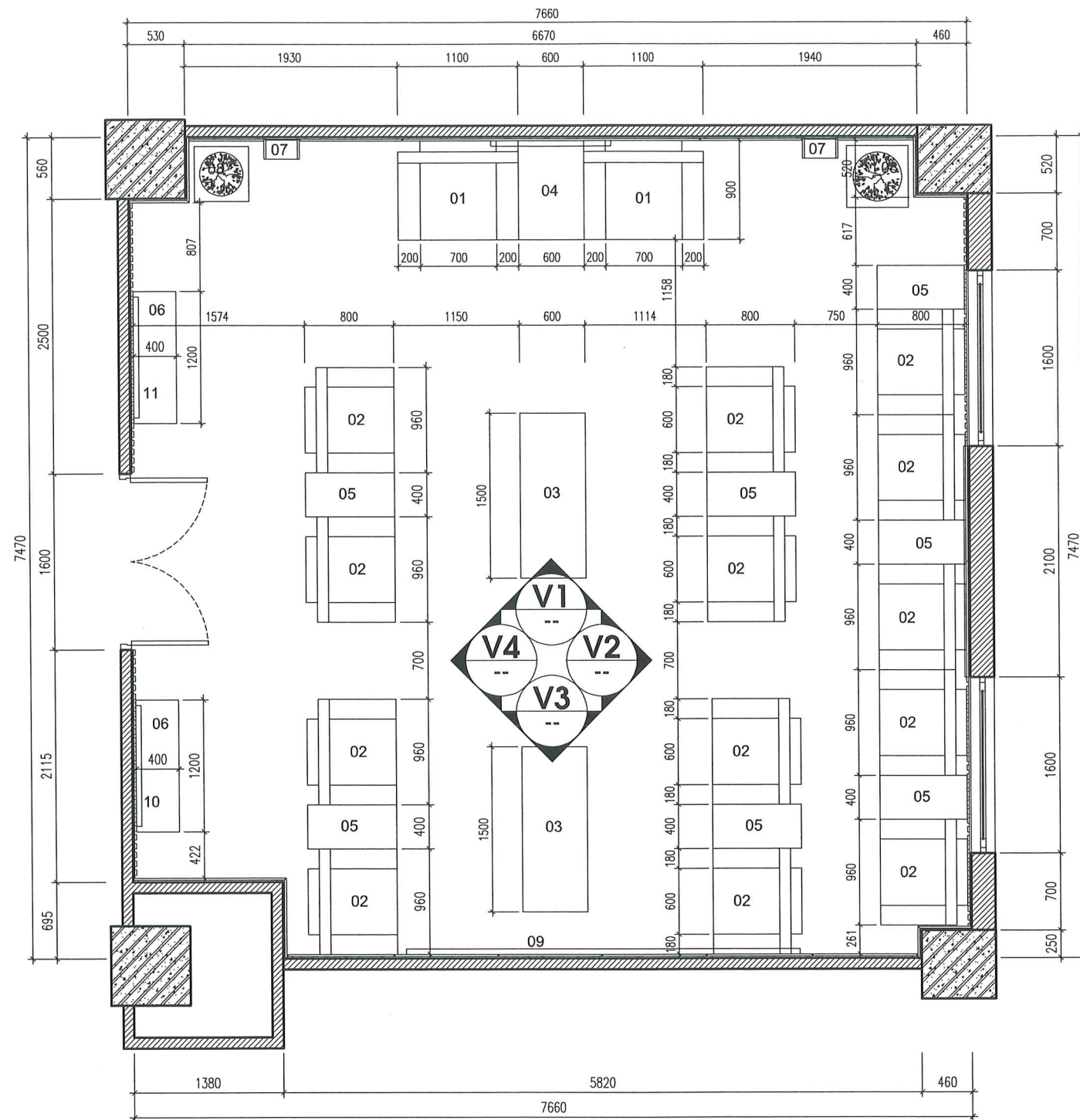
MẶT BẰNG ĐỊNH VỊ NỘI THẤT
