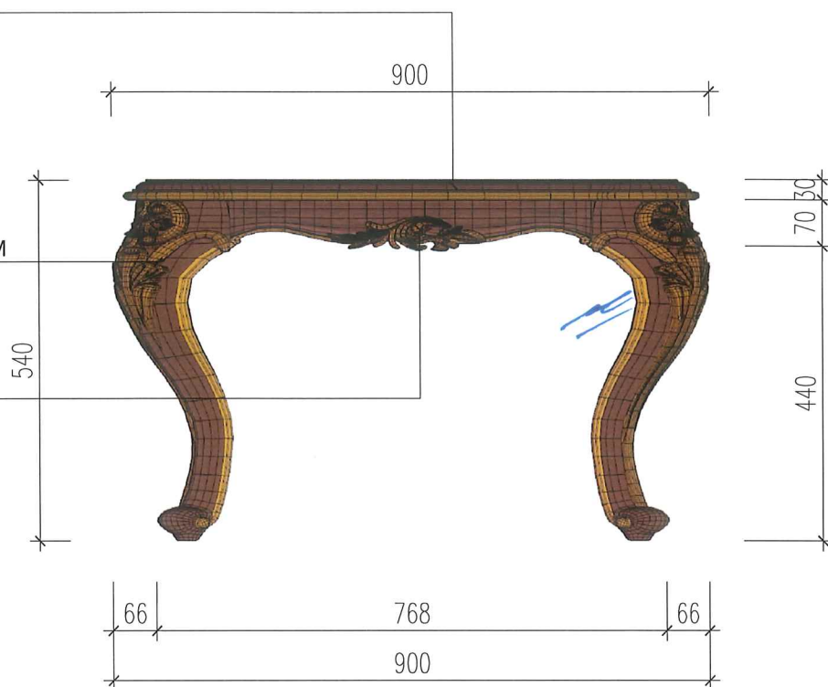
MẶT ĐỨNG
