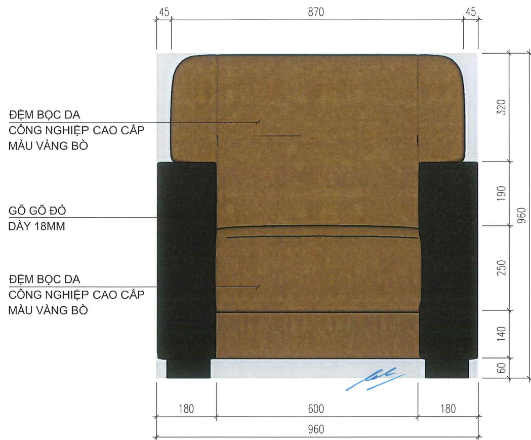
MẶT ĐỨNG
