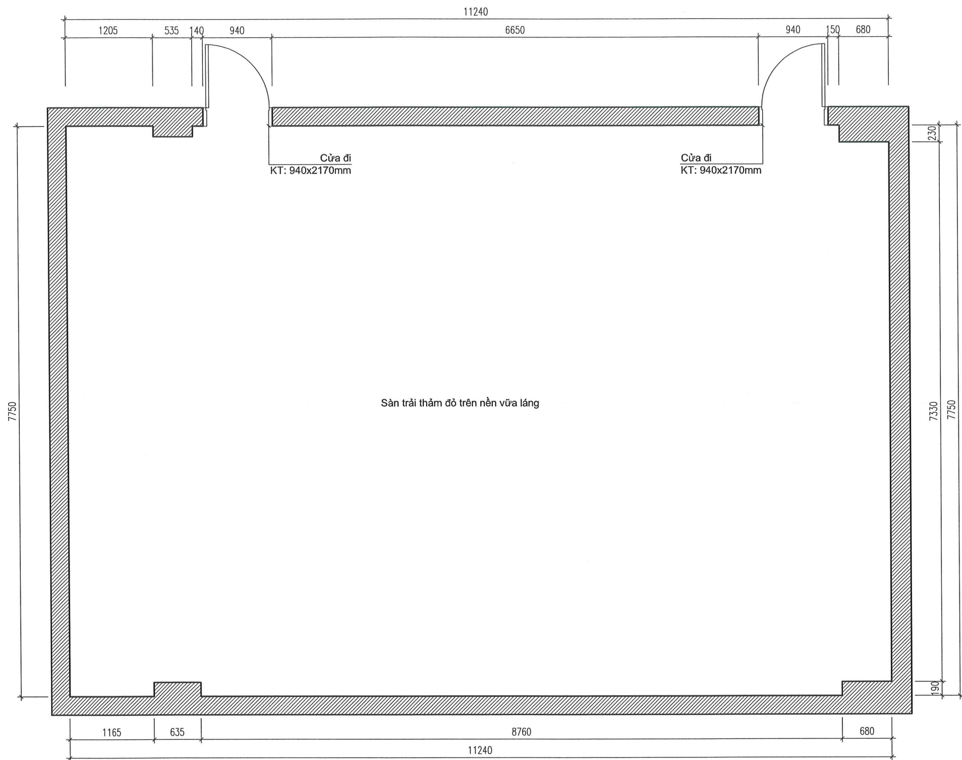
MẶT BẰNG HIỆN TRẠNG
