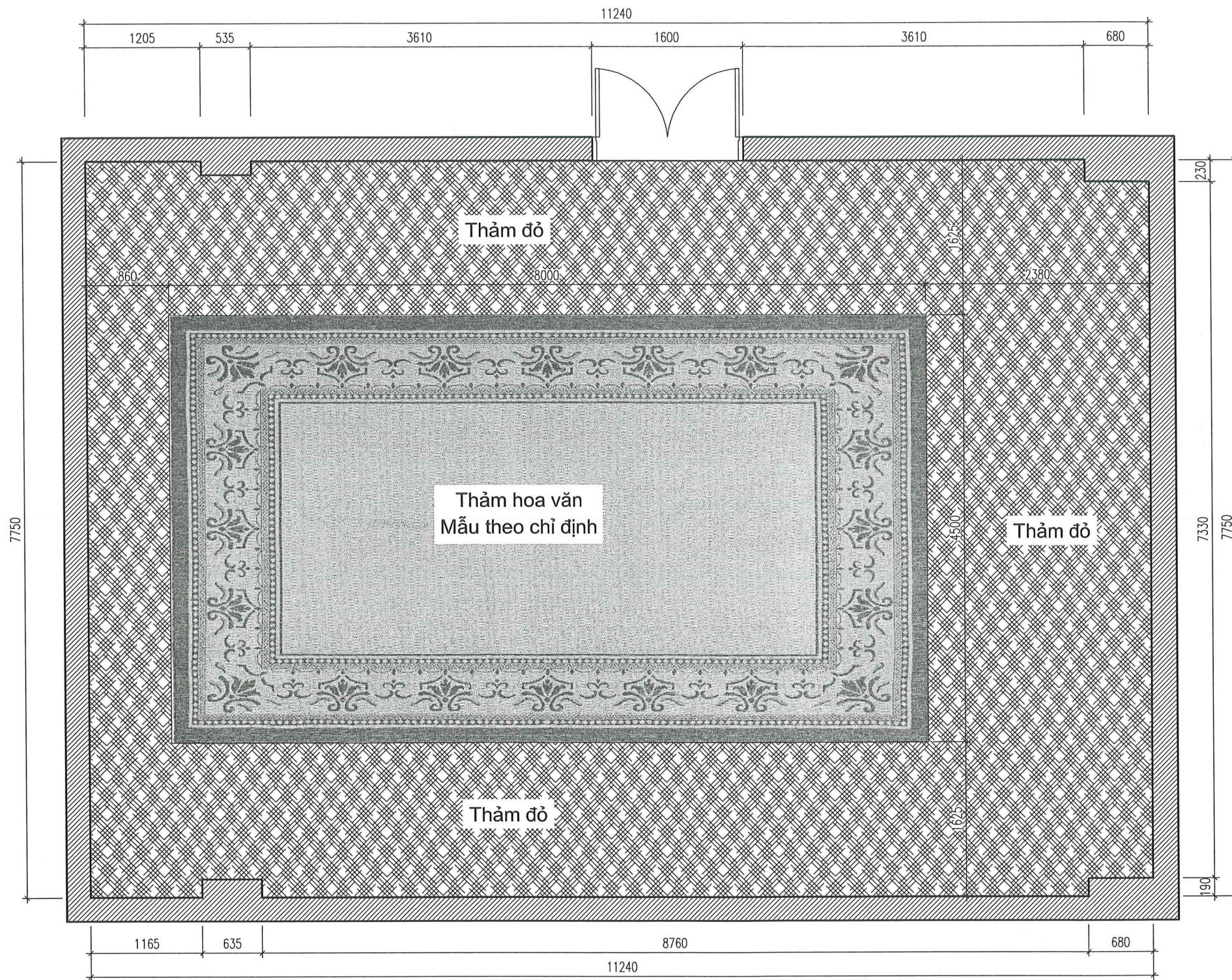
MẶT BẰNG CẢI TẠO SÀN
