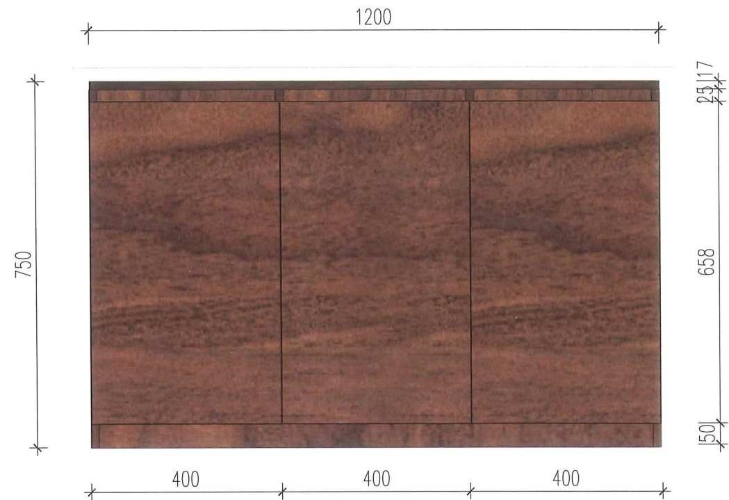
MẶT ĐỨNG
