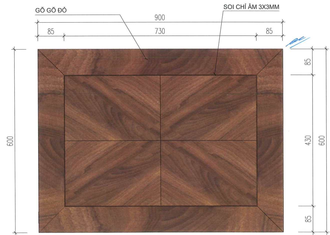
MẶT BẰNG
