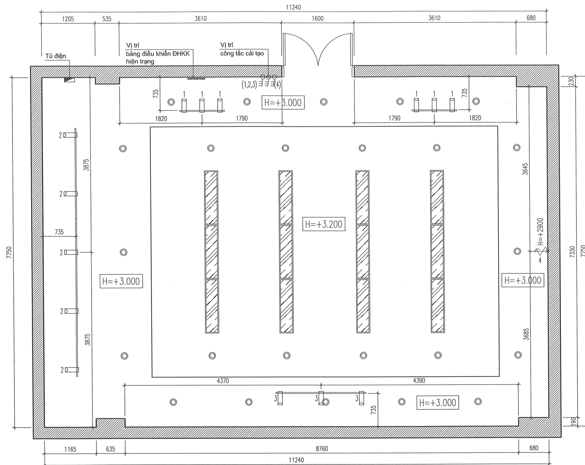
MẶT BẰNG CẤP ĐIỆN CHIẾU SÁNG CẢI TẠO
