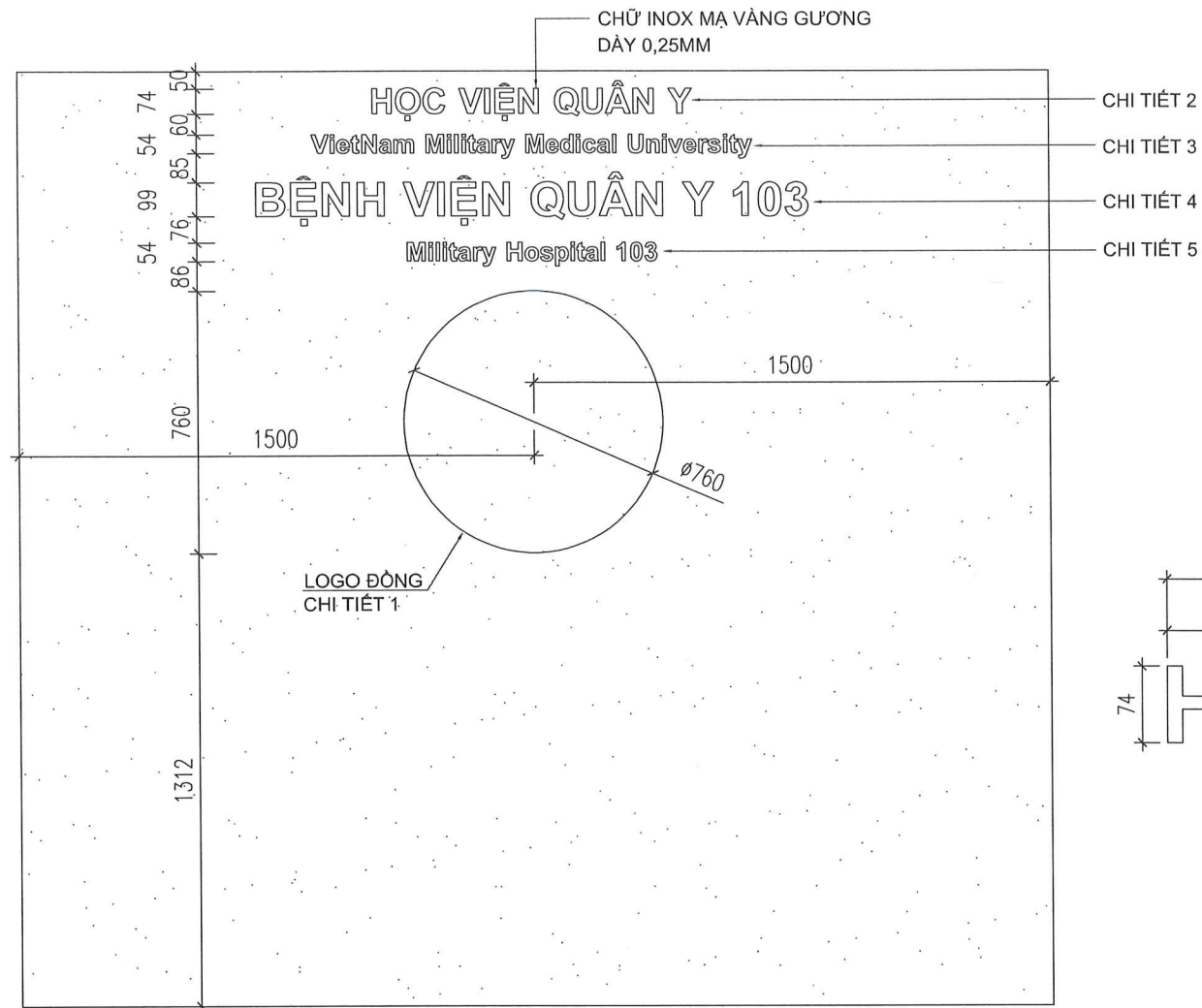
MẶT ĐỨNG ĐỊNH VỊ LOGO
