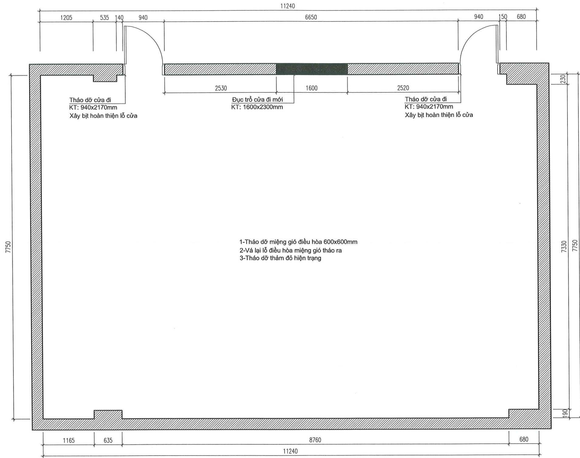
MẶT BẰNG PHÁ DỠ
