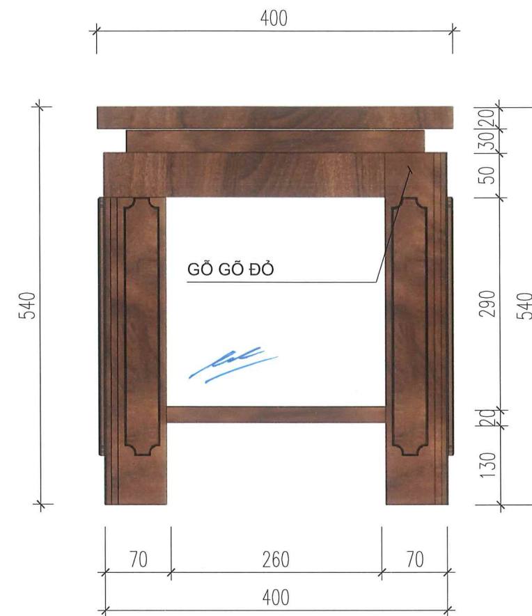
MẶT BÊN
