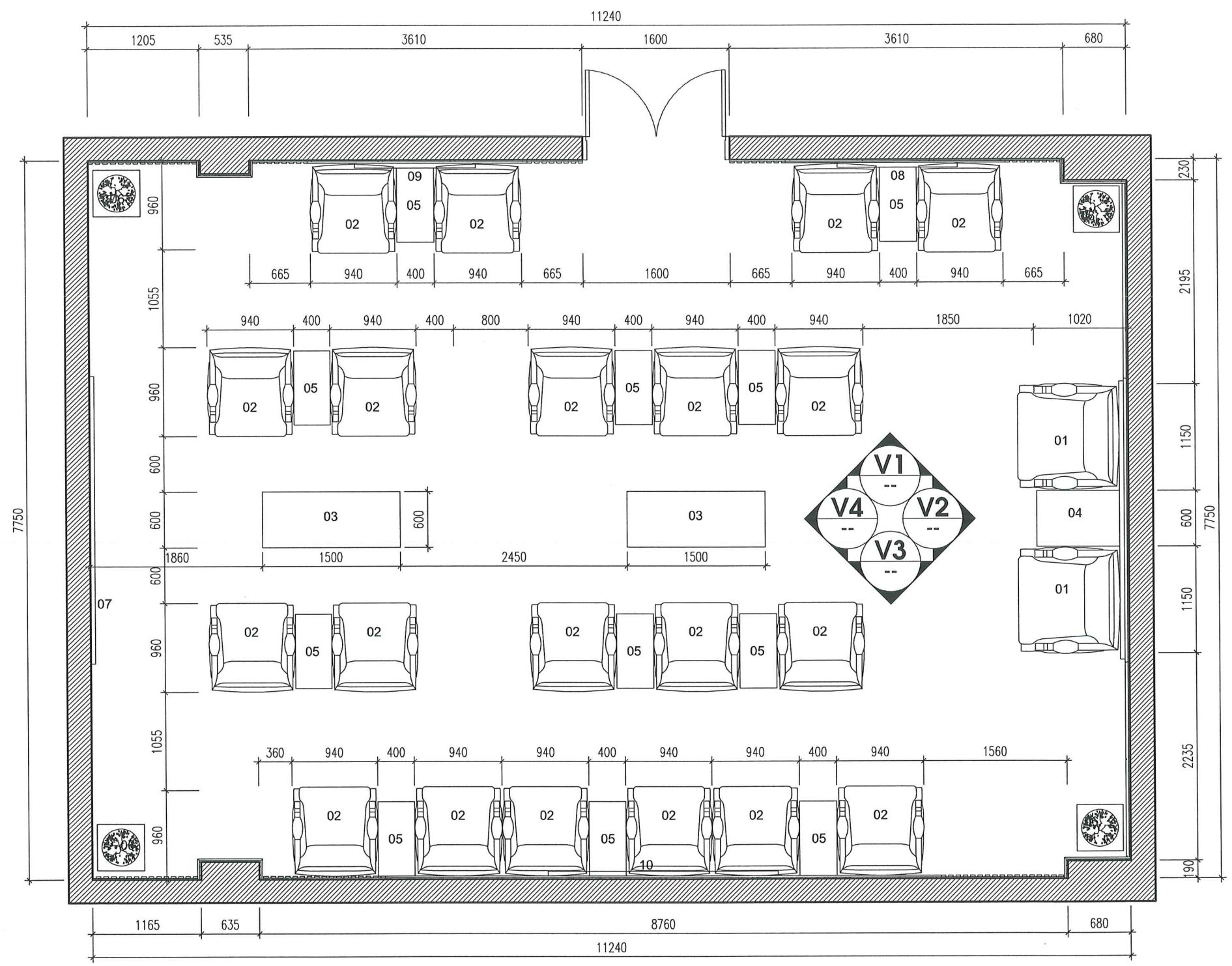
MẶT BẰNG ĐỊNH VỊ NỘI THẤT
