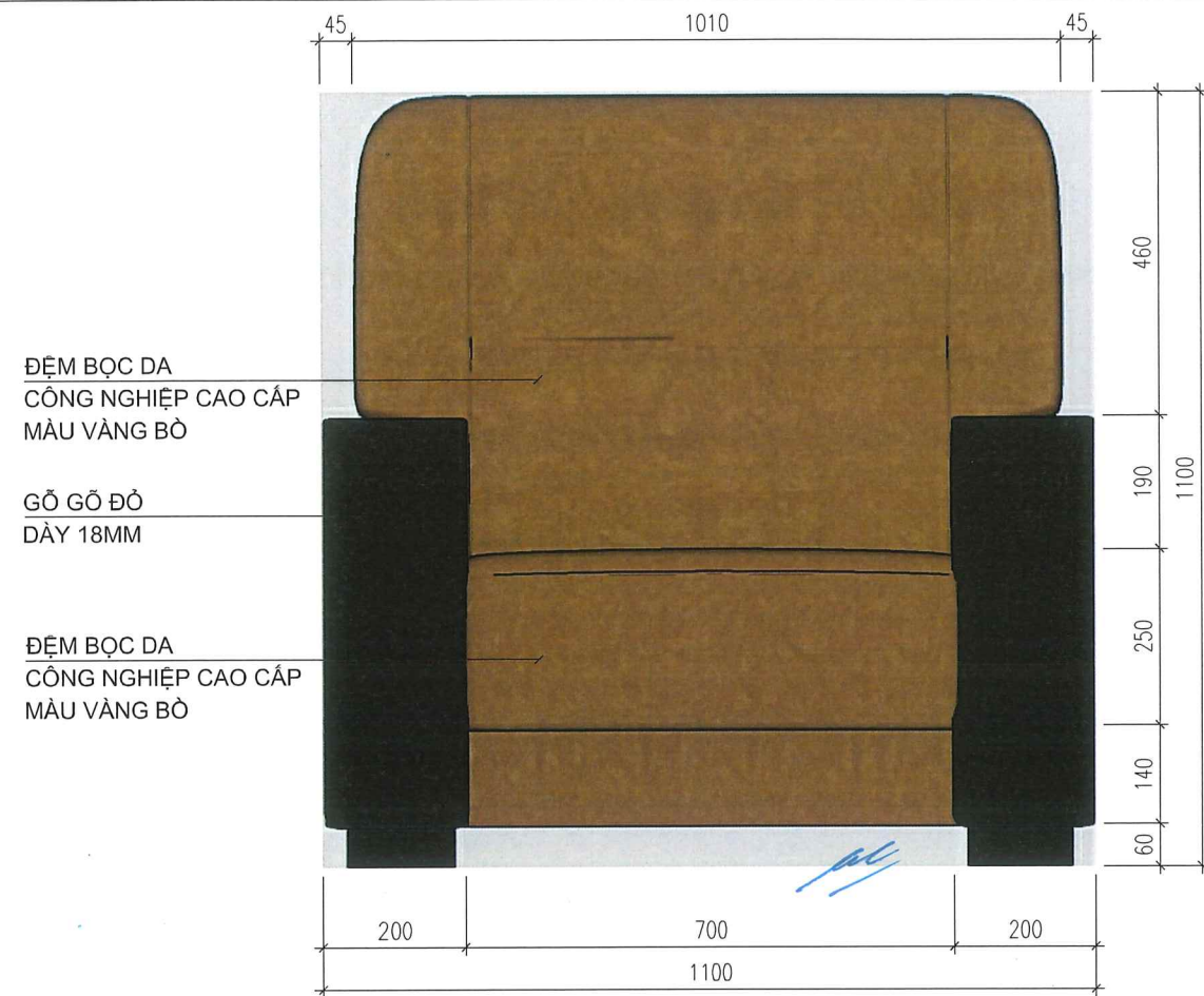
MẶT ĐỨNG
