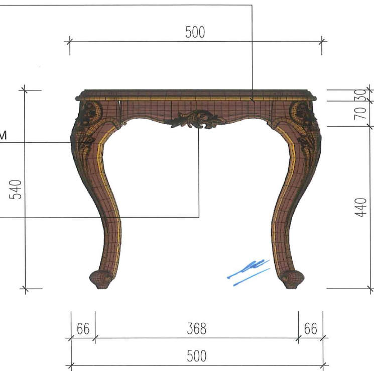
MẶT ĐỨNG
