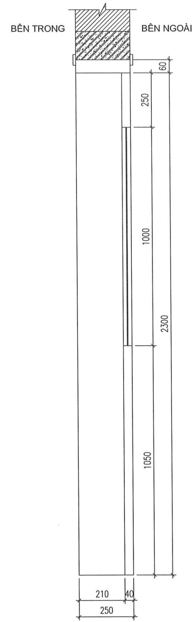
MẶT CẮT DỌC
