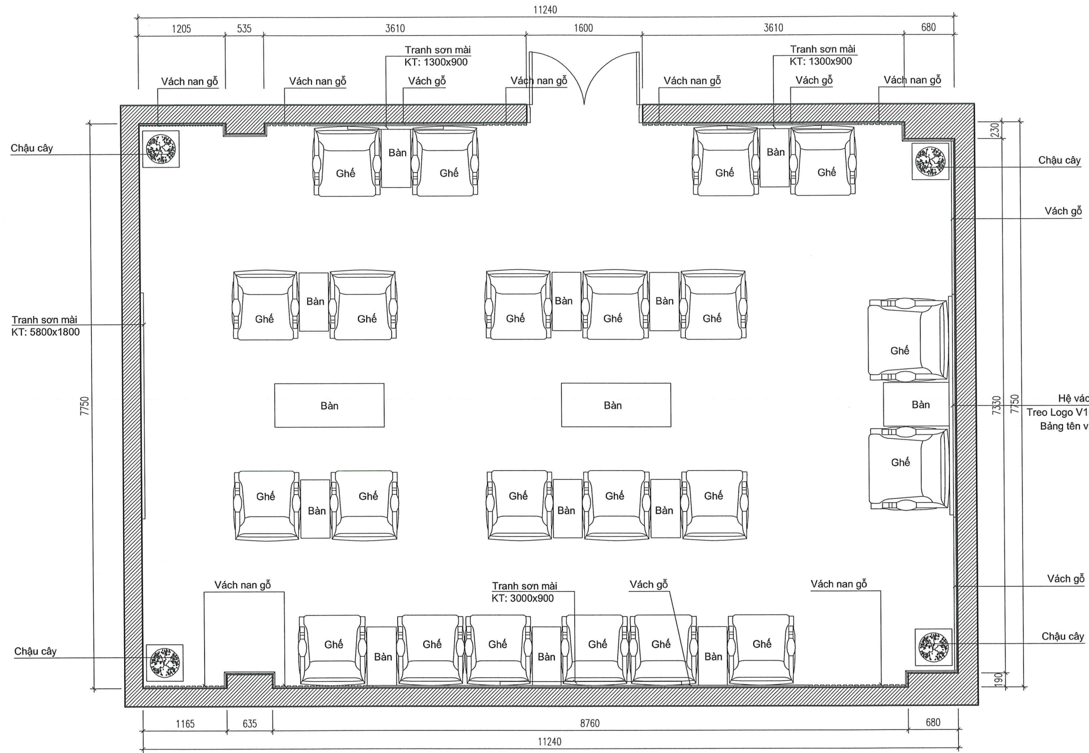
MẶT BẰNG CẢI TẠO NỘI THẤT
