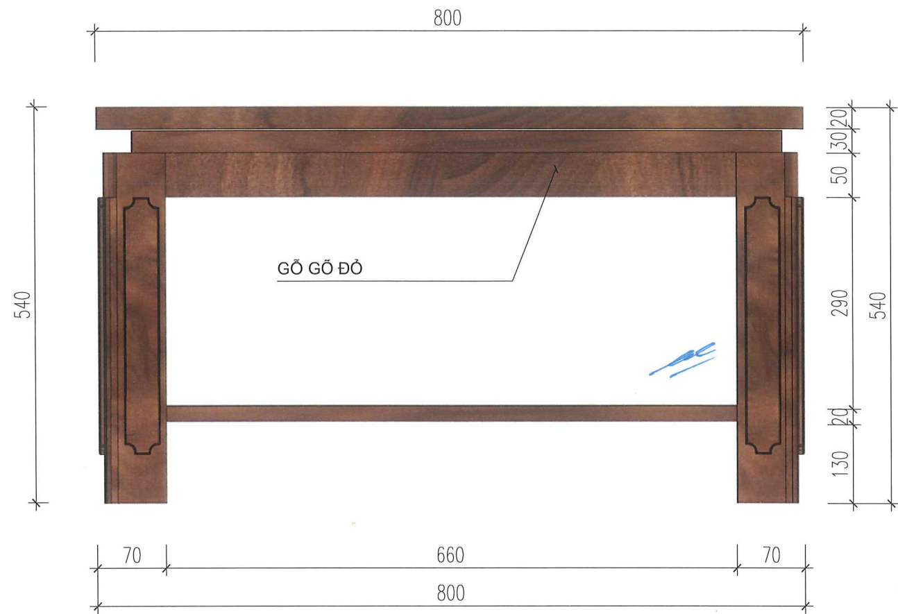
MẶT ĐỨNG
