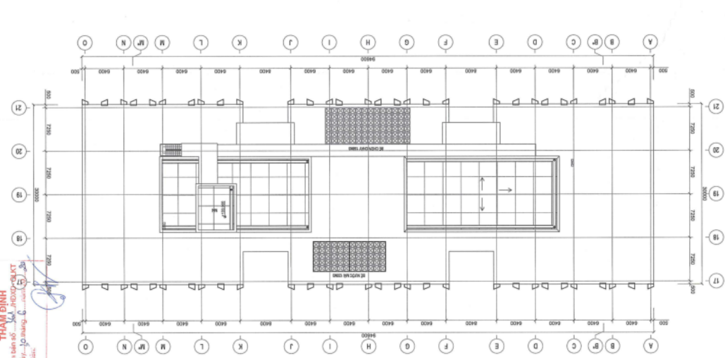
MẶT BẰNG TẦNG 33-M3
