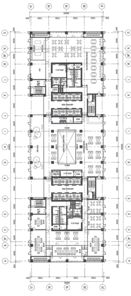
MẶT BẰNG TẦNG 32 TẦNG 32
