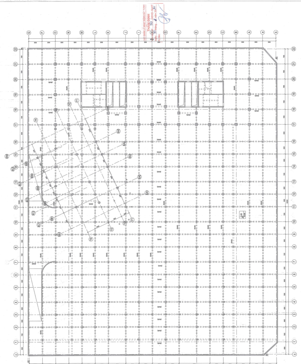
MẶT BẰNG CẦU KIỆN TẦNG B1/F1 B1/F1 FLOOR STRUCTURAL PLAN 1:200
